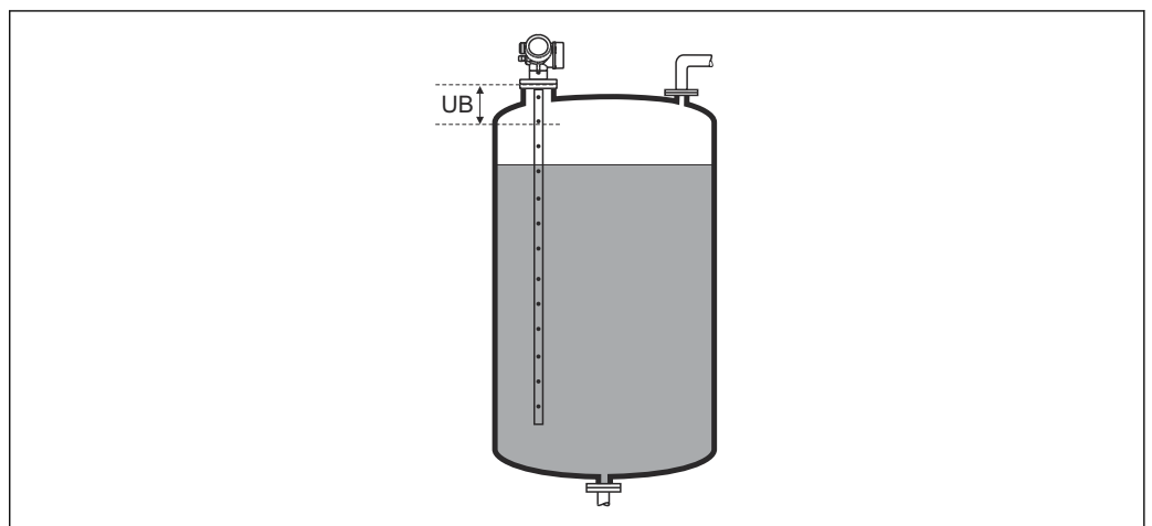
40 液位测量的盲区距离 (UB)
