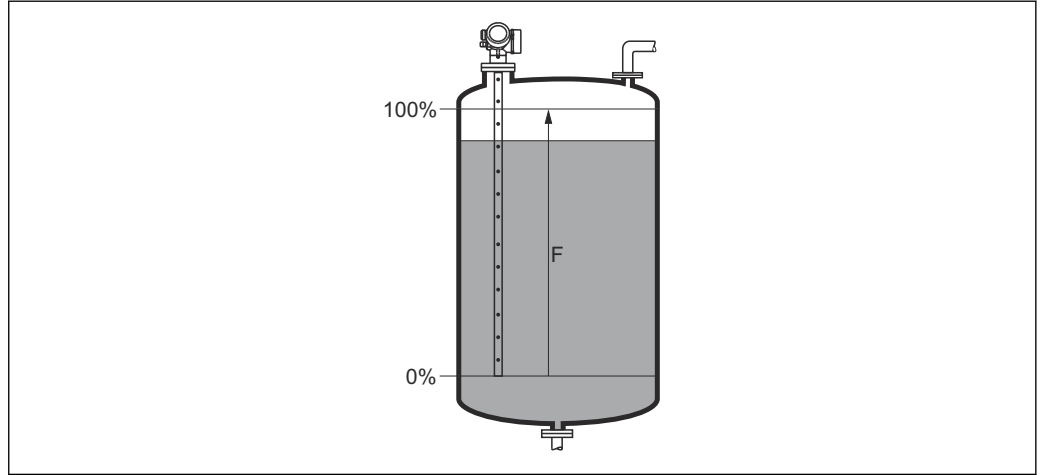
37 液位测量时的满标 (F)
