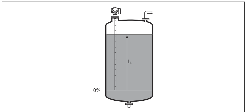
38 液位测量时的液位
