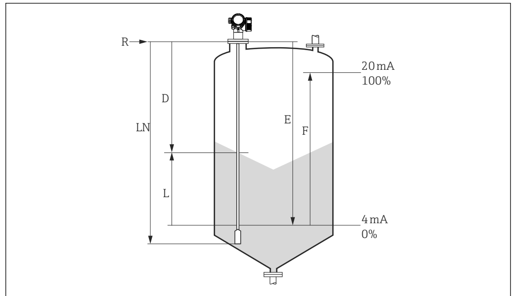
30 Parâmetros de configuração para as medições de nível em sólidos a granel
