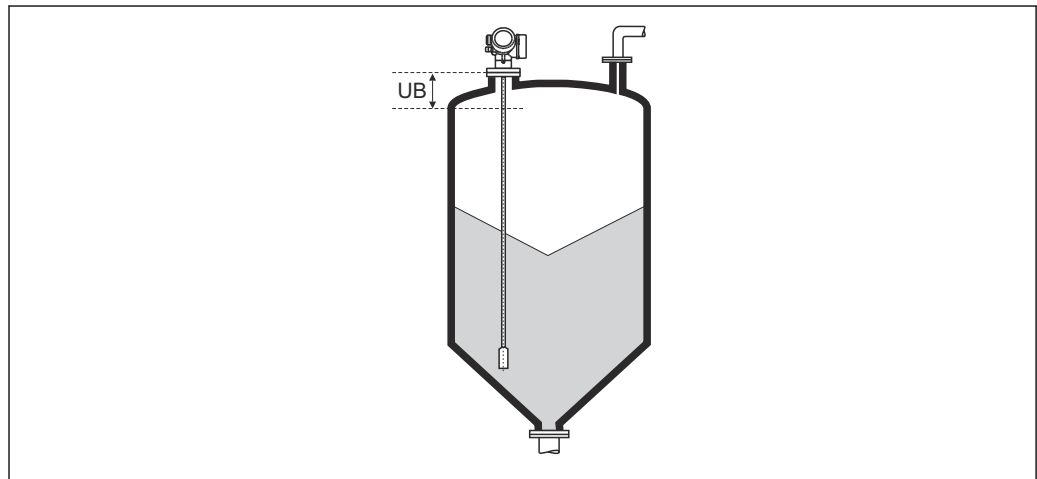
48 Distância de bloqueio (UB) para medições em sólidos
