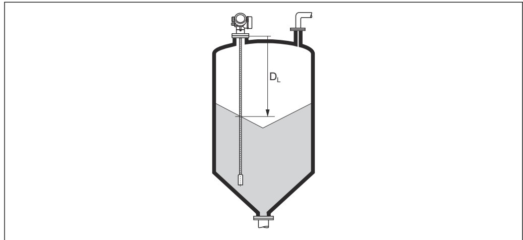
44 Distância para medições de sólidos
