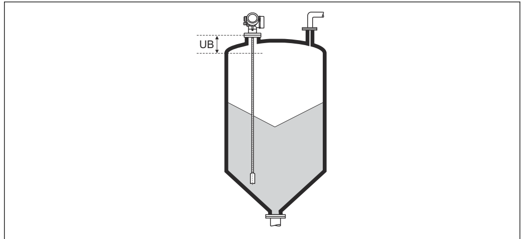
45 Distância de bloqueio (UB) para medições em sólidos
