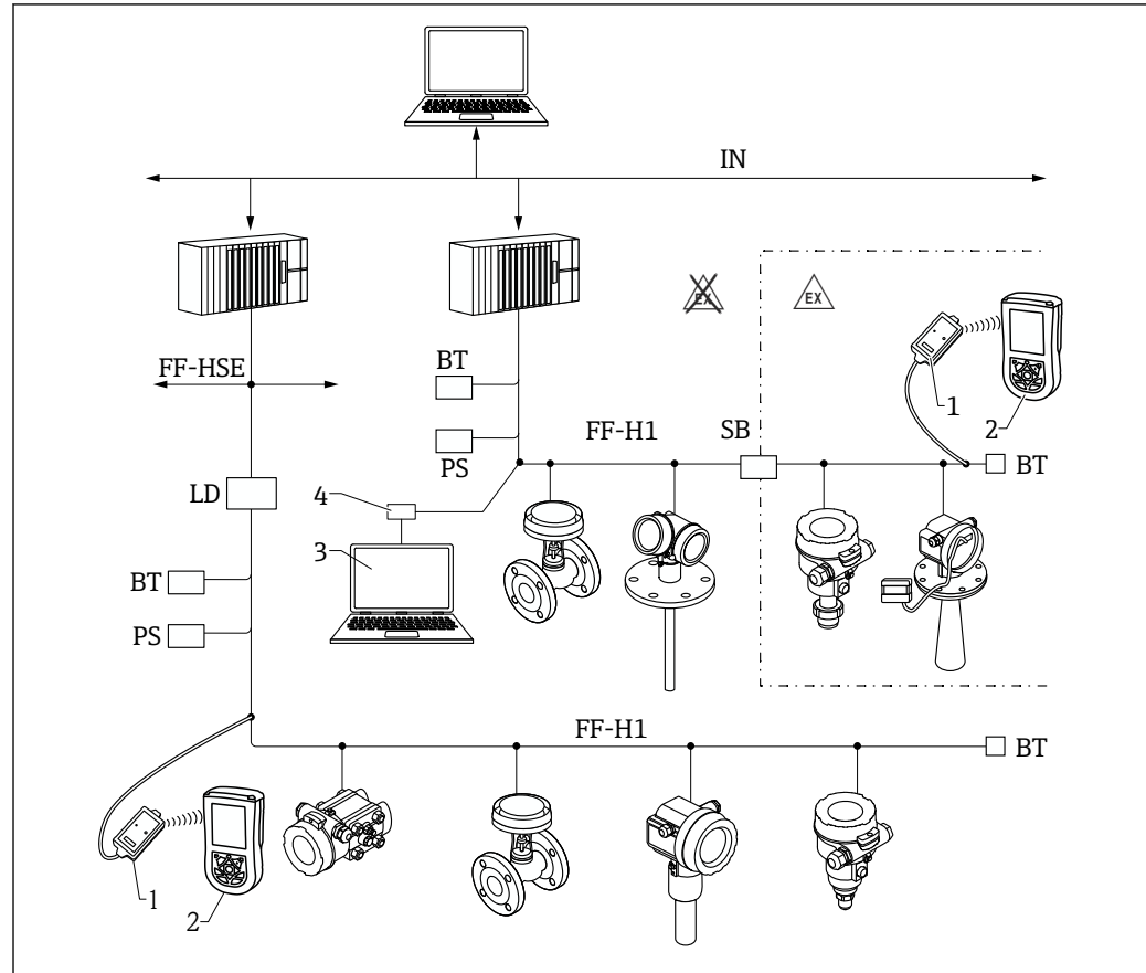
Fig. 20 A arquitetura do sistema da FOUNDATION Fieldbus com componentes associados
