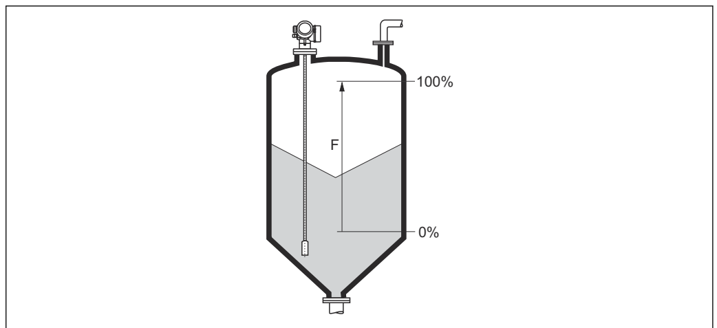
42 Calibração cheia (F) para medições de nível em sólidos
