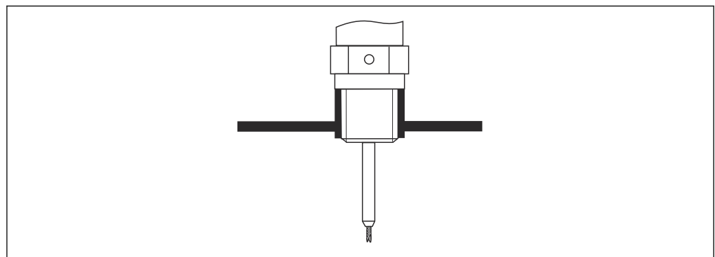
8 安装带螺纹连接的仪表；与罐顶齐平安装
