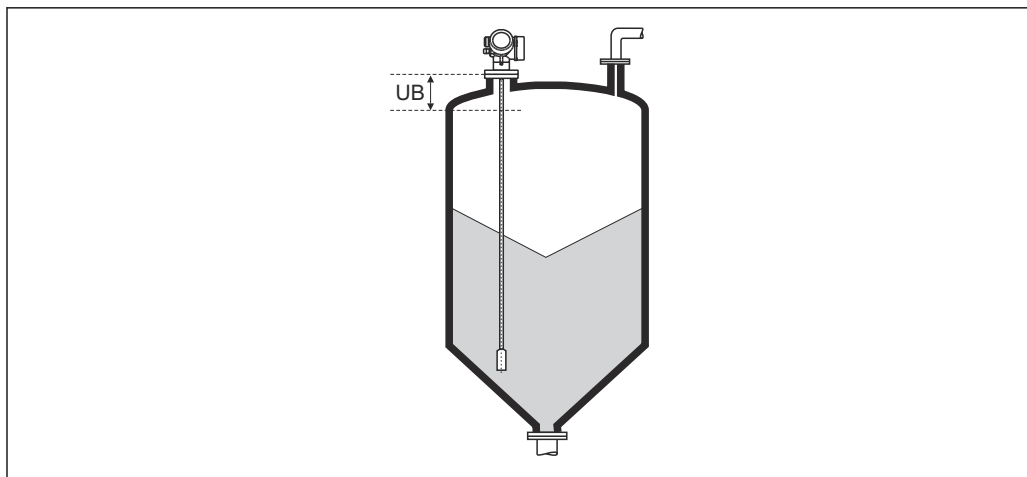
图 48 料位测量的盲区距离 (UB)
