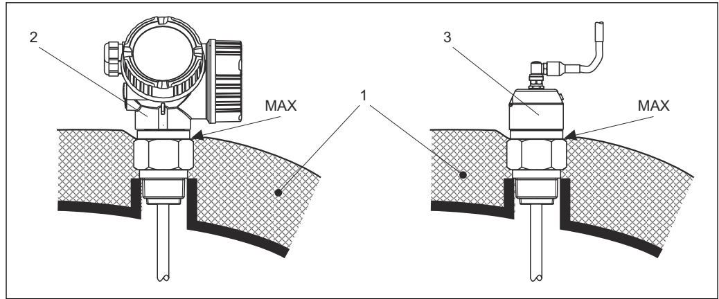
图 9 螺纹过程连接
