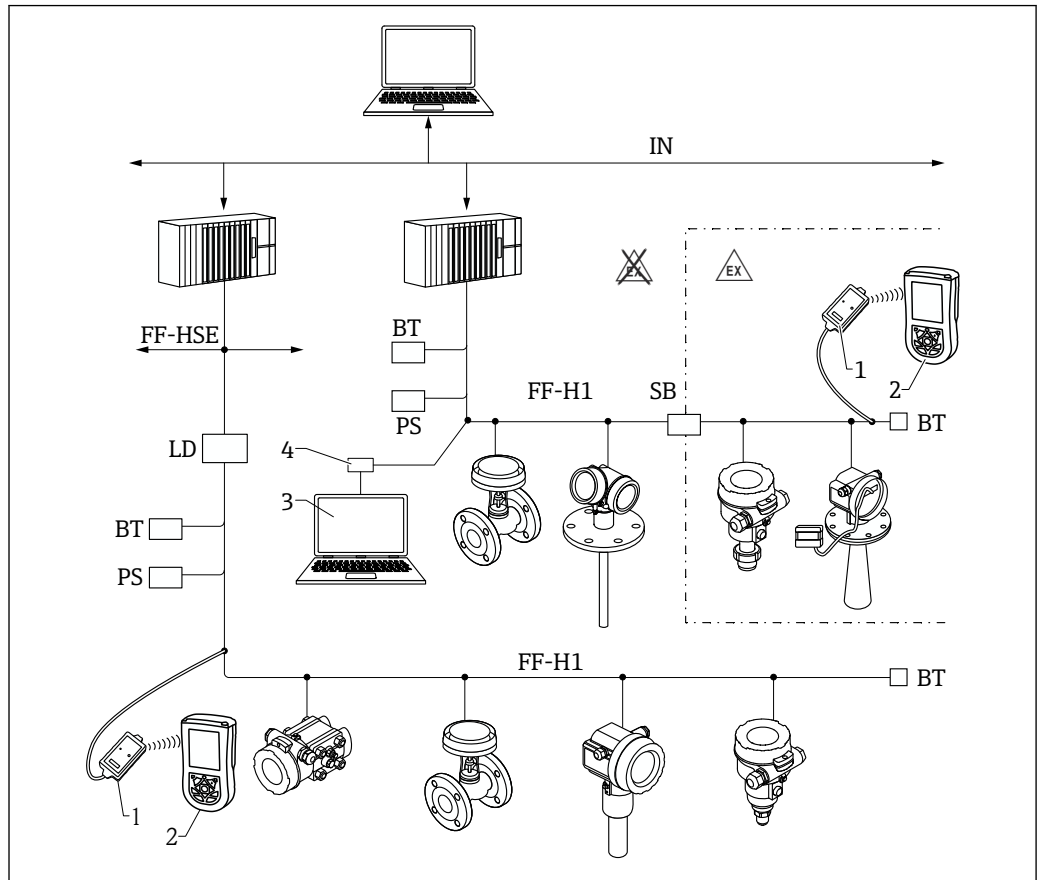
图 20 FOUNDATION Fieldbus 系统架构及组件
