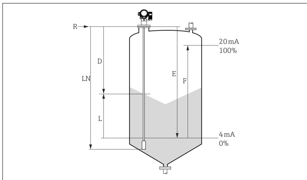
图 27 固体散料料位测量的设置参数
