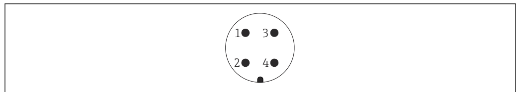
图 16 7/8"插头的针脚分配
