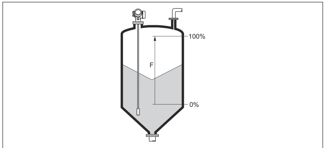
42 料位测量时的满标 (F)
