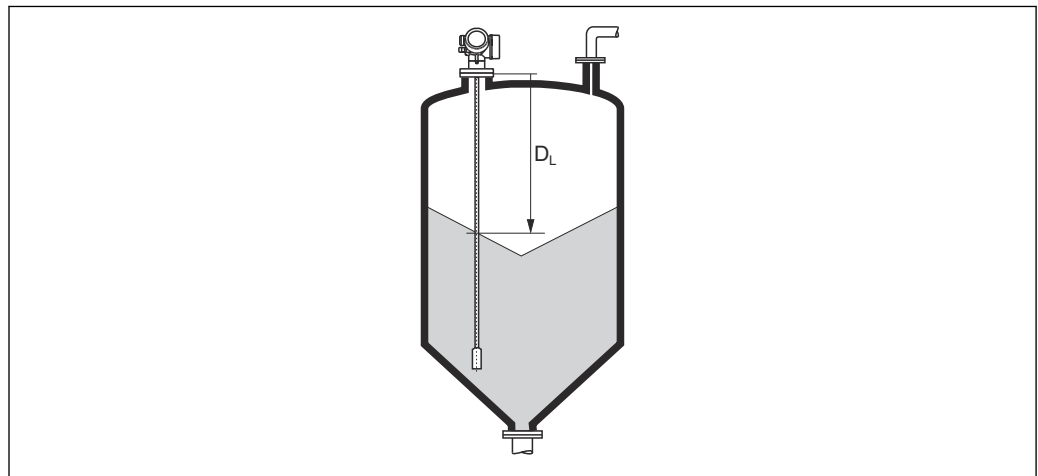
图 44 料位测量时的距离
