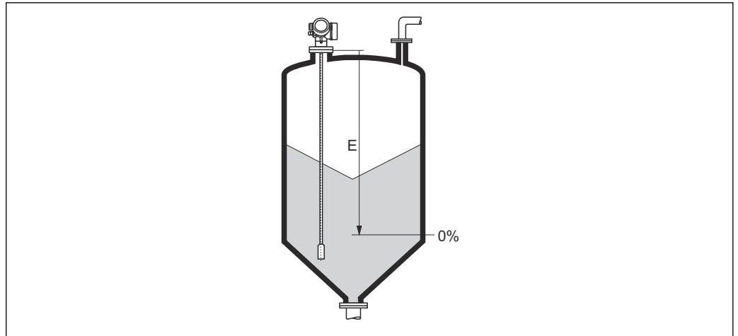
41 料位测量时的空标 (E)
