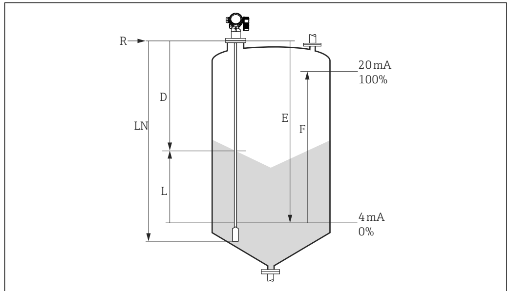
图 30 固体散料料位测量的设置参数
