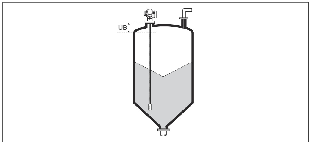
图 45 料位测量的盲区距离 (UB)
