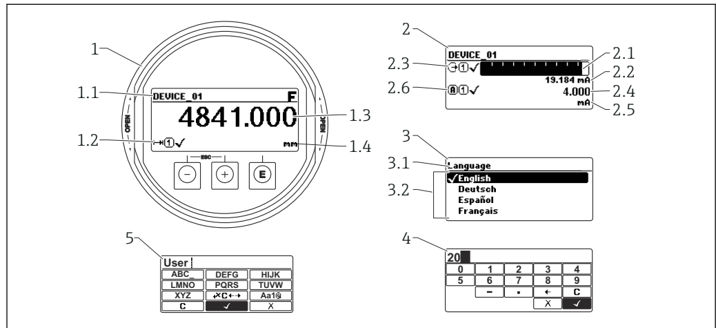
图 23 显示与操作单元的显示格式
