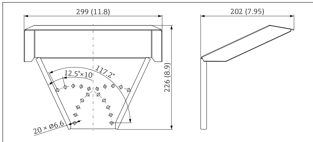
25 Размеры. Единица измерения мм (дюйм)
