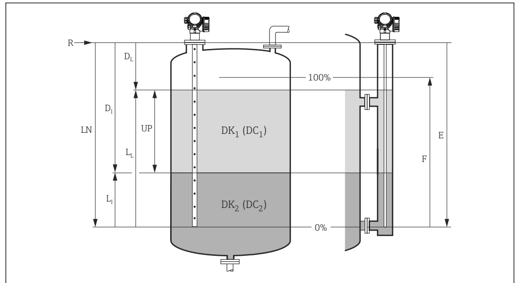
19 Параметры конфигурации измерения границы раздела фаз
