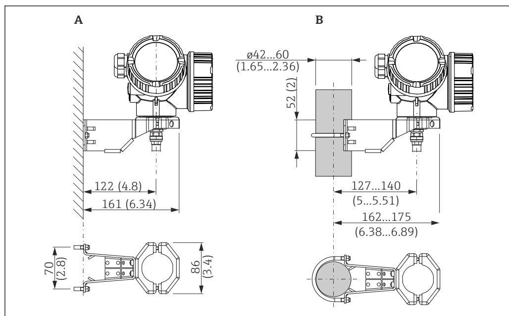
8 Монтаж корпуса блока электроники на монтажном кронштейне. Единица измерения мм (дюйм)
