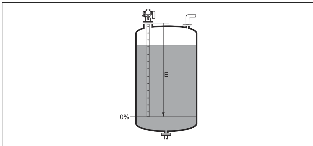
30 Калибровка пустой емкости (E) для измерения уровня жидких сред
