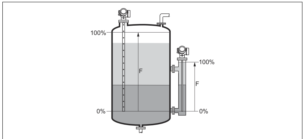
33 Калибровка полной емкости (F) для измерения уровня границы раздела фаз
