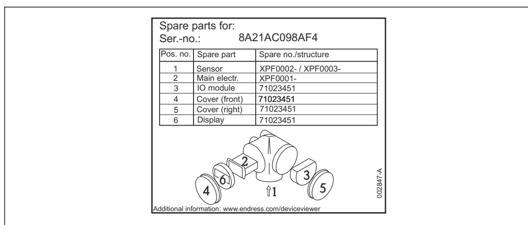
▣ 22 Пример заводской таблички с перечнем запасных частей, размещаемой на крышке присоединительного отсека
