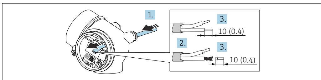
11 Единица измерения: мм (дюймы)
