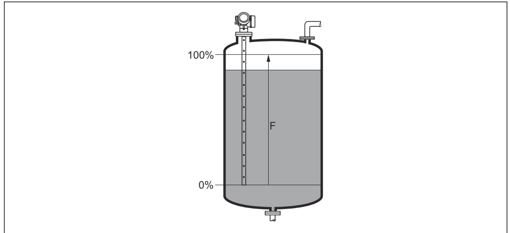
32 Калибровка полной емкости (F) для измерения уровня жидких сред
