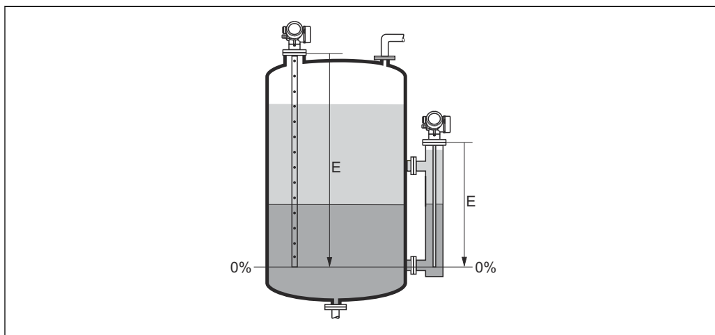
31 Калибровка пустой емкости (E) для измерения уровня границы раздела фаз
