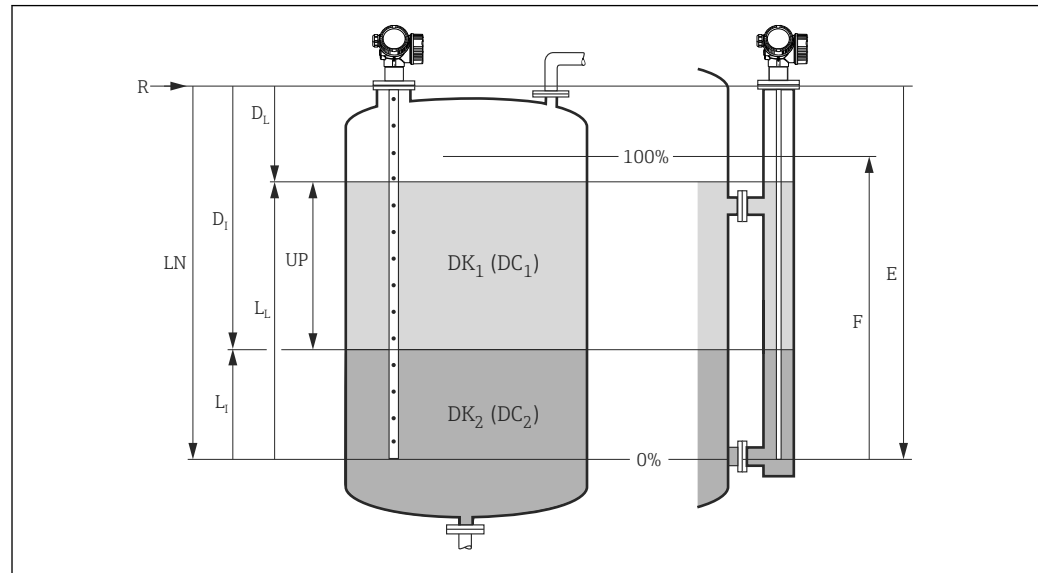
19 Parámetros de configuración para la medición de la interfase
