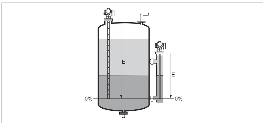
31 Calibración vacío (E) para mediciones de la interfase
