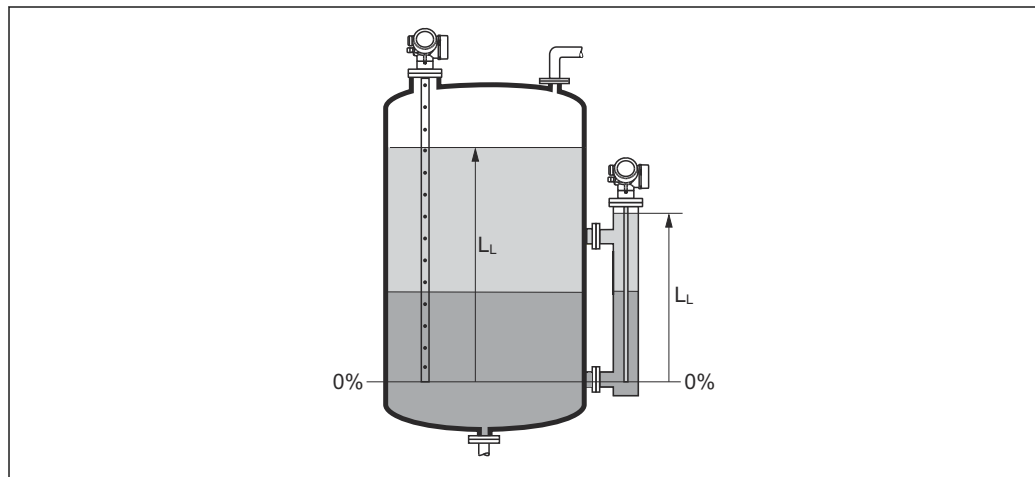
35 Nivel en caso de mediciones de la interfase
