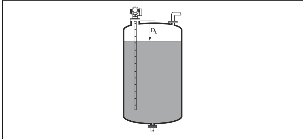
36 Distancia para mediciones de líquidos
