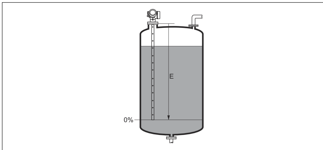
30 Calibración vacío (E) para mediciones de nivel en líquidos
