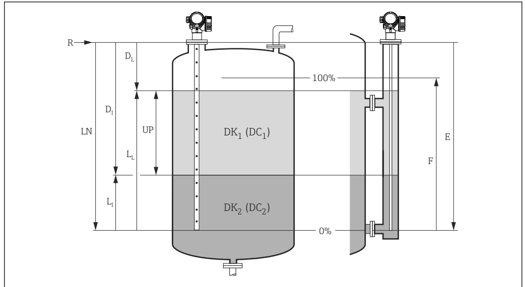
図 24 界面測定用パラメータの設定
