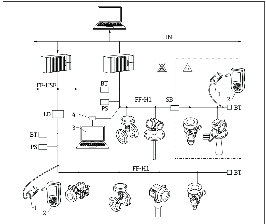
図 14 FOUNDATION フィールドバスシステム構成および関連するコンポーネント
