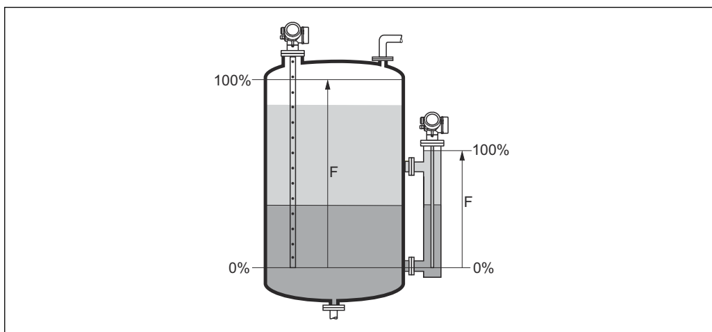
図 35 界面測定用の満量校正 (F)
