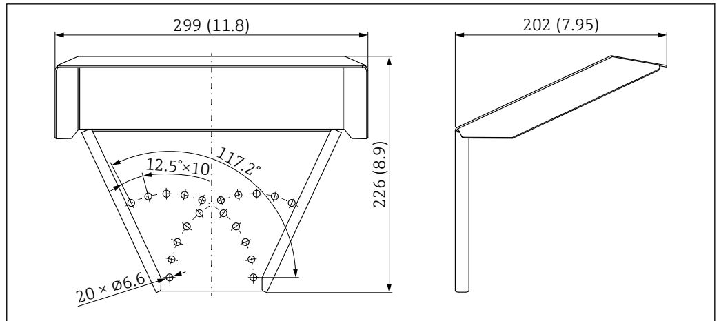
図 31 寸法。測定単位 mm (in)
