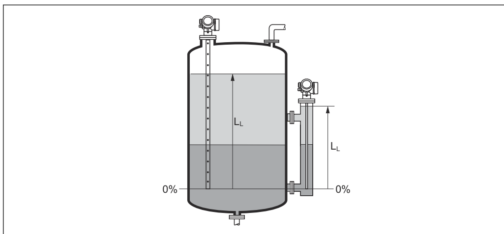
図 36 界面測定時のレベル
