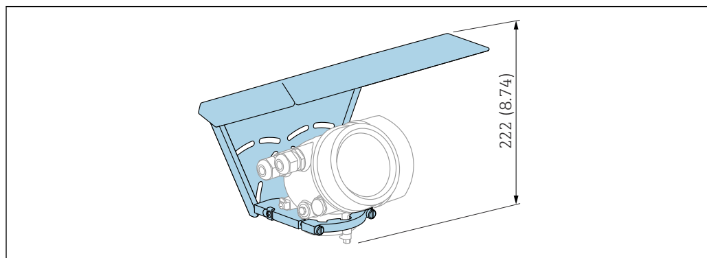
図 30 高さ。測定単位 mm (in)
