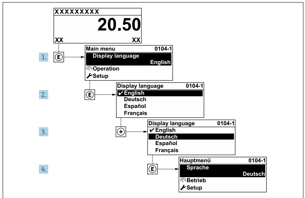
📖 20 現場表示器の使用例
