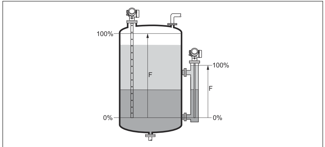
35 界面测量时的满标 (F)
