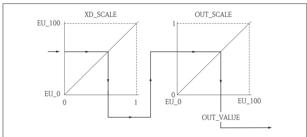
图 23 按比例转换 AI 块中的测量值
