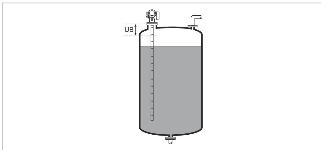
40 Блокирующая дистанция (UB) для измерения в жидких средах
