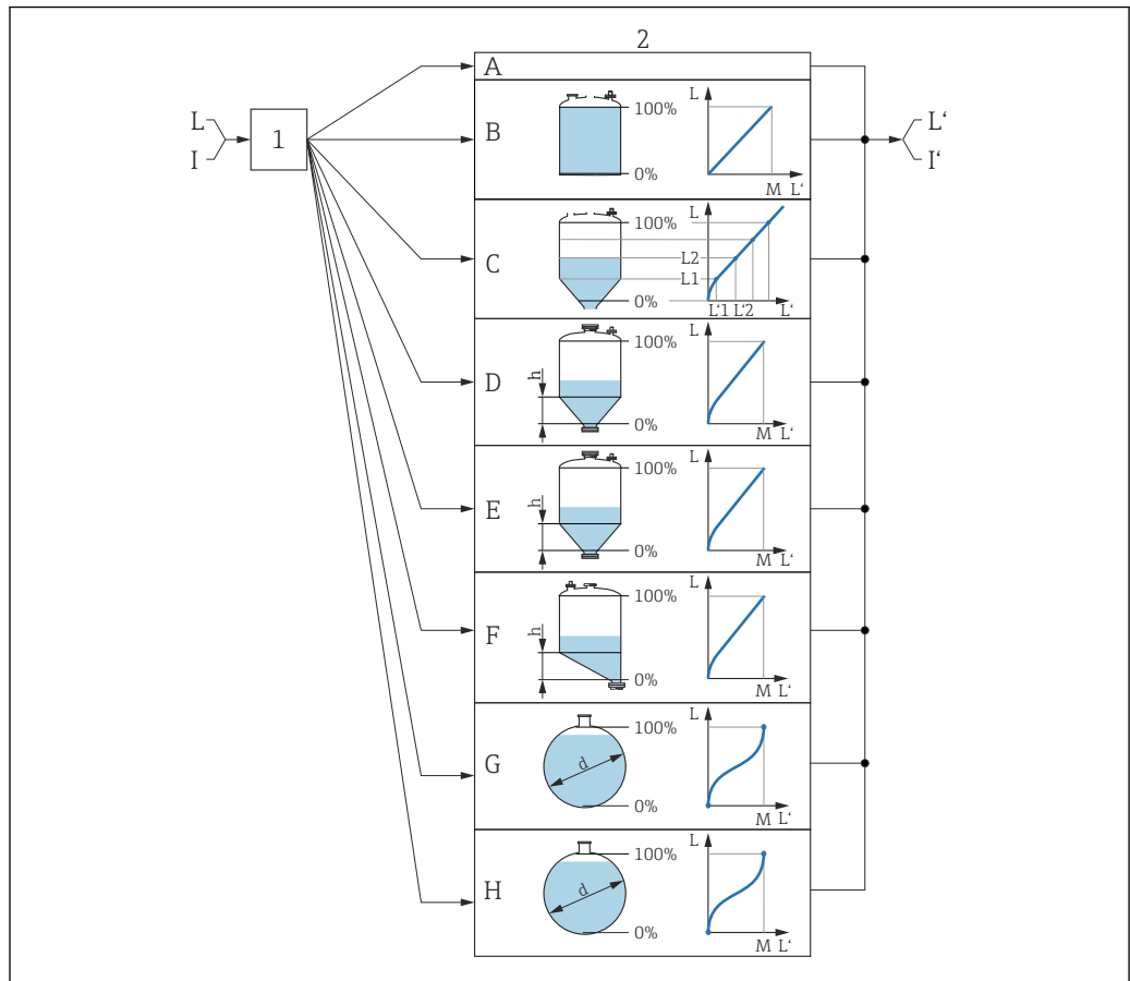
38 Линеаризация: преобразование уровня и, если применимо, границы раздела фаз в объем или массу; преобразование зависит от формы резервуара
