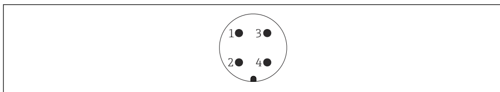
10 Назначение контактов разъема 7/8
