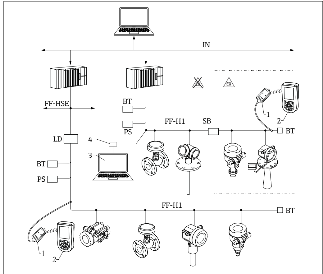
14 Системная архитектура FOUNDATION Fieldbus и сопутствующие компоненты
