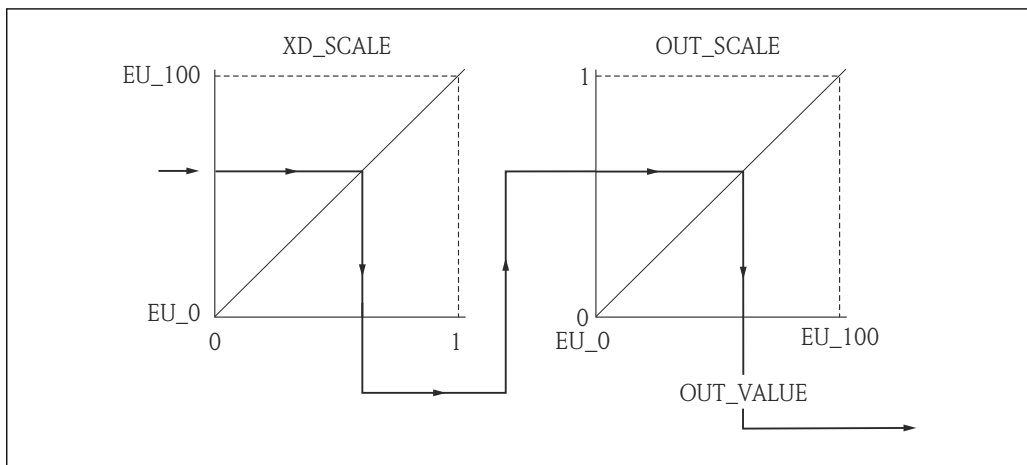
23 Масштабирование измеренного значение в блоке аналоговых входов
