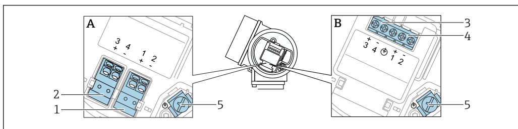
8 Назначение клемм; PROFIBUS PA/FOUNDATION Fieldbus
