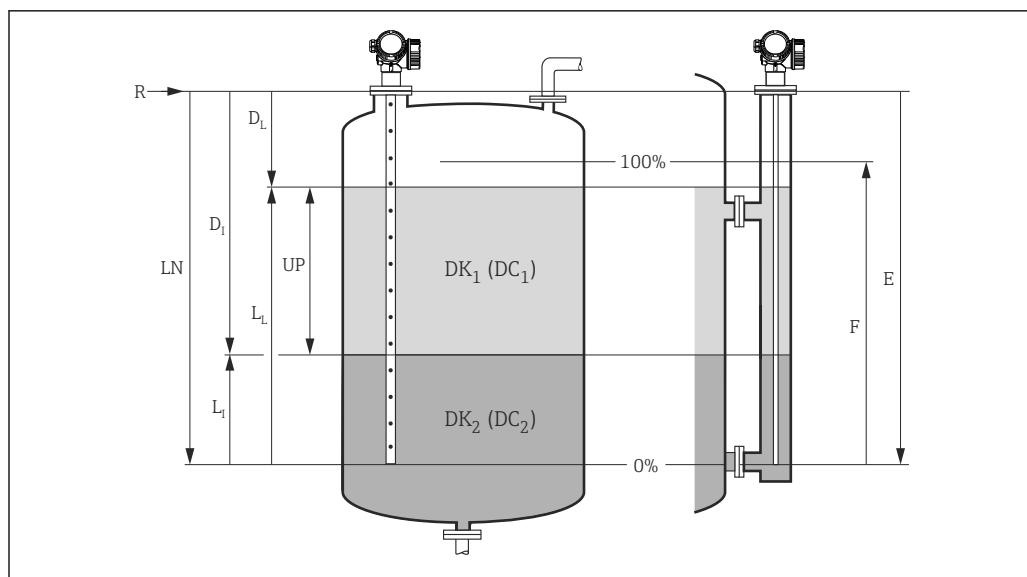
24 Параметры конфигурации измерения границы раздела фаз
