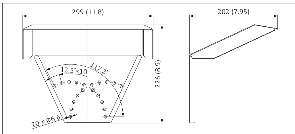
31 Размеры. Единица измерения мм (дюйм)
