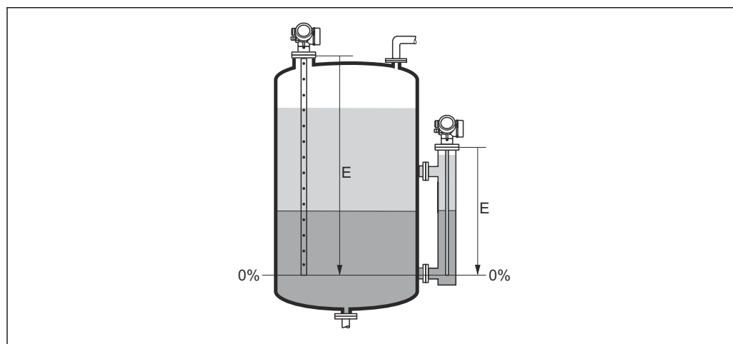
🔍 34 Калибровка пустой емкости (E) для измерения уровня границы раздела фаз
