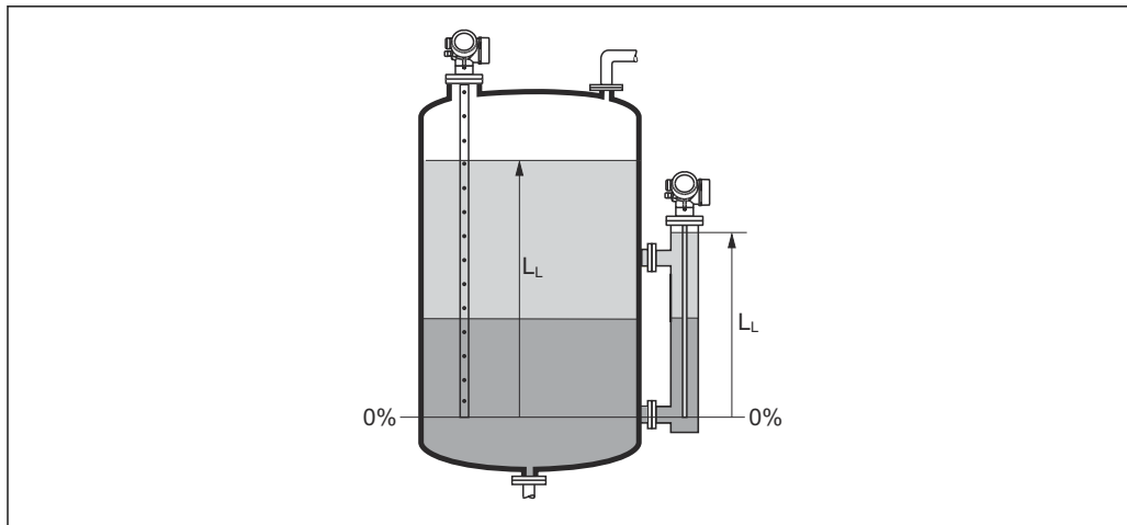
36 Уровень при измерении уровня границы раздела фаз
