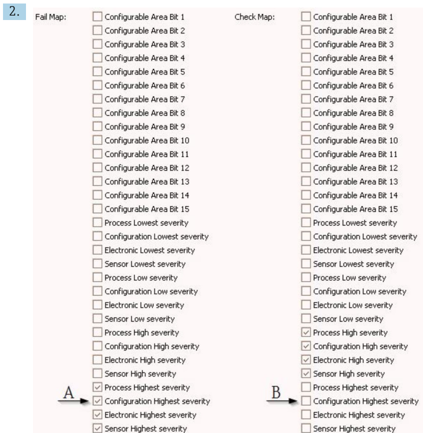
25 Стандартное состояние столбцов "Карта неисправностей" и "Карта проверок"
