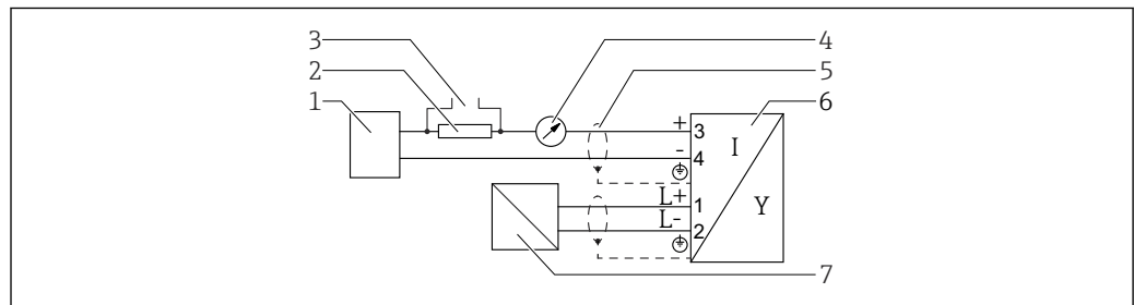
图 14 功能框图，四线制：4 ... 20 mA HART (10.4 ... 48 V DC )
