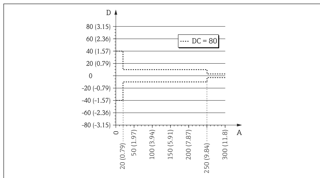
图 22 缆式探头底部附近的测量误差
