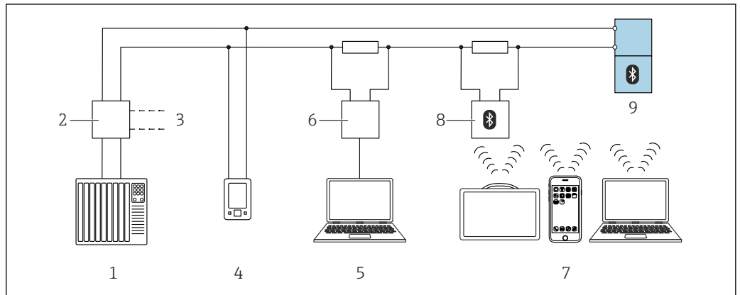
图 36 通过 HART 通信实现远程操作
