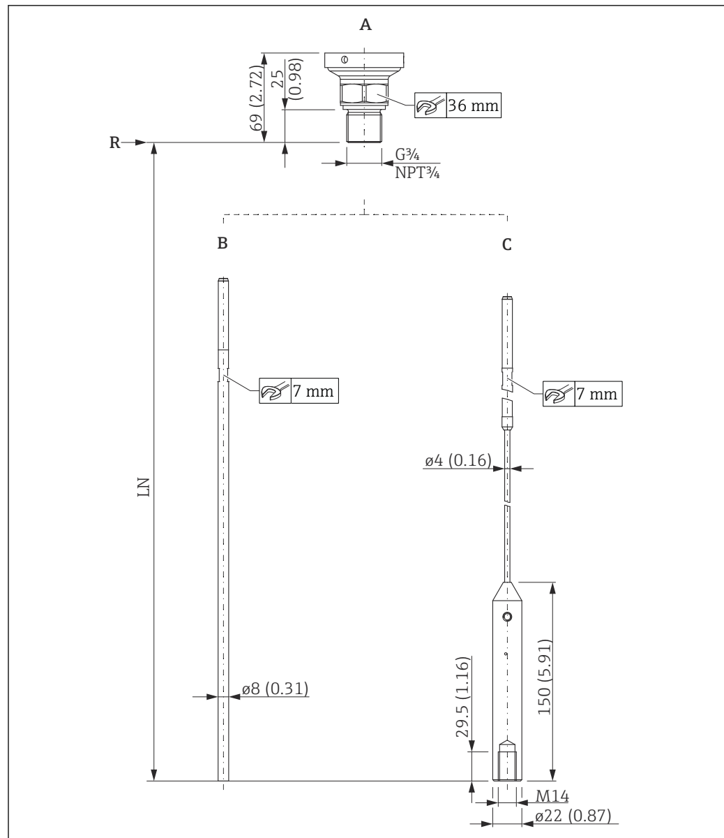
图 31 FMP50: 过程连接和探头。测量单位 mm (in)
