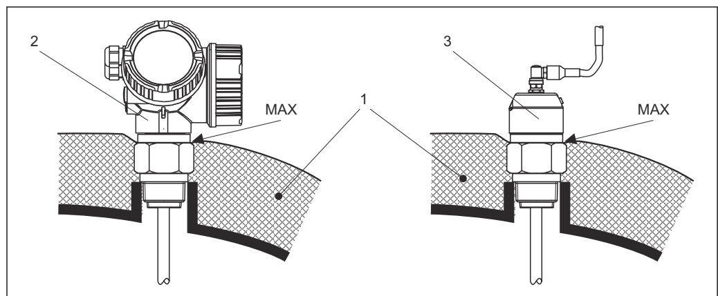
图 26 螺纹过程连接
