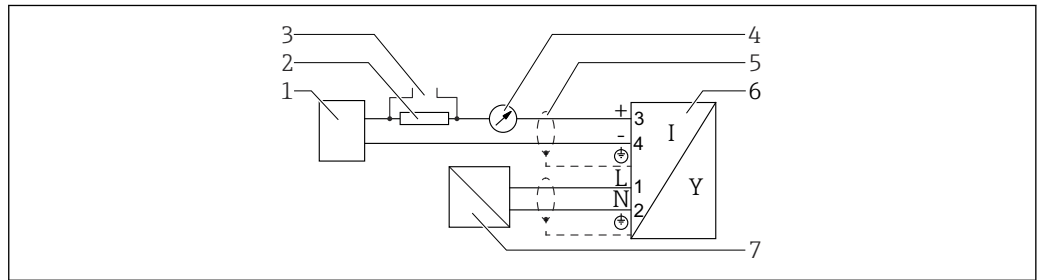
图 16 功能框图，四线制：4 ... 20 mA HART (90 ... 253 V AC )
