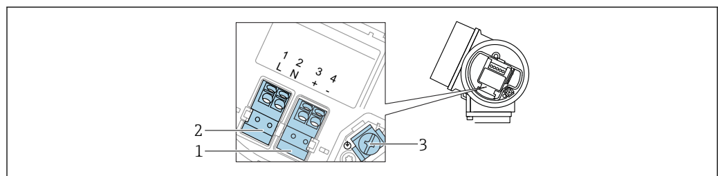
图 15 接线端子分配，四线制：4 ... 20 mA HART (90 ... 253 V AC )
