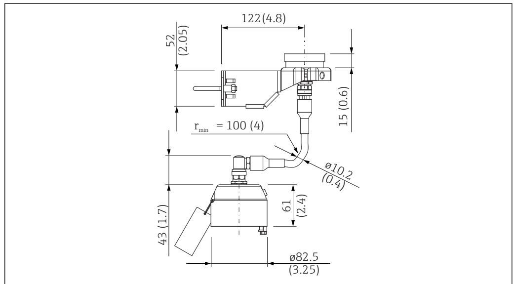
图 30 分体式探头连接件；连接电缆长度为订购长度。测量单位 mm (in)
