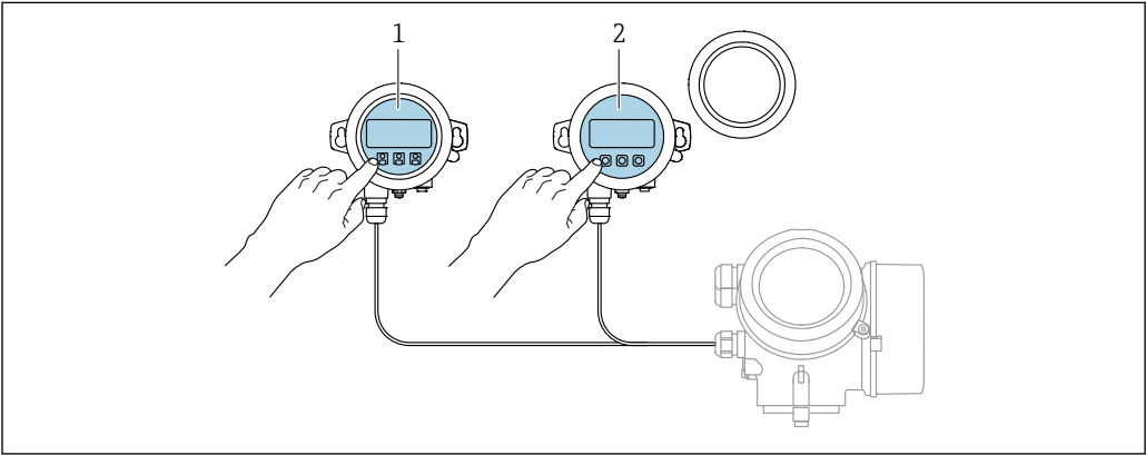
44 FHX50 的操作选项 1 显示与操作单元 SD03，光敏键操作，可以在玻璃盖板外部操作 2 显示与操作单元 SD02，按键操作；必须打开盖板
