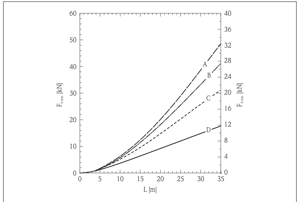
图 26 张力负载与物位 (L) 关系曲线图; 6 mm (0.24 in) 和 4 mm (0.16 in) 缆式探头, 石英砂料仓; 光滑金属仓壁
