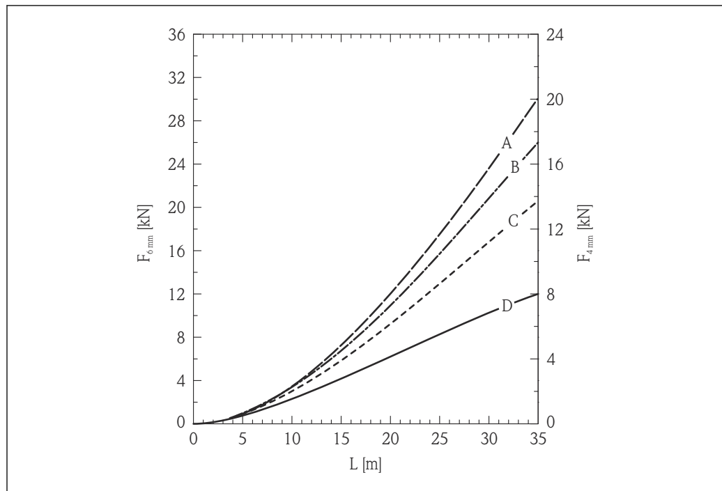
图 28 张力负载与物位 (L) 关系曲线图; 6 mm (0.24 in) 和 4 mm (0.16 in) 缆式探头, 小麦料仓; 光滑金属仓壁
