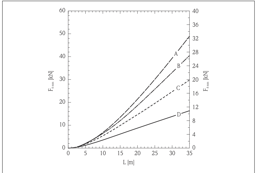
图 29 张力负载与物位 (L) 关系曲线图; 6 mm (0.24 in) 和 4 mm (0.16 in) 缆式探头, 水泥料仓; 光滑金属仓壁
