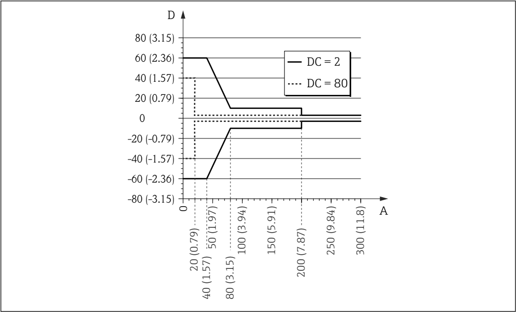
22 杆式探头和同轴探头底部附近的测量误差
