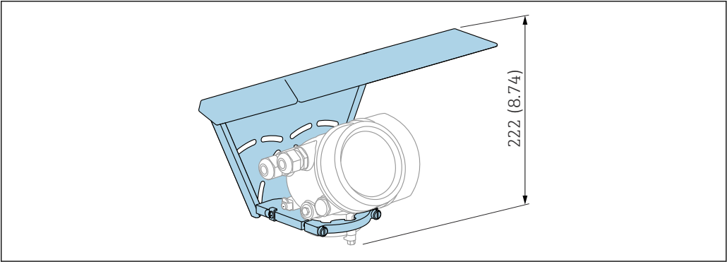
52 高度。测量单位 mm (in)
