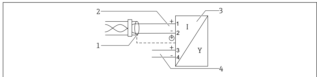
图 19 功能框图：PROFIBUS PA / FOUNDATION Fieldbus
