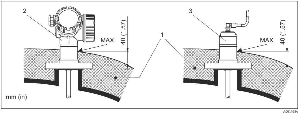
图 32 带法兰过程连接的 FMP57
