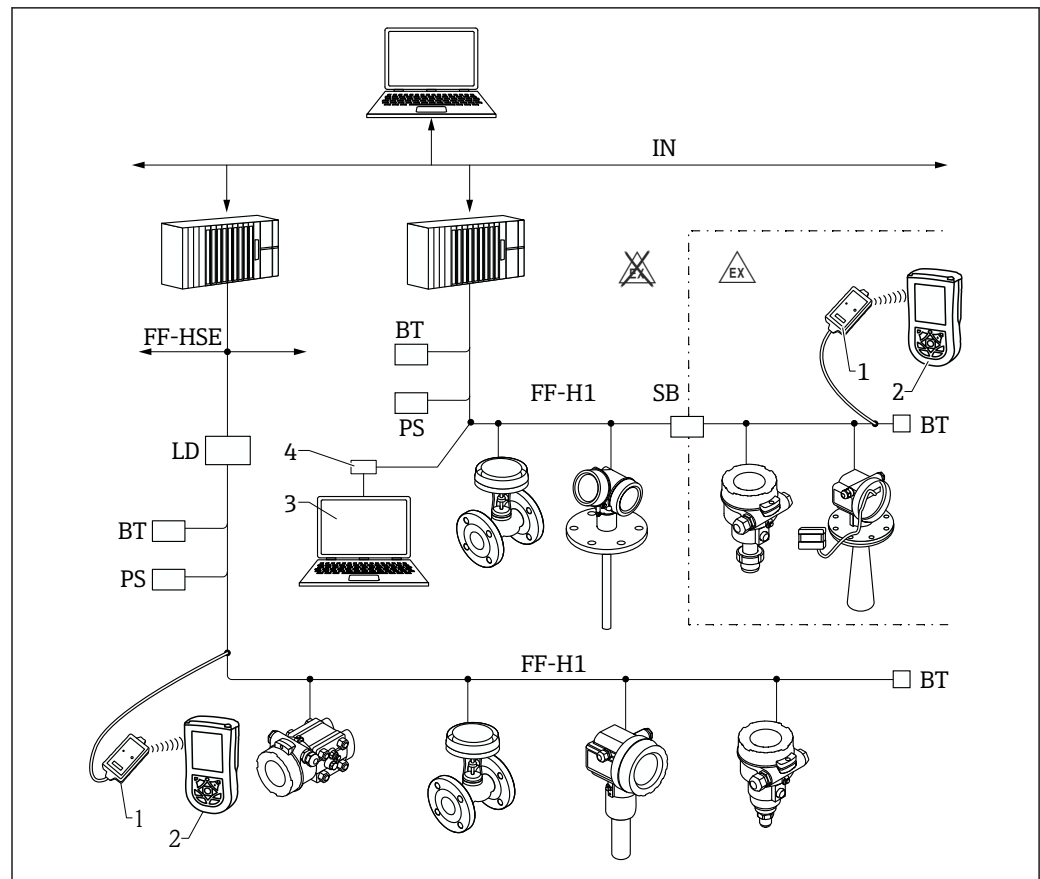
图 46 FOUNDATION Fieldbus 系统架构及组件
