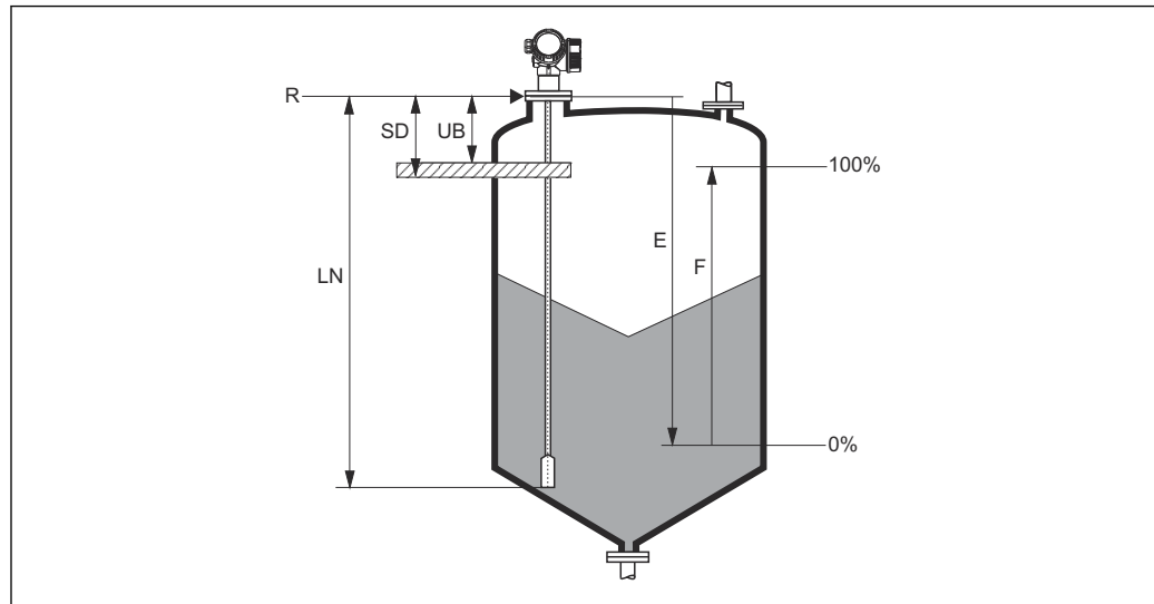
图 5 确定盲区距离和安全距离
