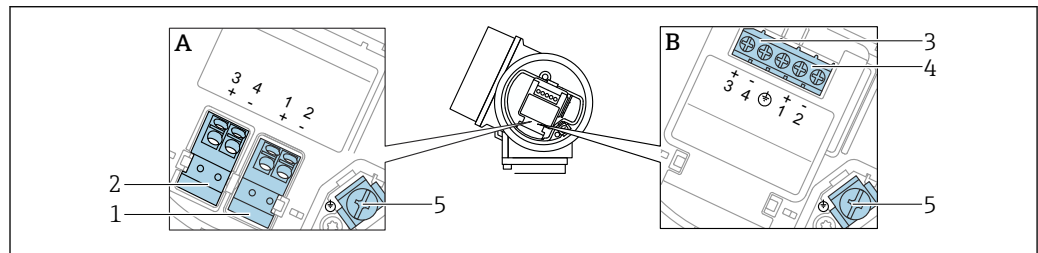
图 18 接线端子分配：PROFIBUS PA / FOUNDATION Fieldbus
