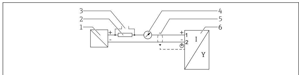
图 7 功能框图：4 ... 20 mA HART
