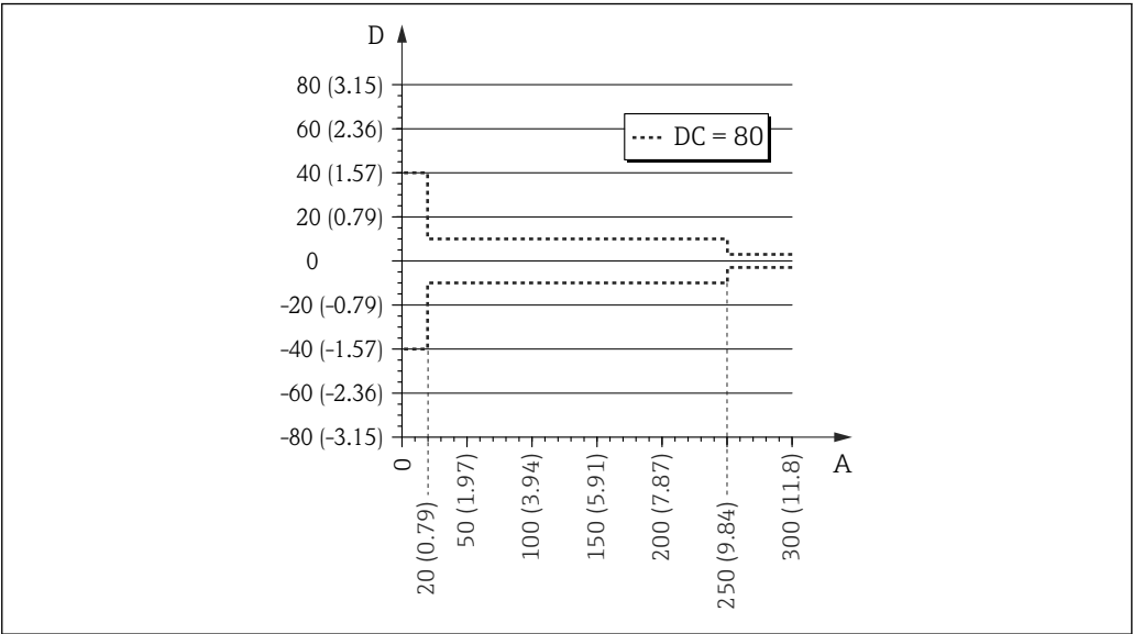
23 缆式探头底部附近的测量误差
