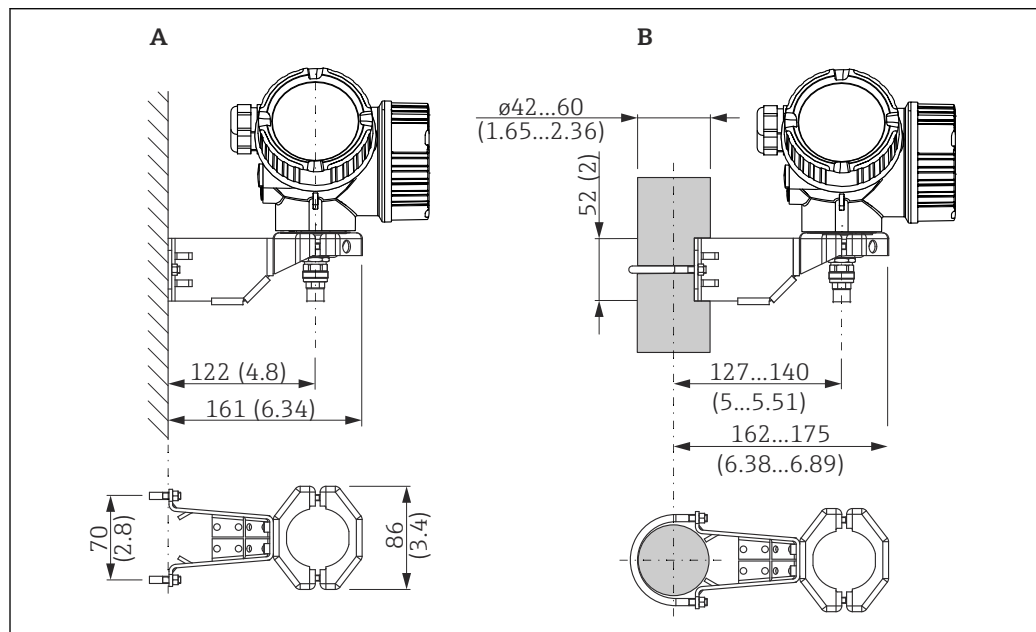
图 54 电子腔外壳安装架; 单位: mm (in)
