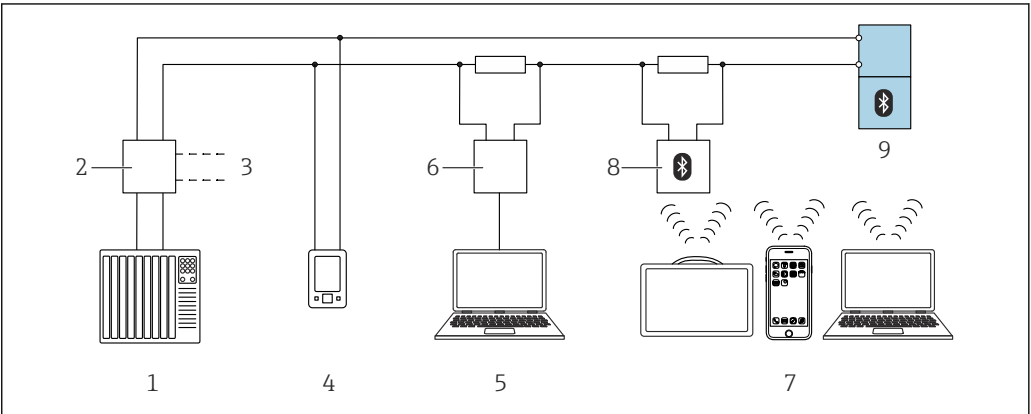
45 通过 HART 通信实现远程操作
