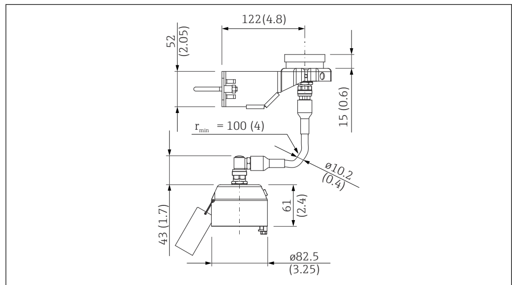
图 37 分体式探头连接件；连接电缆长度为订购长度。测量单位 mm (in)
