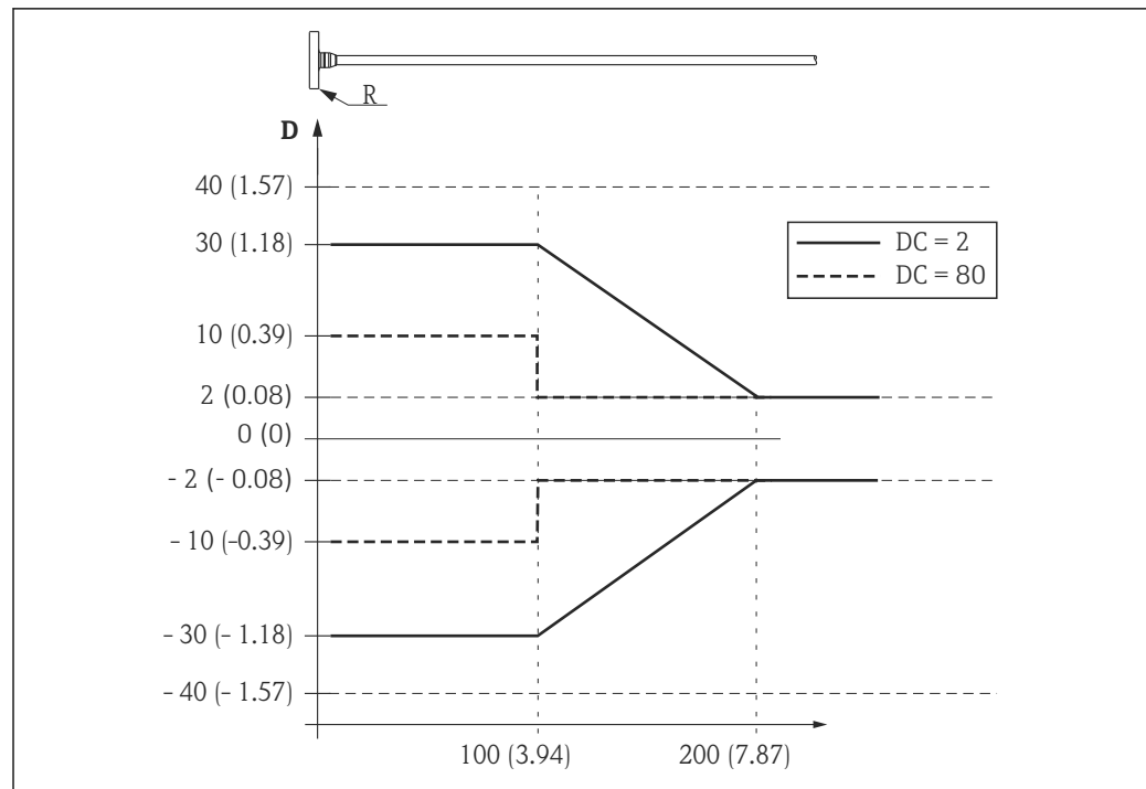
图 24 探头顶部出现的测量误差；单位：mm (in)
