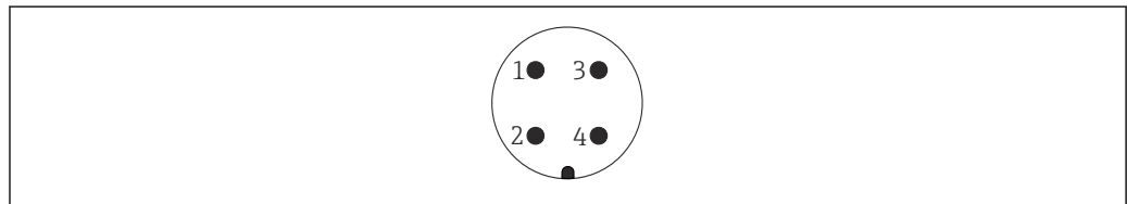
21 Atribuição de pinos do conector 7/8"
