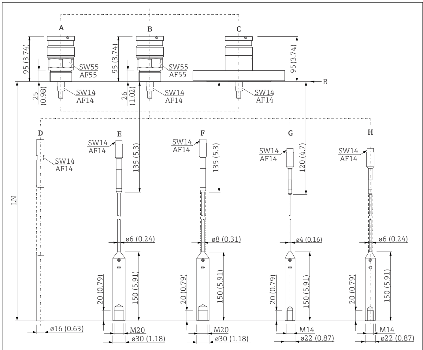
39 FMP57: Conexão do processo/haste. Unidade de medida mm (in)
