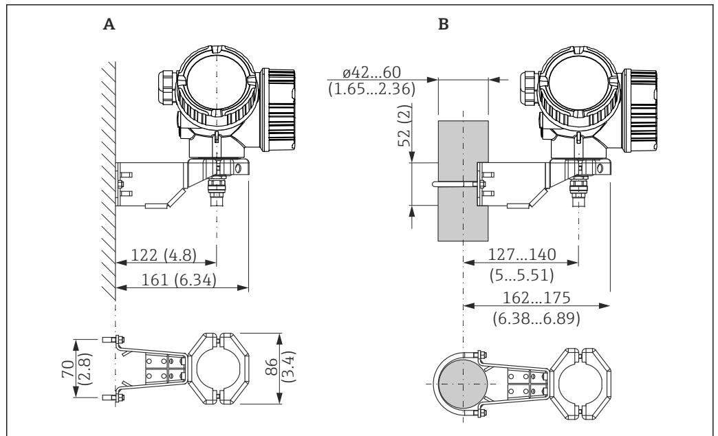
54 Suporte de montagem para invólucro dos componentes eletrônicos; unidade: mm (pol.)
