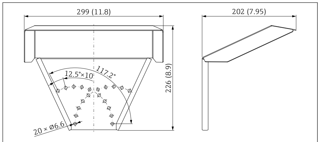
53 Dimensões. Unidade de medida mm (in)
