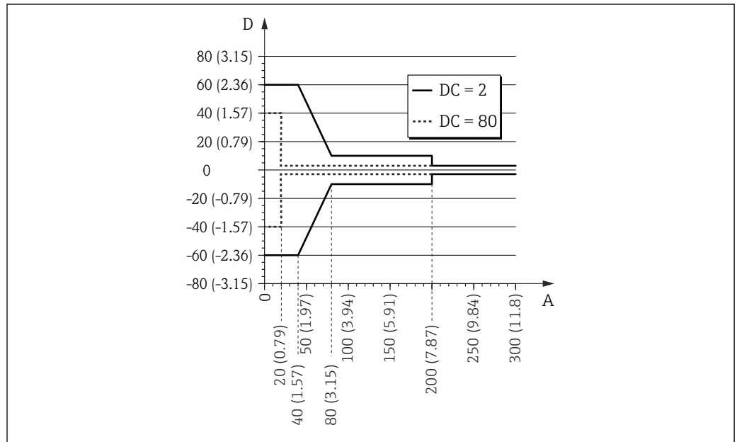
22 Erro de medição na extremidade da sonda para hastes rígidas e sondas coaxiais
