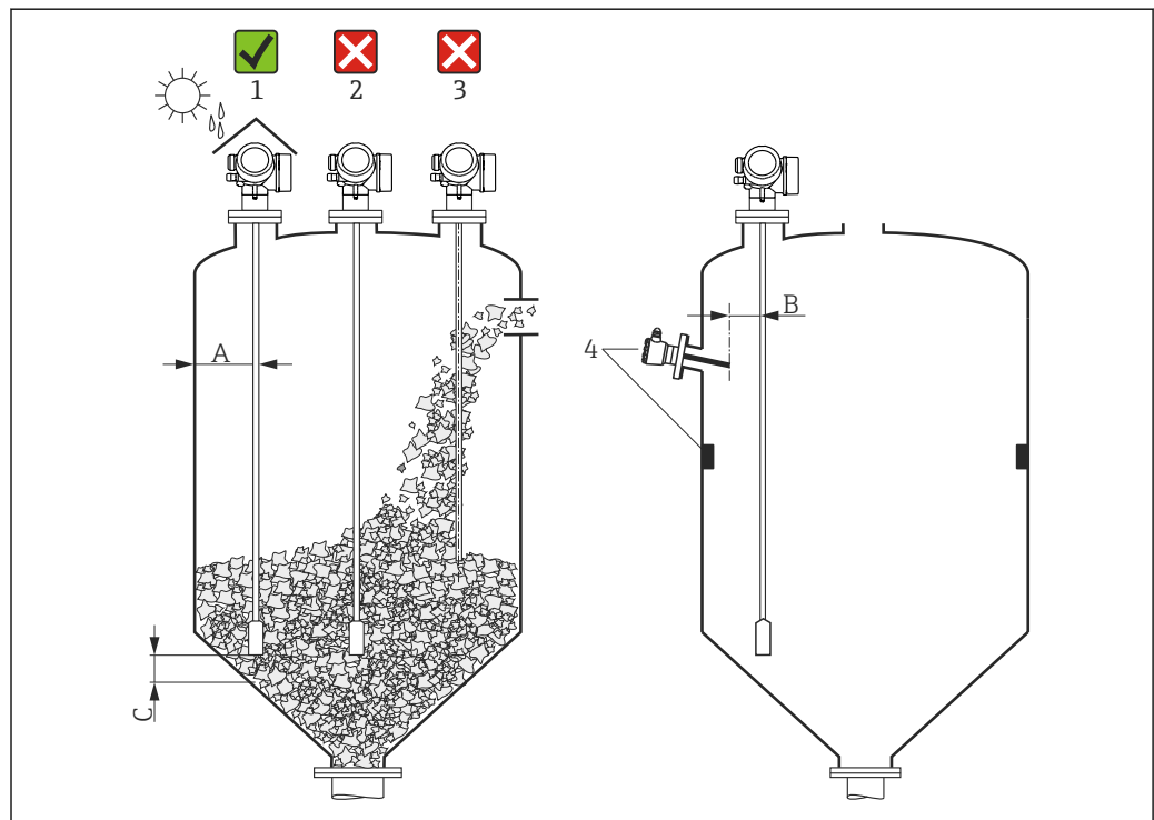
25 Posições de instalação
