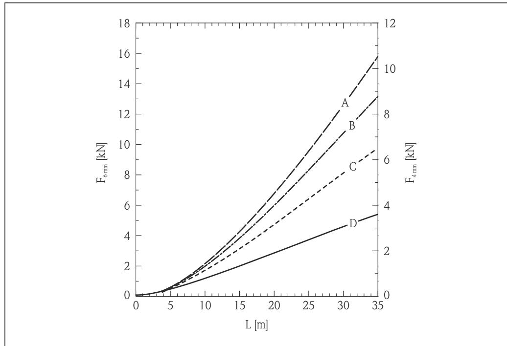
27 Pellets de polietileno em silo metálico com paredes lisas; carga de tração como uma função do nível L para diâmetros da haste flexível de 6 mm (0.24 in) e 4 mm (0.16 in)
