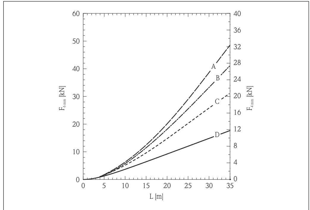
26 Areia de sílica em silo metálico com paredes lisas; carga de tração como uma função do nível L para diâmetros da haste flexível de 6 mm (0.24 in) e 4 mm (0.16 in)
