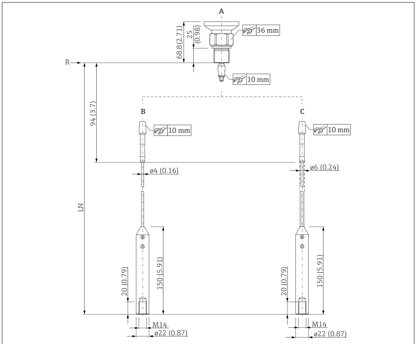
38 FMP56: Conexão do processo/sonda. Unidade de medida mm (in)
