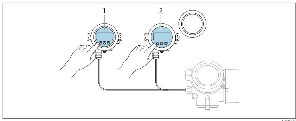
44 Opções de funcionamento do FHX50
