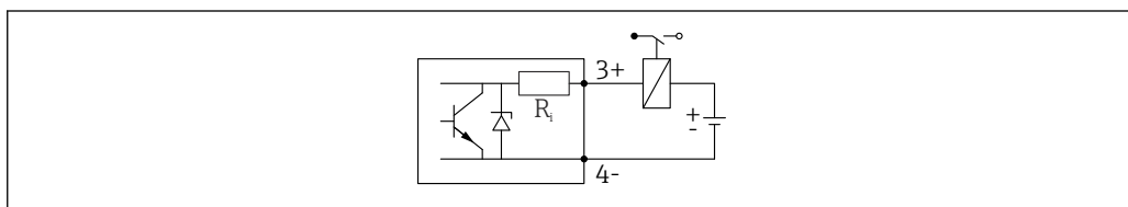
11 Пример подключения реле
