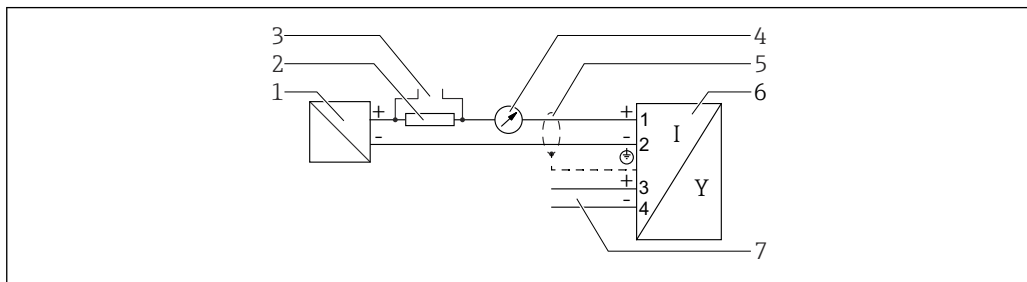
10 Функциональная схема 4 до 20 мА HART, релейный выход
