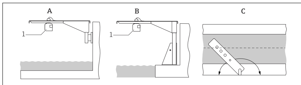
A Support d'angle avec bras de montage et support mural B Support d'angle avec bras de montage et traverse de montage C Le support d'angle peut être pivoté pour positionner le capteur au-dessus du centre du canal 1 Capteur
