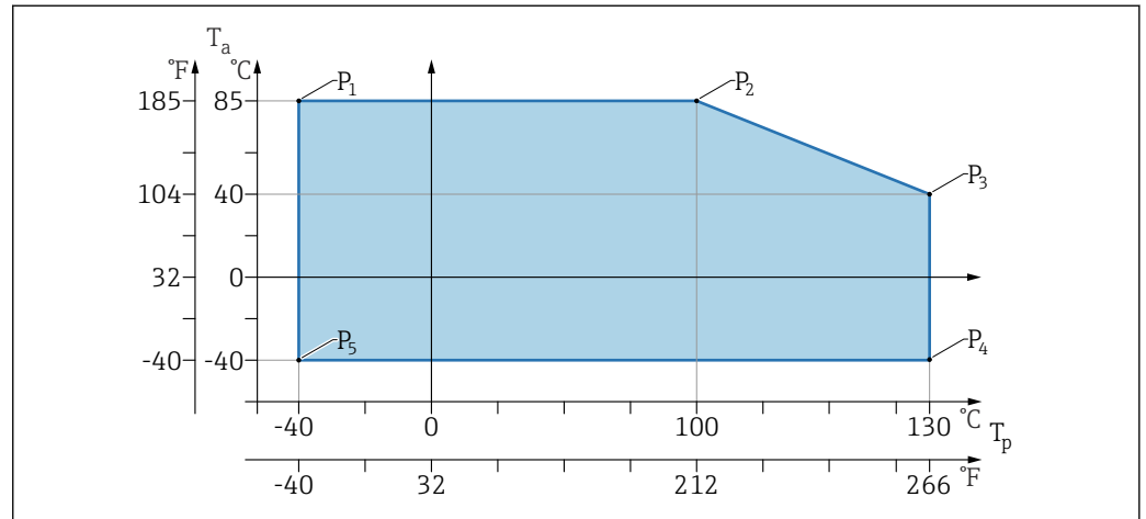
4 Température ambiante T_a dépendant de la température de process T_p
