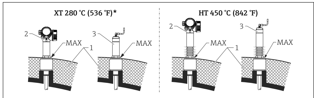
図 39 プロセス接続 (ネジ) - センサバージョン XT および HT
