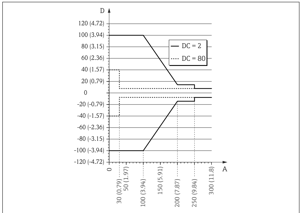
31 金属製センターリングディスクの場合のプローブ先端での測定誤差（製品構成：仕様コード 610「取付アクセサリ」、バージョン OA、OB または OC）
