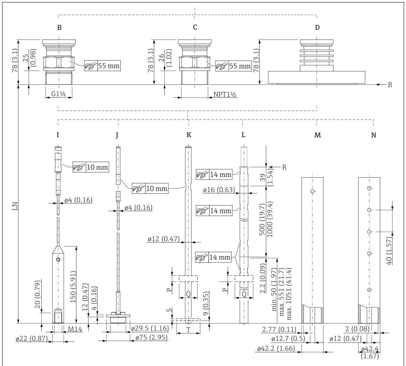
図 47 FMP51 : プロセス接続部/プローブ。測定単位 mm (in)
