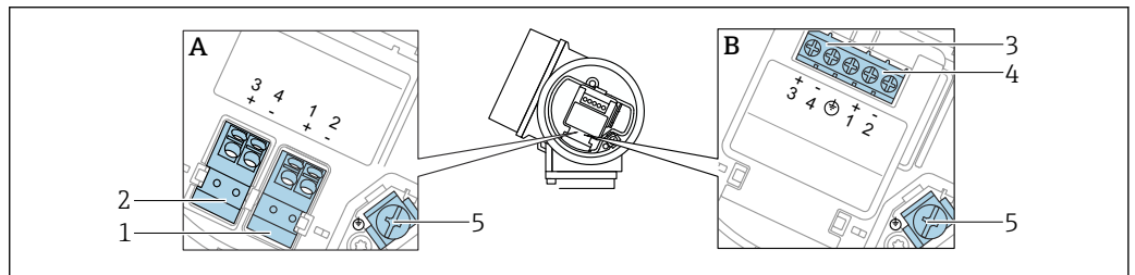
☐ 24 端子の割当て PROFIBUS PA / FOUNDATION フィールドバス
