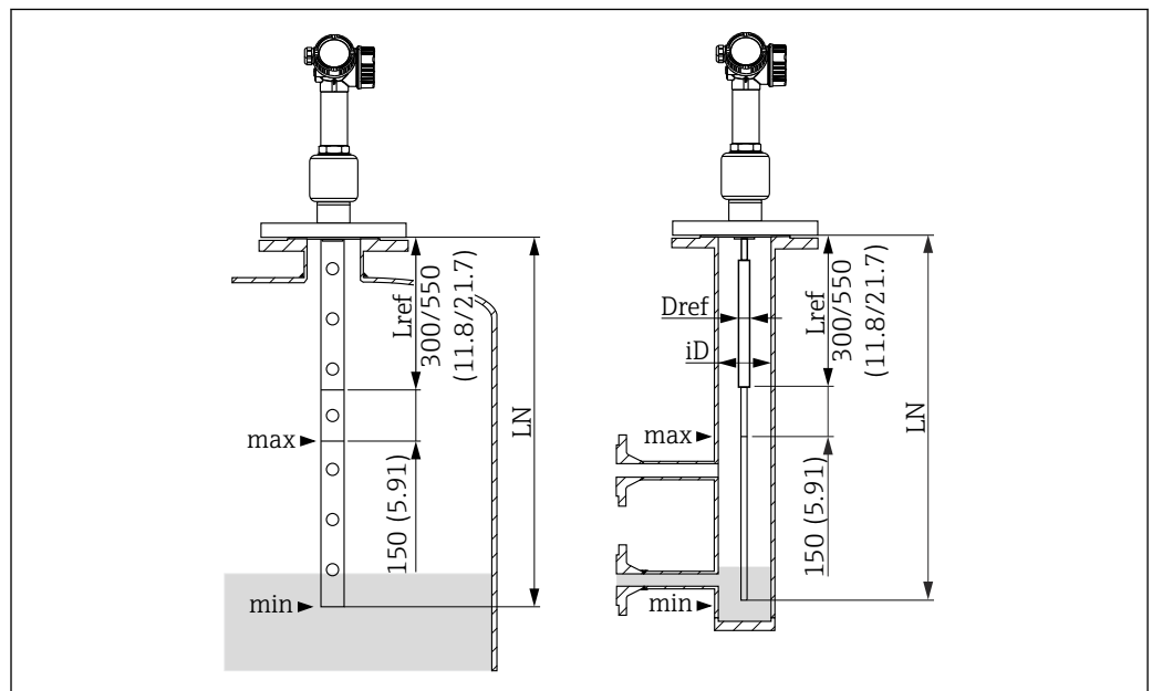
図 33 気相補正用の基準信号を備えた FMP54 ; 単位 : mm (in)
