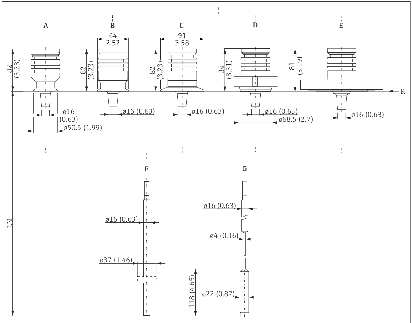
49 FMP52 : プロセス接続部/プローブ。測定単位 mm (in)
