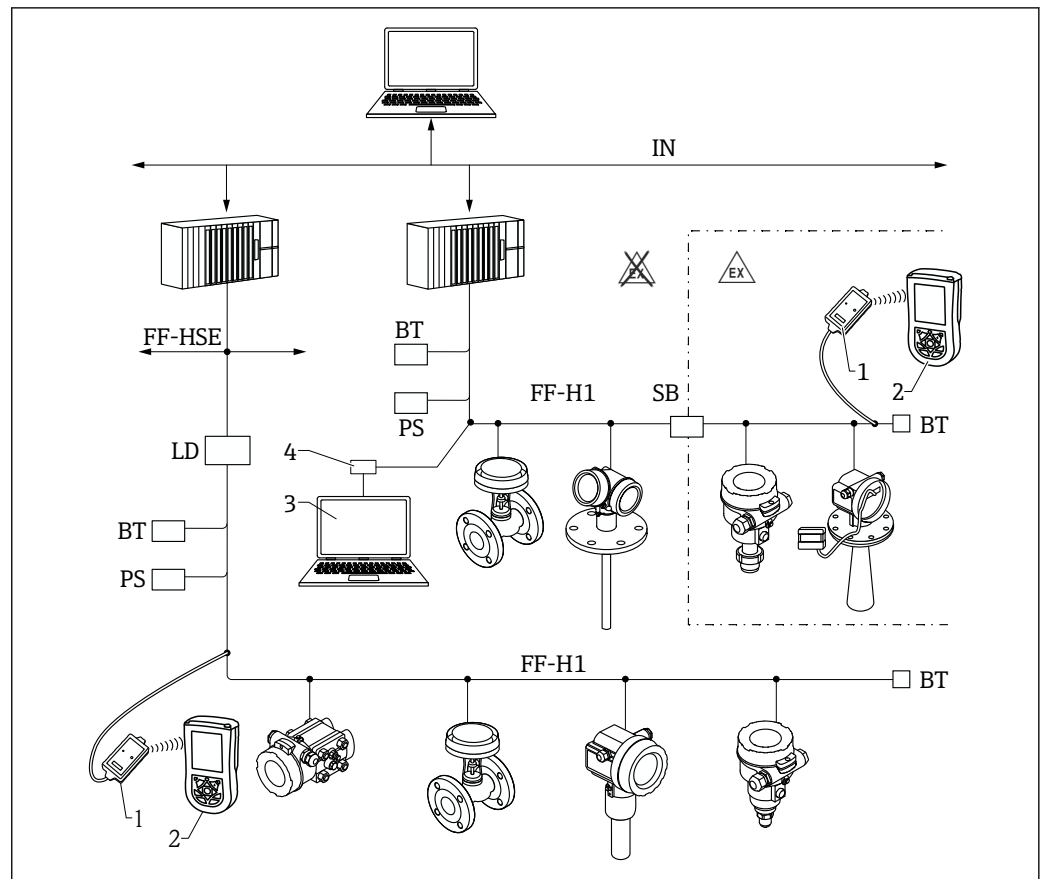
図 57 FOUNDATION フィールドバスシステム構成および関連するコンポーネント
