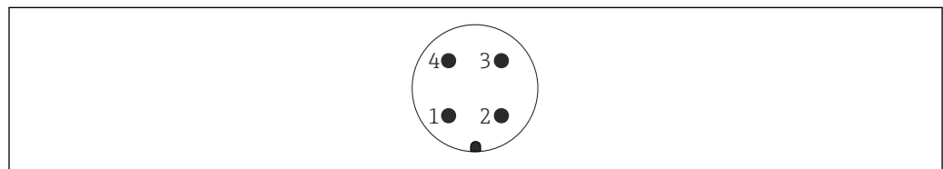
図 27 M12 プラグのピン割当て
