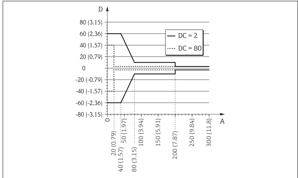
図 29 ロッドプローブおよびコアキシャルプローブのプローブ終端での測定誤差
