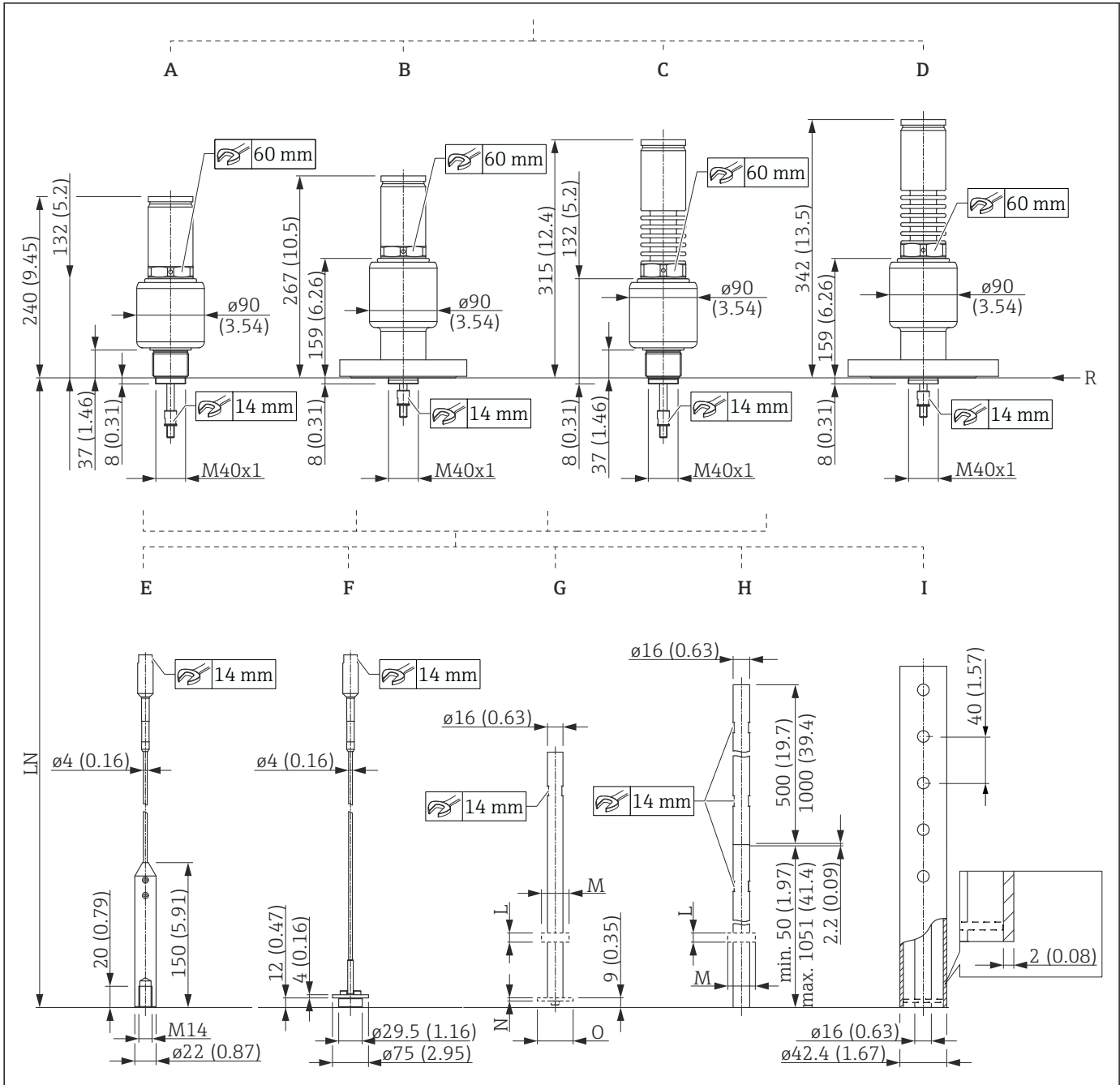
50 FMP54 : プロセス接続部/プローブ。測定単位 mm (in)
