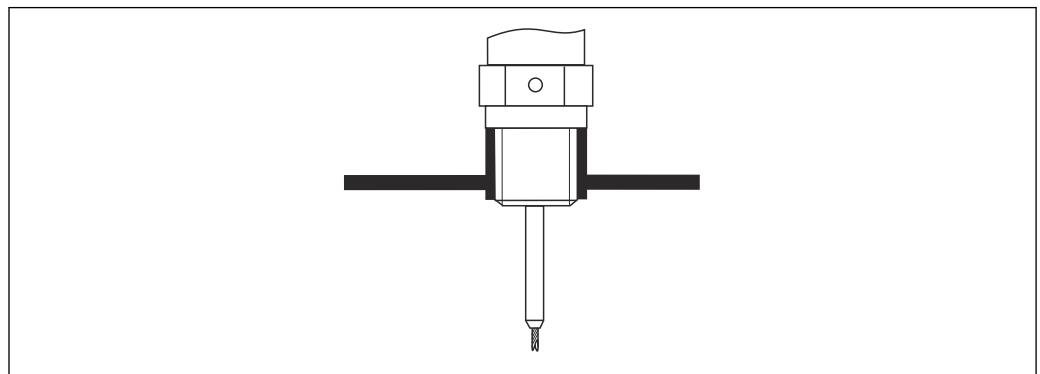
図 35 ネジ込み接続による取付け；容器天井と同一平面上
