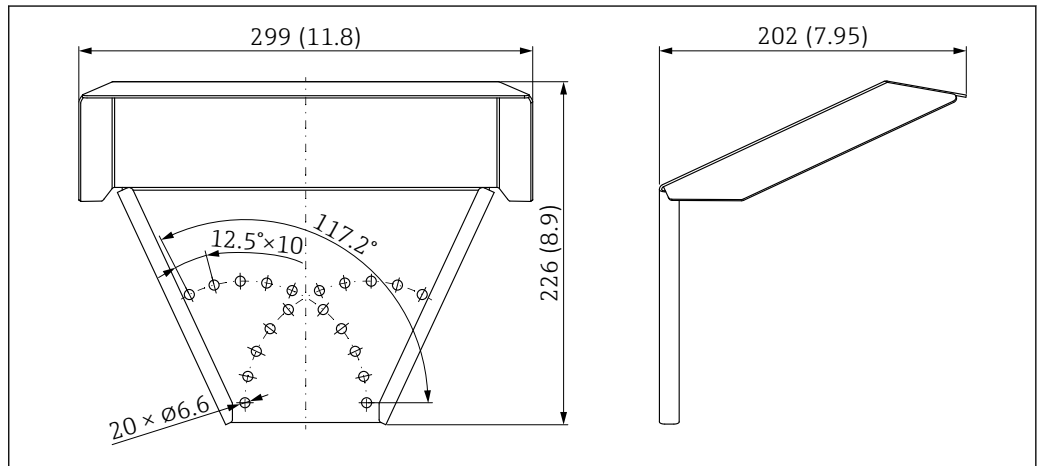
図 65 寸法。測定単位 mm (in)
