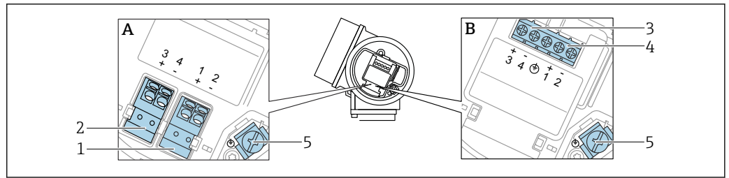
☐ 18 端子の割当て、2線式：4～20 mA HART、4～20 mA
