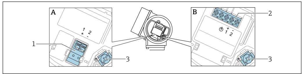
図 12 端子の割当て、2線式：4～20 mA HART
