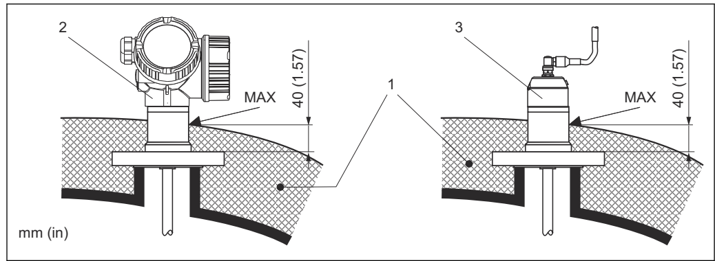
図 38 プロセス接続 (フランジ)
