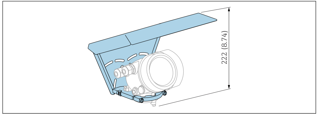
図 64 高さ。測定単位 mm (in)
