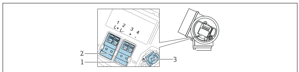
☐ 20 端子の割当て、4線式：4～20 mA HART (10.4～48 V DC )
