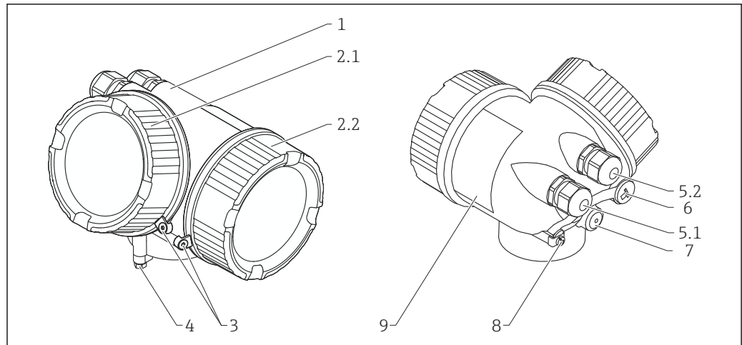
図 53 材質：GT20ハウジング
