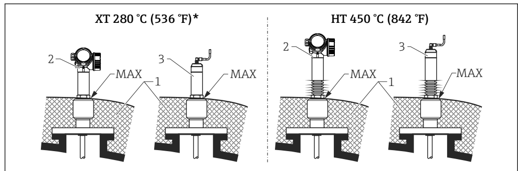
図 40 プロセス接続 (フランジ) - センサバージョン XT および HT
