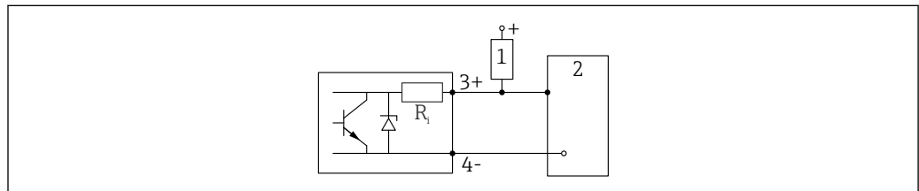
図 17 デジタル入力の接続例
