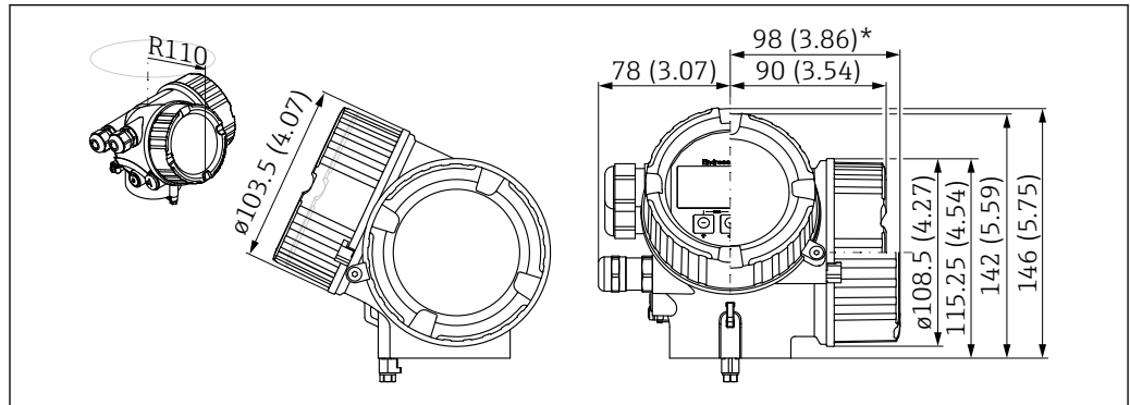
図 41 ハウジング GT18 (SUS 316L 相当)。測定単位 mm (in)
