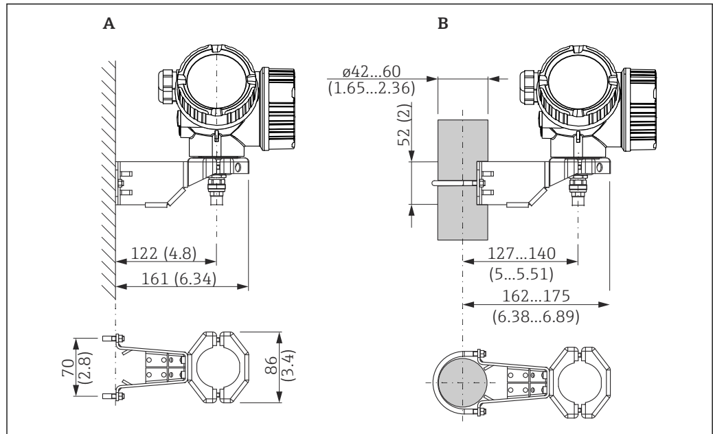
図 66 電子部ハウジングの取付ブラケット、単位：mm (in)
