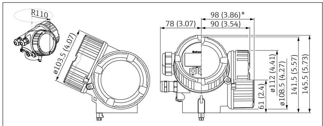
図 43 ハウジング GT20 (アルミダイカスト、塗装)。測定単位 mm (in)
