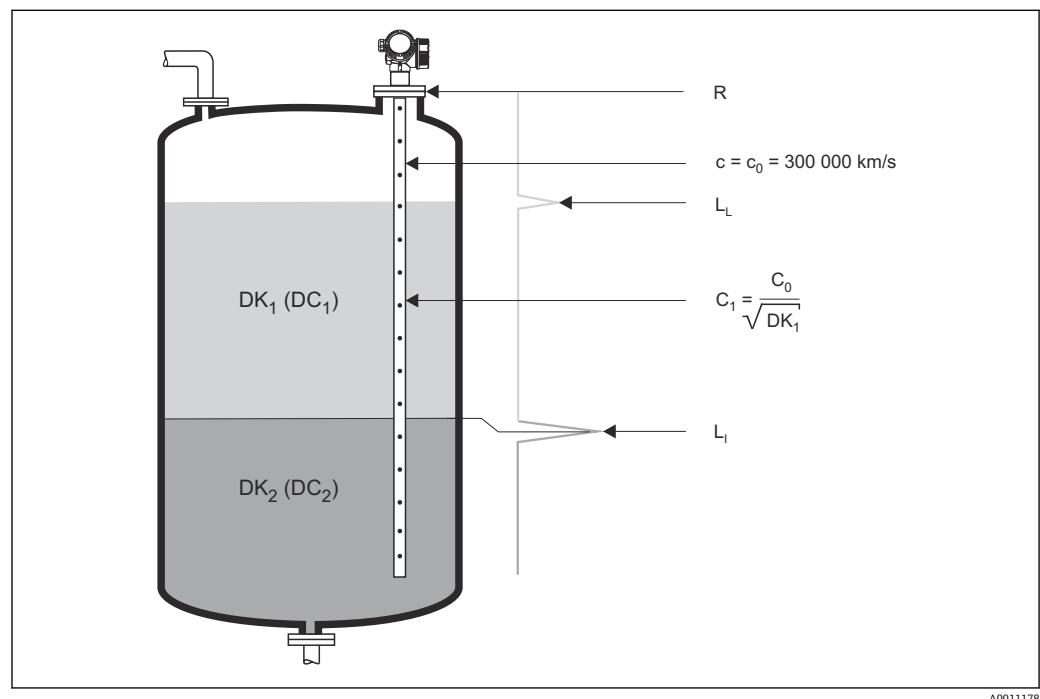
図 2 ガイドレーダーによる界面測定
