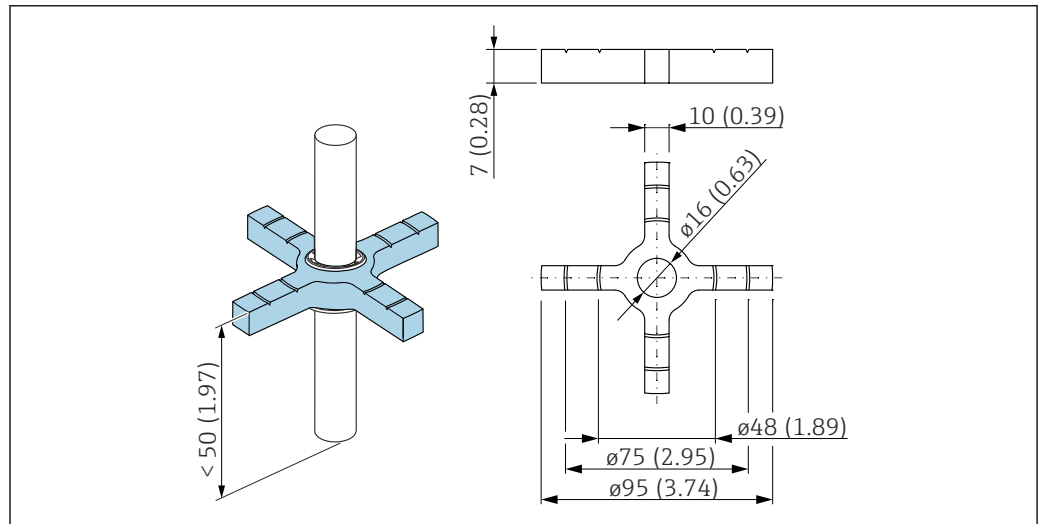
図 69 寸法；センタリングスター PEEK、ø48~95 mm (1.89~3.74 in)
