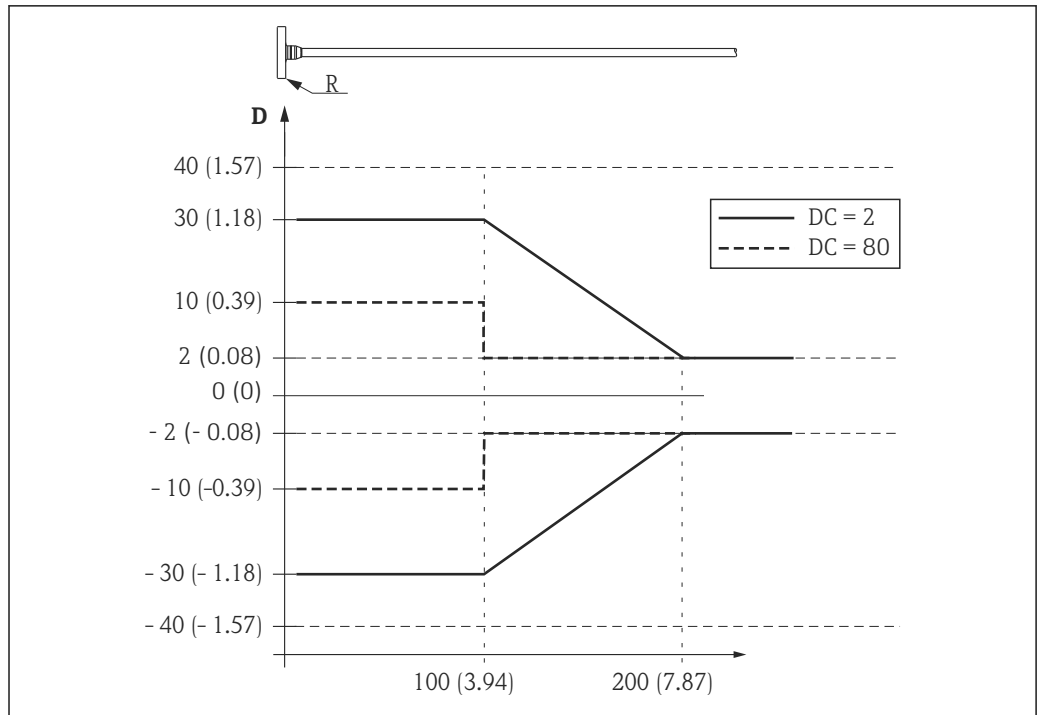
図 32 プローブ先端での測定誤差、単位 mm (in)
