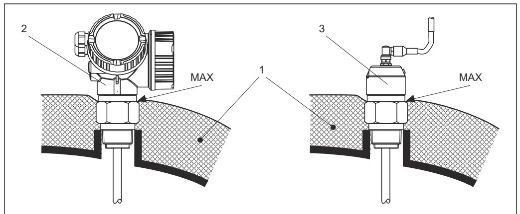
図 37 プロセス接続 (ネジ)
