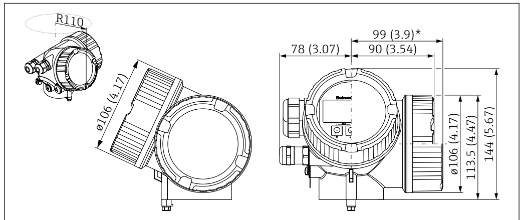
図 42 GT19 ハウジング (プラスチック PBT)。測定単位 mm (in)
