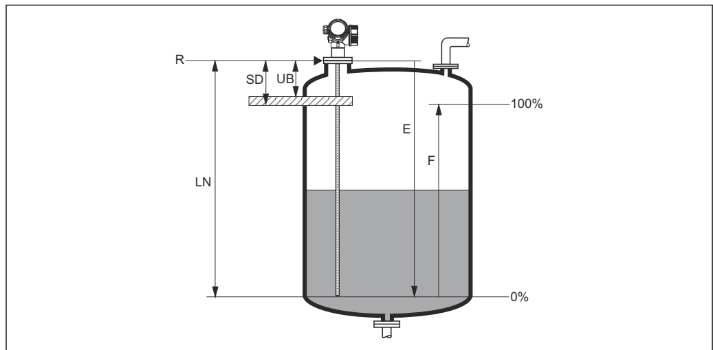
図 11 不感知距離および安全距離の定義
