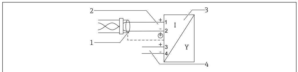
☐ 25 ブロック図：PROFIBUS PA / FOUNDATION フィールドバス
