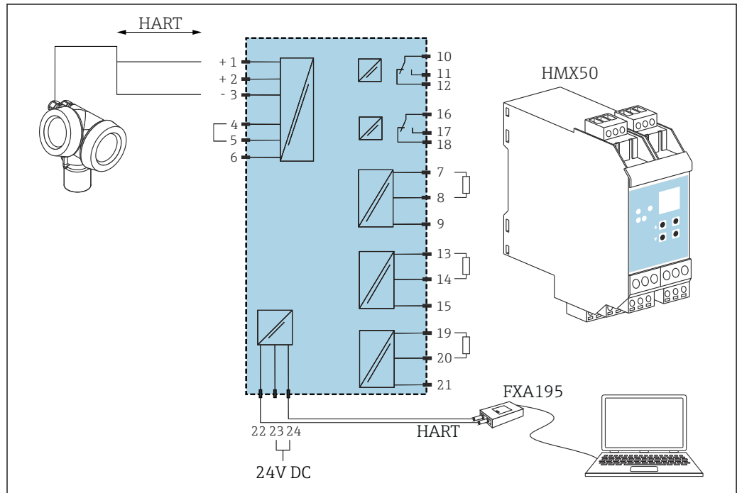
図 26 HART ループコンバータ HMX50 の接続図 (例：パッシブ 2 線機器と電流出力 (電源として接続))
