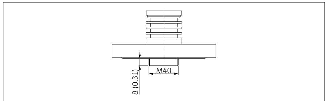
図 48 アロイ C フランジの寸法。測定単位 mm (in)
