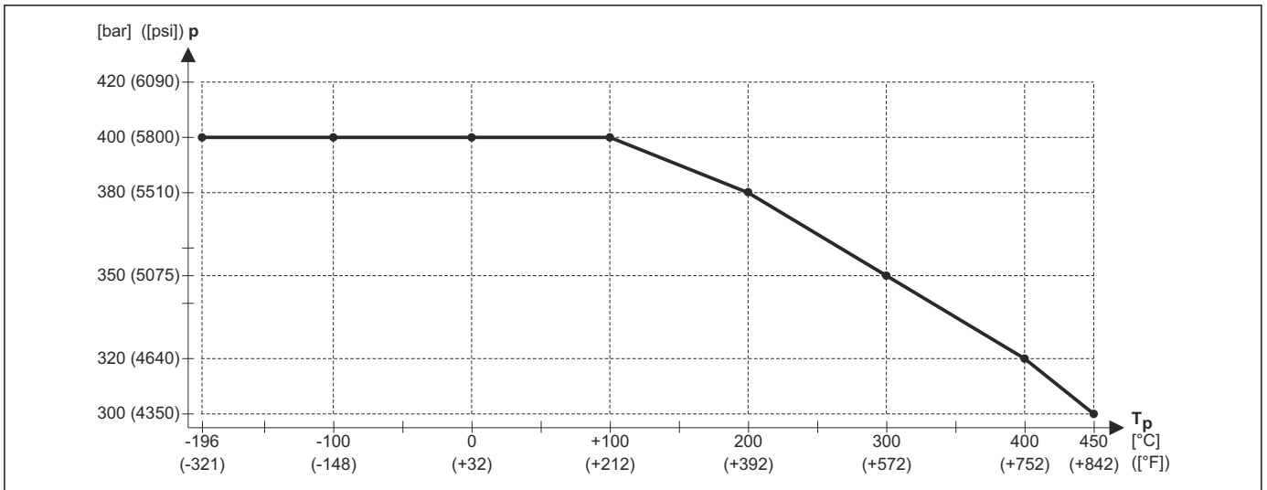
FMP54 - 許容プロセス圧力はプロセス温度に依存
