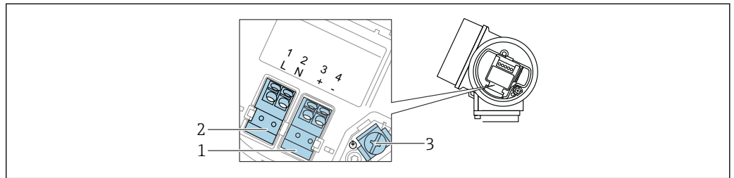
図 14 端子の割当て、4線式：4～20 mA HART（90～253 V AC ）
