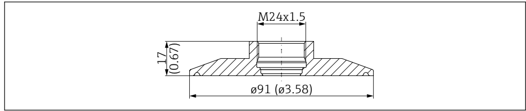
図 36 トリクランプ ISO2852 DN70-76.1 (3"), SUS 316L 相当。測定単位 mm (in)
