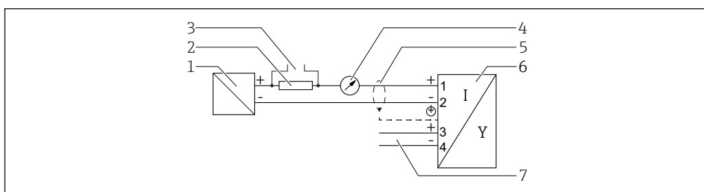
図 7 機能図：4～20 mA HART、スイッチ出力
