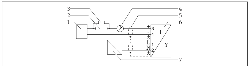
図 15 機能図、4線式：4～20 mA HART（90～253 V AC ）
