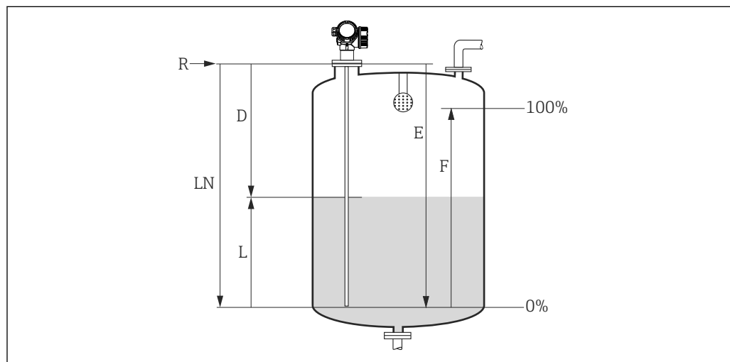
図 1 ガイドレーダーレベル計によるレベル測定のパラメータ
