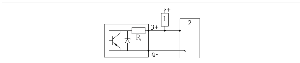
図 9 デジタル入力の接続例
