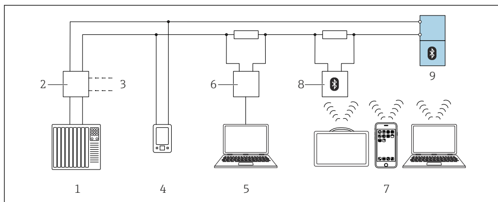
図 47 HART プロトコル経由のリモート操作オプション
