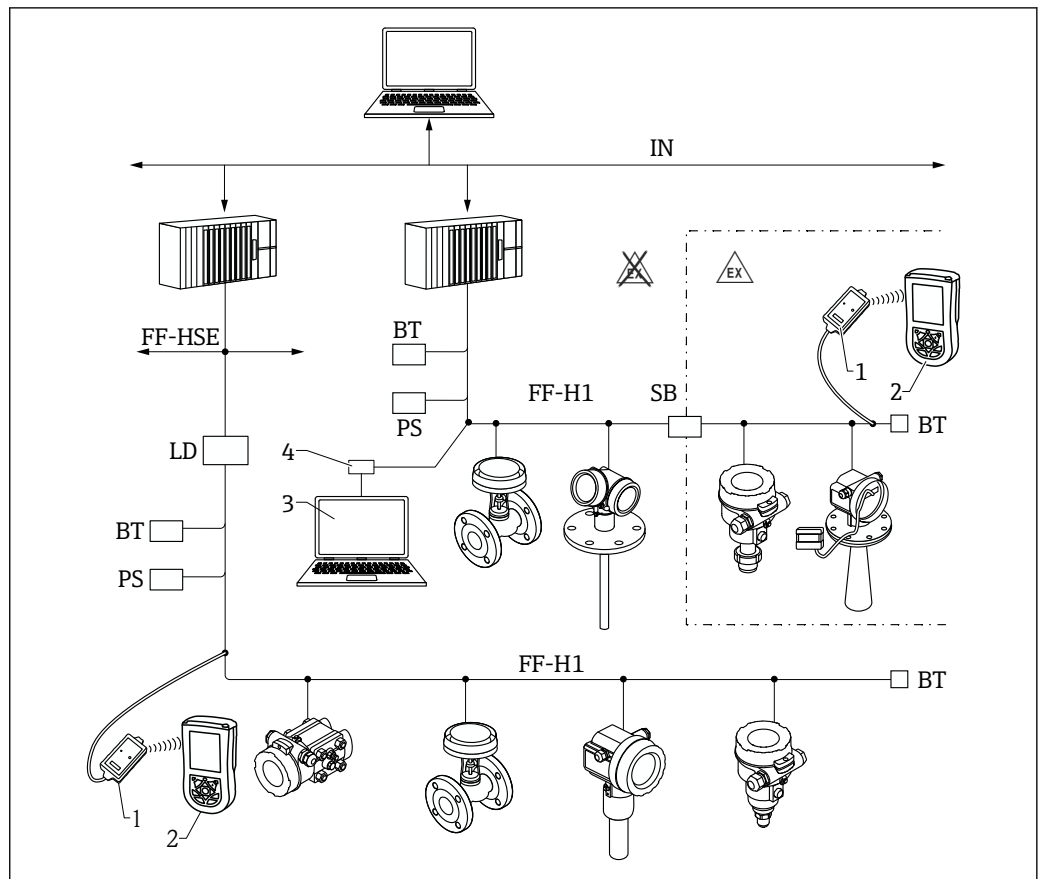
図 48 FOUNDATION フィールドバスシステム構成および関連するコンポーネント
