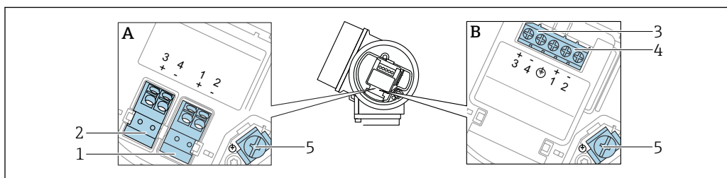
図 6 端子の割当て、2 線式：4～20 mA HART、スイッチ出力
