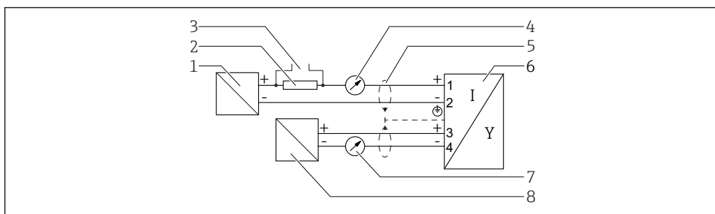
図 11 機能図：4～20 mA HART + 4～20 mA アナログ
