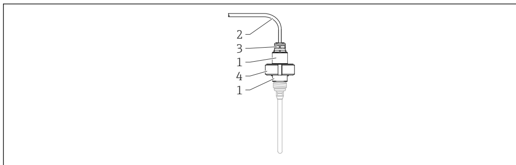
図 45 材質：「分離型センサ」バージョン用のアダプタおよびケーブル
