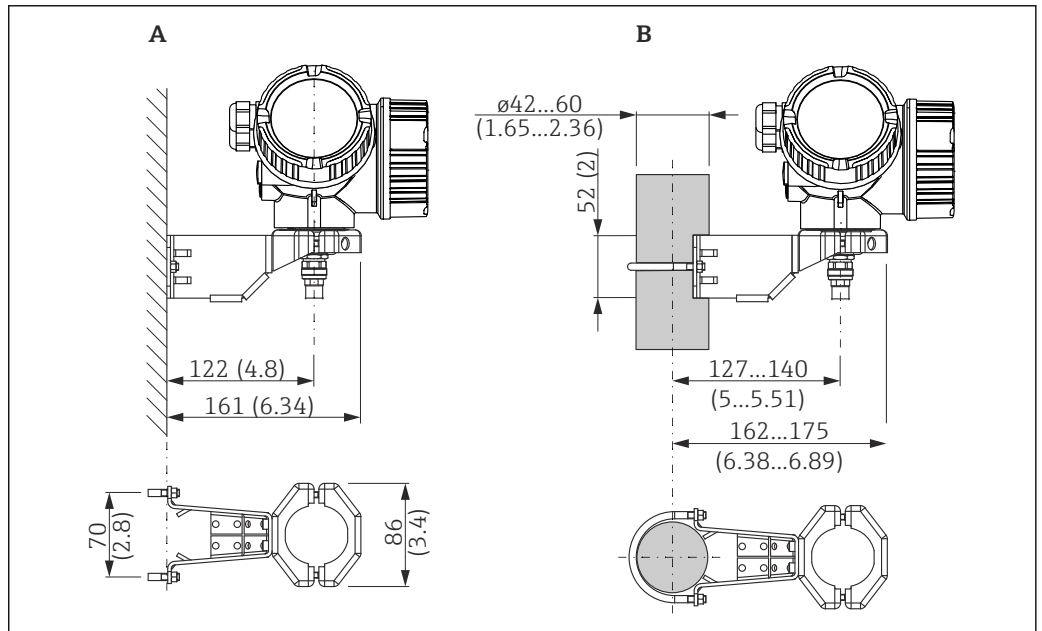
図 26 電子部ハウジングの取付ブラケット。測定単位 mm (in)
