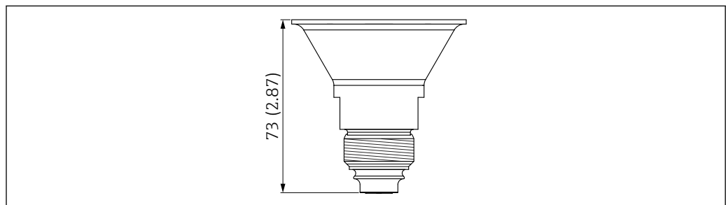
図 40 ネジ M24、SUS 316L 相当。測定単位 mm (in)
