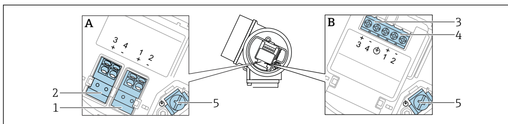
図 10 端子の割当て、2線式：4~20 mA HART、4~20 mA
