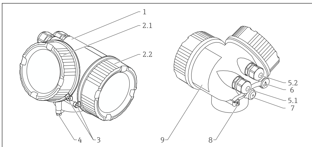
図 44 材質：GT20ハウジング
