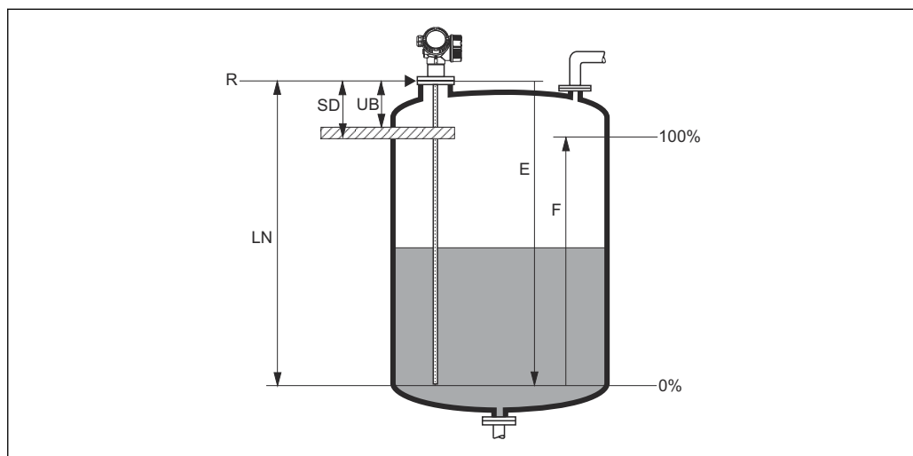
図 3 不感知距離および安全距離の定義
