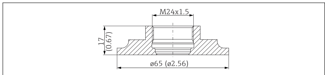
図 39 SMS 2" PN25、SUS 316L 相当。測定単位 mm (in)
