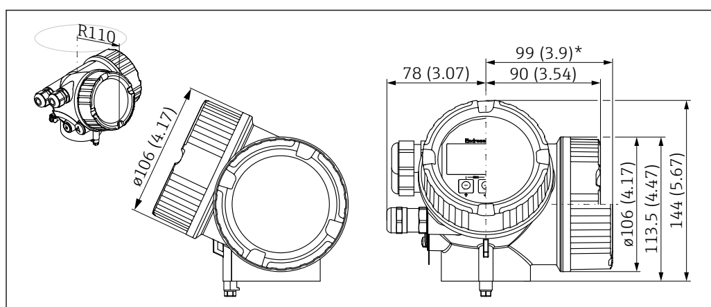
図 24 GT19 ハウジング (プラスチック PBT)。測定単位 mm (in)
