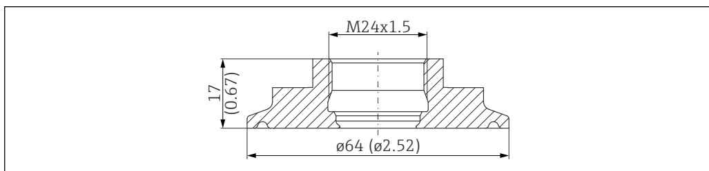
35 トリクランプ ISO2852 DN40-51 (2"), SUS 316L 相当。測定単位 mm (in)
