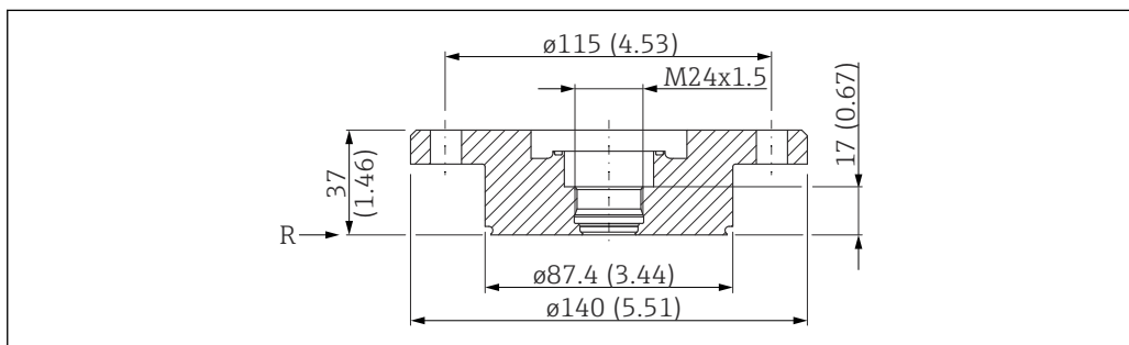
33 NEUMO バイオコントロール D80 PN16、SUS 316L 相当。測定単位 mm (in)
