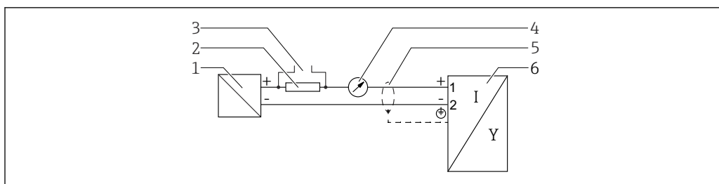
図 5 機能図：4～20 mA HART
