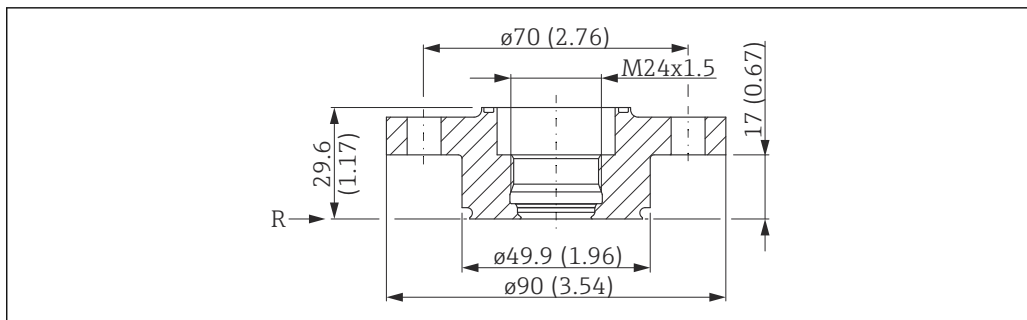
32 NEUMO バイオコントロール D50 PN16、SUS 316L 相当。測定単位 mm (in)
