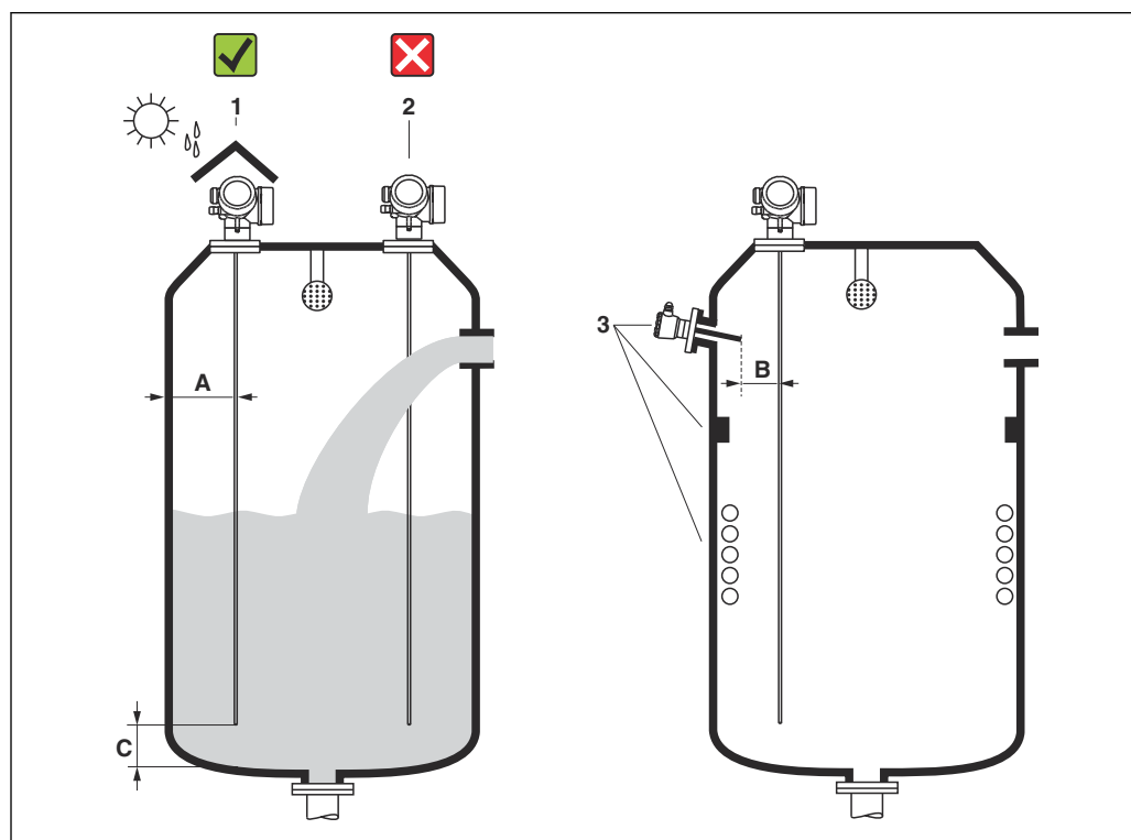
図 22 取付け位置
