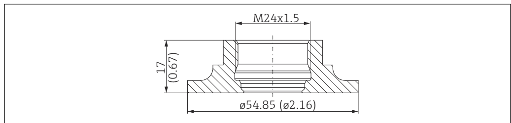
図 38 SMS 1 1/2" PN25、SUS 316L 相当。測定単位 mm (in)
