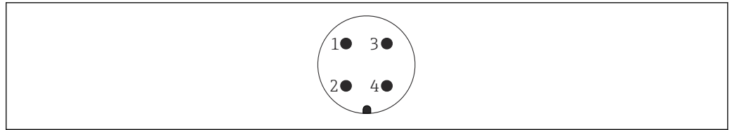
図 19 7/8" プラグのピン割当て
