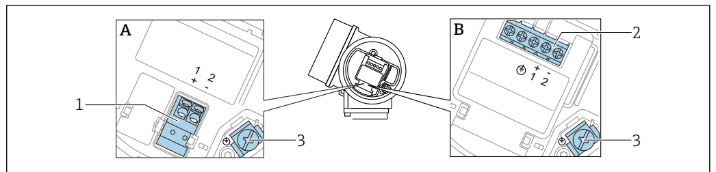
図4 端子の割当て、2線式：4~20 mA HART
