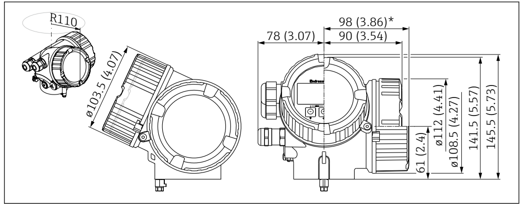
図 25 ハウジング GT20 (アルミダイカスト、塗装)。測定単位 mm (in)
