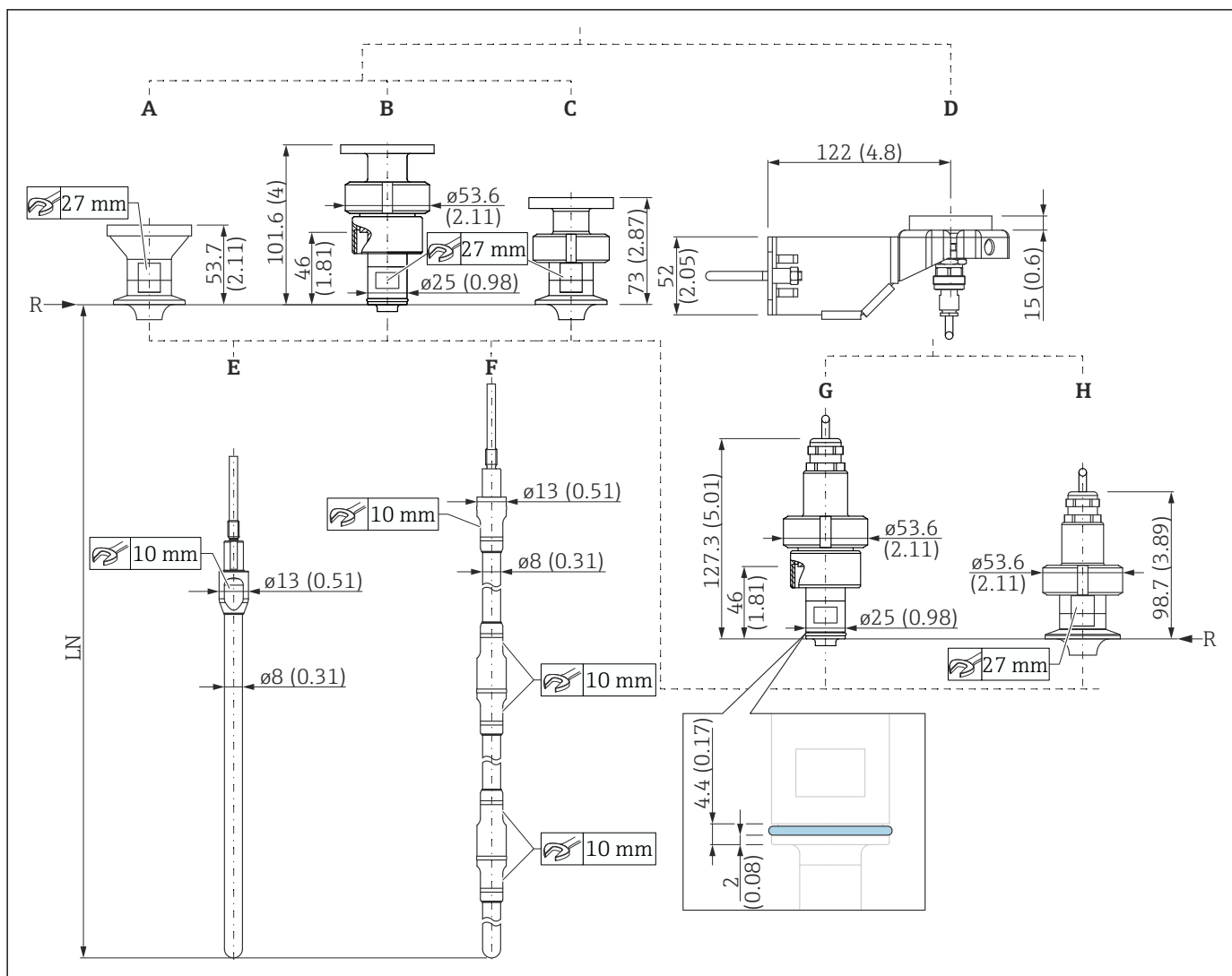
図 42 FMP53 : プローブ。測定単位 mm (in)
