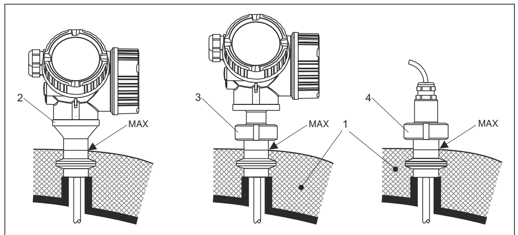
図 23 サニタリ接続
