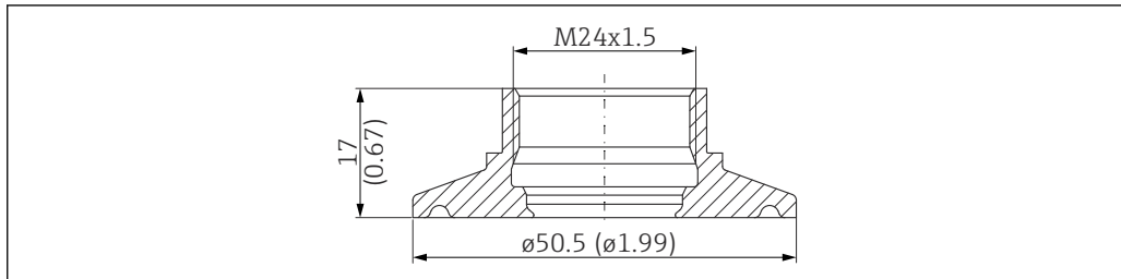
34 トリクランプ ISO2852 DN25-38 (1~1½"), SUS 316L 相当。測定単位 mm (in)
