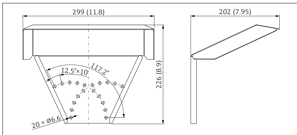
図 56 寸法。測定単位 mm (in)
