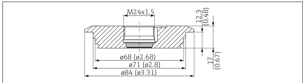
図 37 バリベント N チューブ DN40-162 PN16、SUS 316L 相当。測定単位 mm (in)
