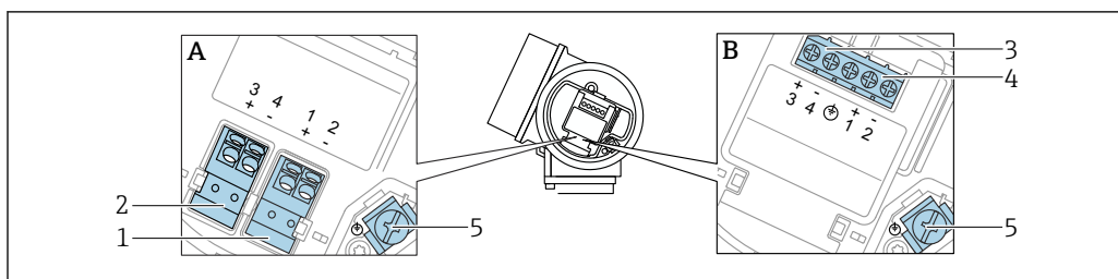
図 16 端子の割当て PROFIBUS PA / FOUNDATION フィールドバス
