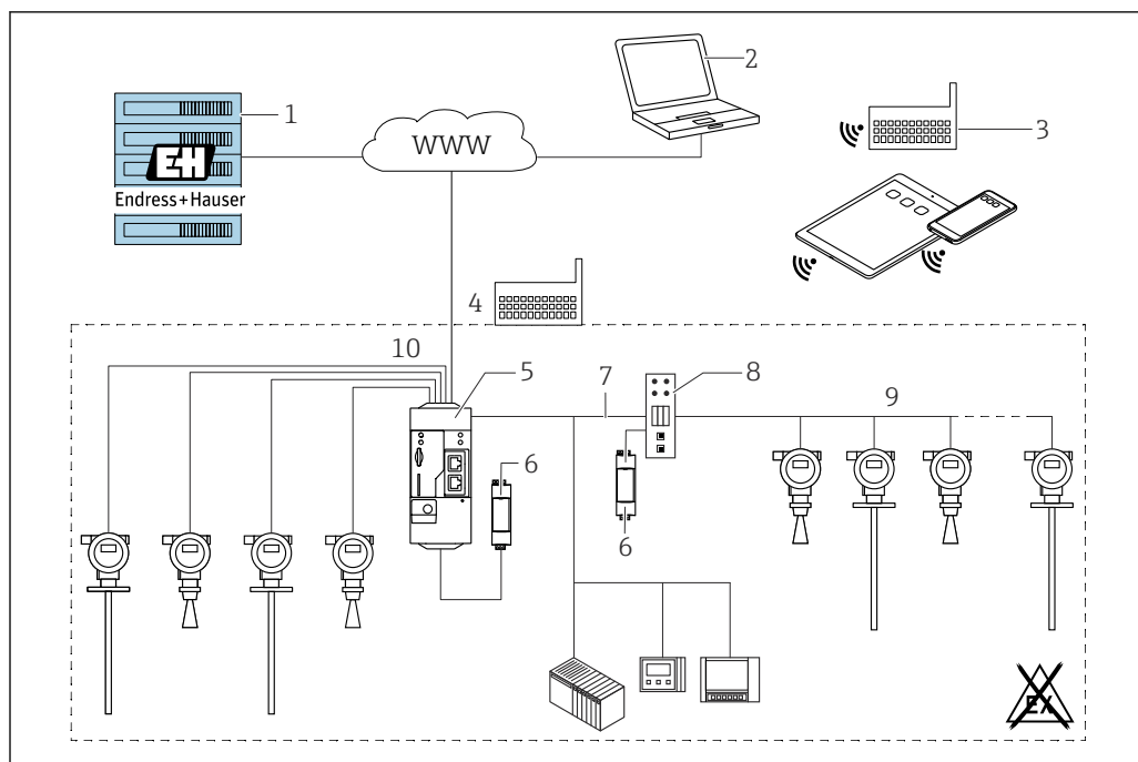
図 53 SupplyCare Hosting SCH30 を使用した在庫管理プラットフォームの例
