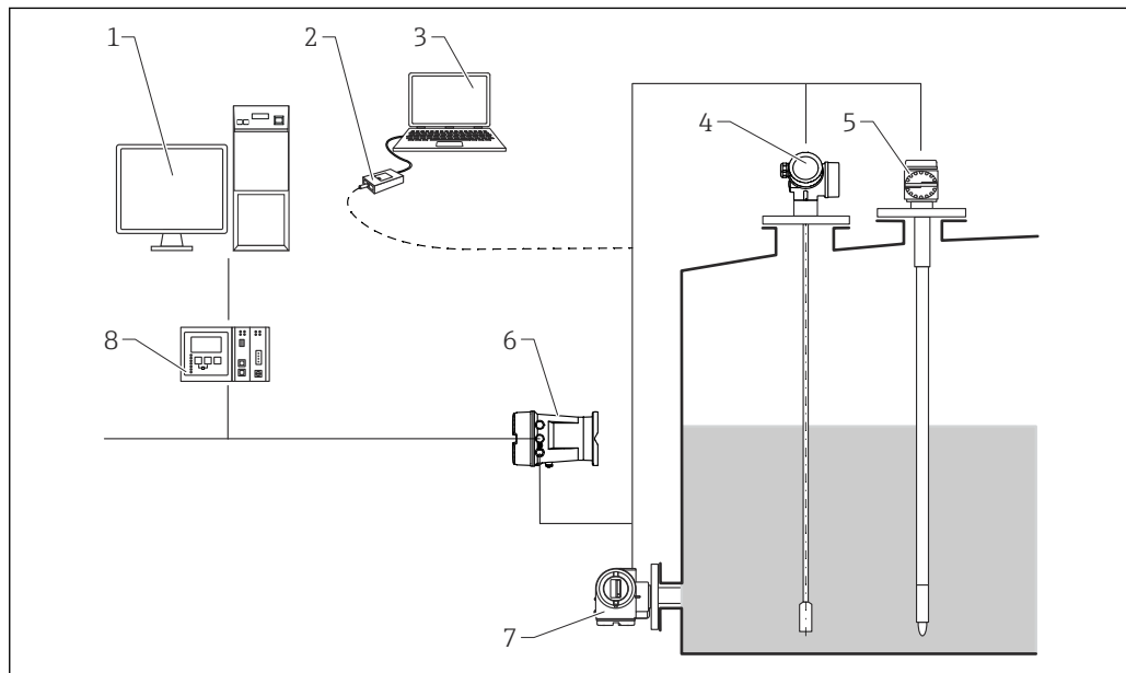
図 51 計測システム一式の構成内容：
