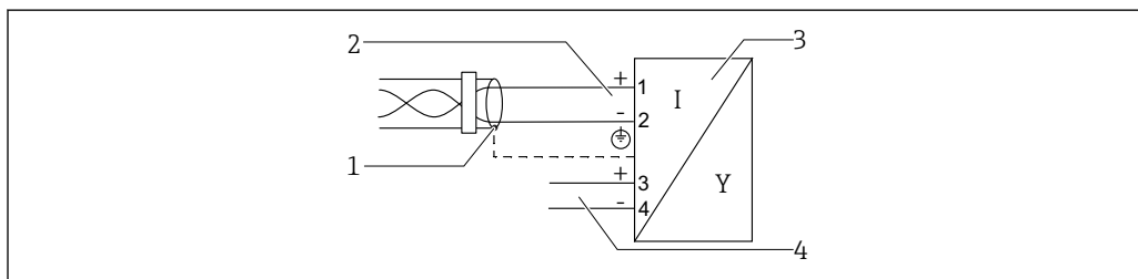
図 17 ブロック図：PROFIBUS PA / FOUNDATION フィールドバス
