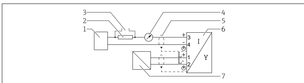
図 13 機能図、4 線式：4～20 mA HART (10.4～48 V DC )
