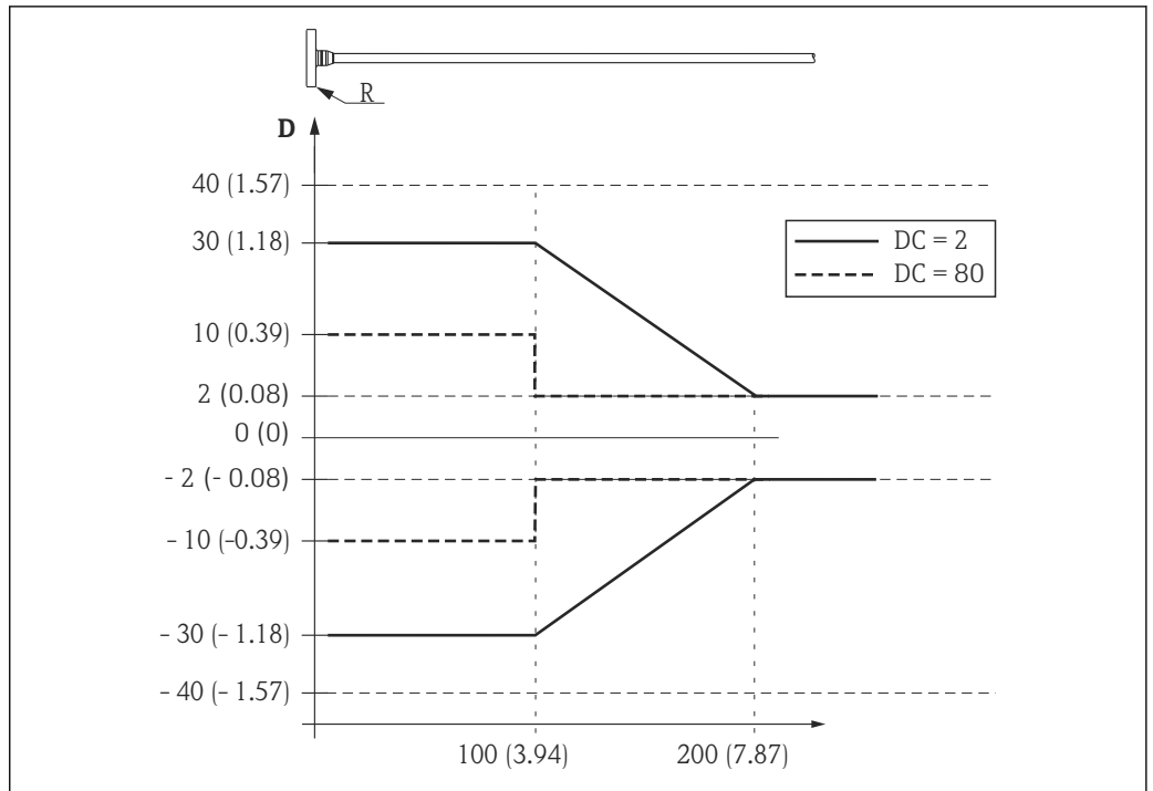
図 21 プローブ上端での測定誤差、単位 mm (in)
