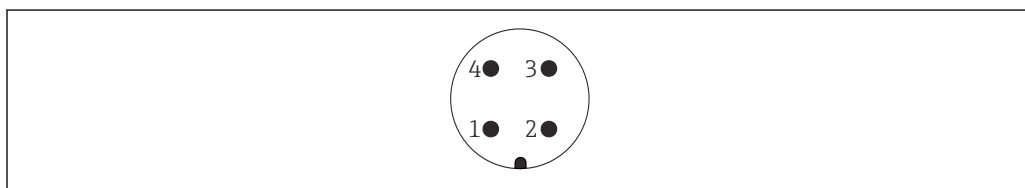
図 18 M12 プラグのピン割当て
