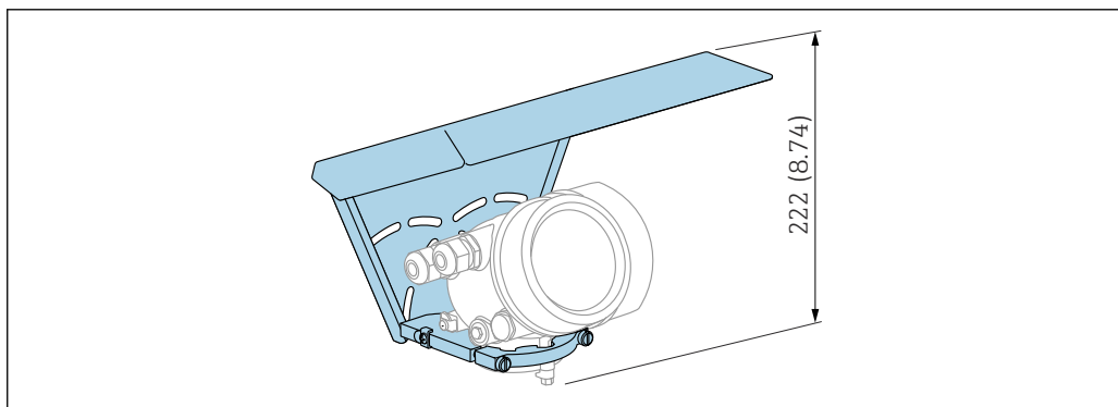
55 高さ。測定単位 mm (in)
