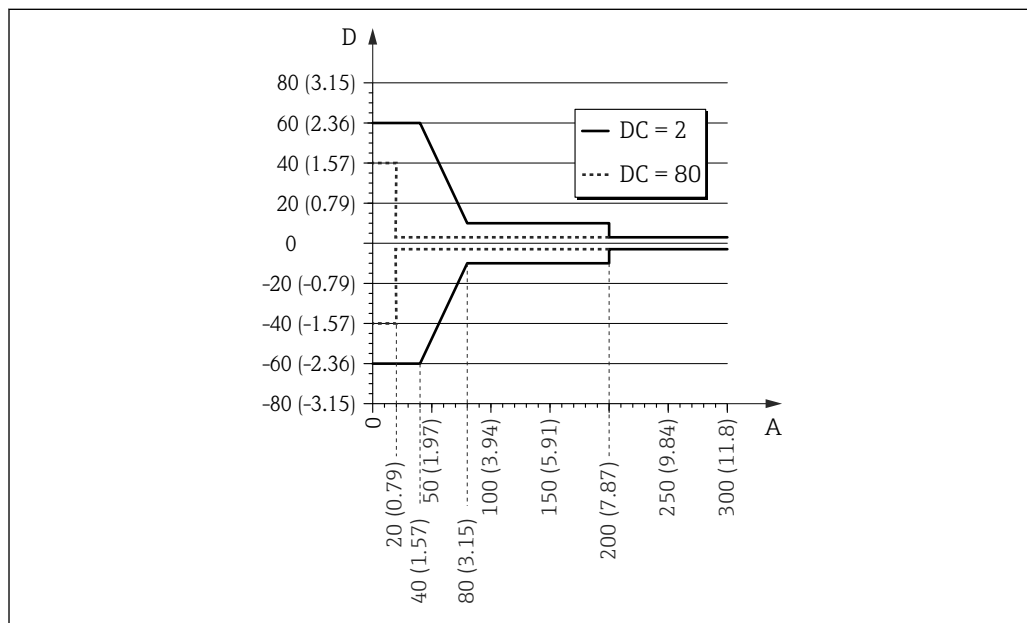
図 20 ロッドプローブおよびコアキシャルプローブのプローブ終端での測定誤差
