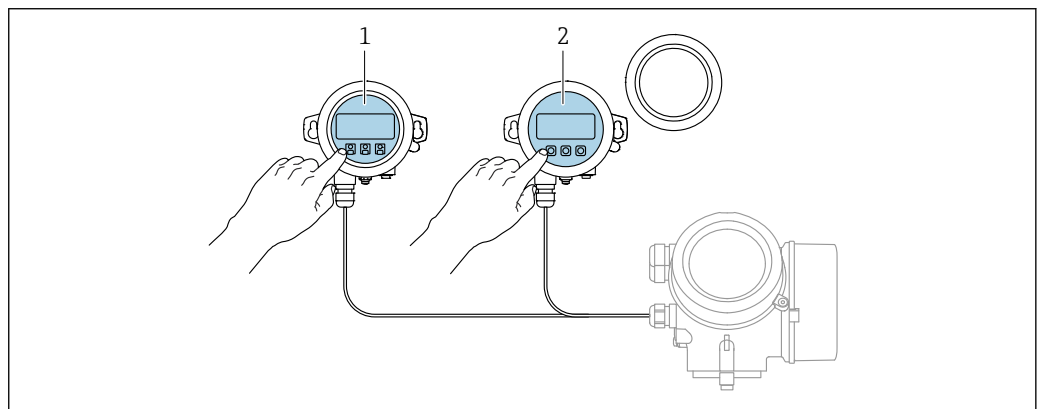
図 46 FHX50 操作オプション
