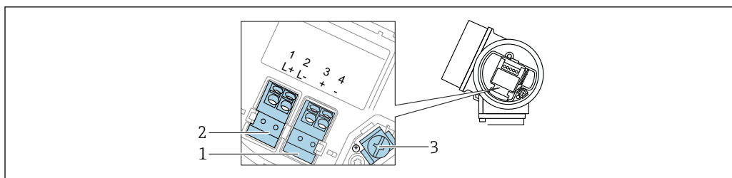
図 12 端子の割当て、4 線式：4～20 mA HART (10.4～48 V DC )
