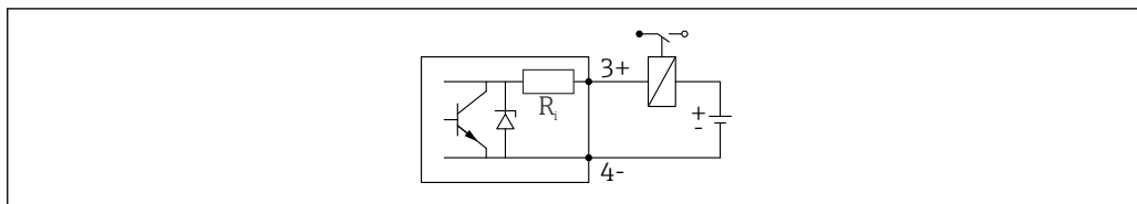
図 8 リレーの接続例
