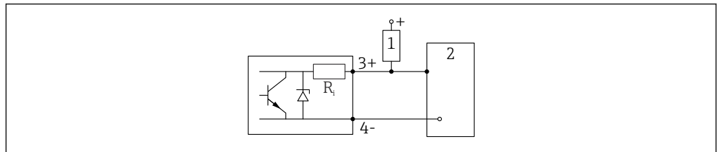
図 12 デジタル入力の接続例
