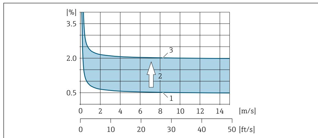
25 Exemple d'écart de mesure dans une conduite avec un diamètre nominal DN > 200 (8")
