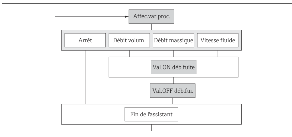
21 Assistant "Suppression des débits de fuite" dans le menu "Configuration"
