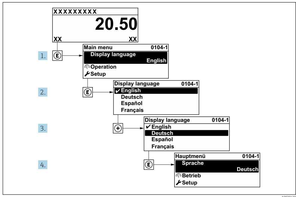
19 Exemple d'afficheur local
