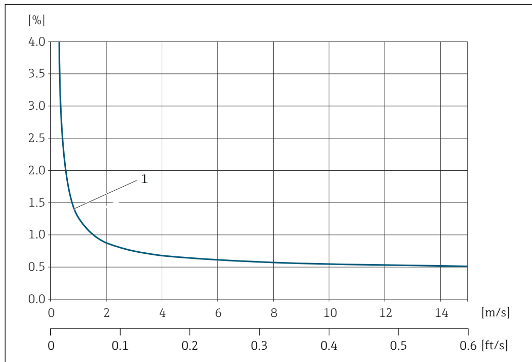
26 Exemple d'écart de mesure max. (débit volumique) en % de m.
