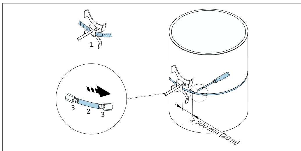
21 Support avec colliers de serrage (grands diamètres nominaux)
