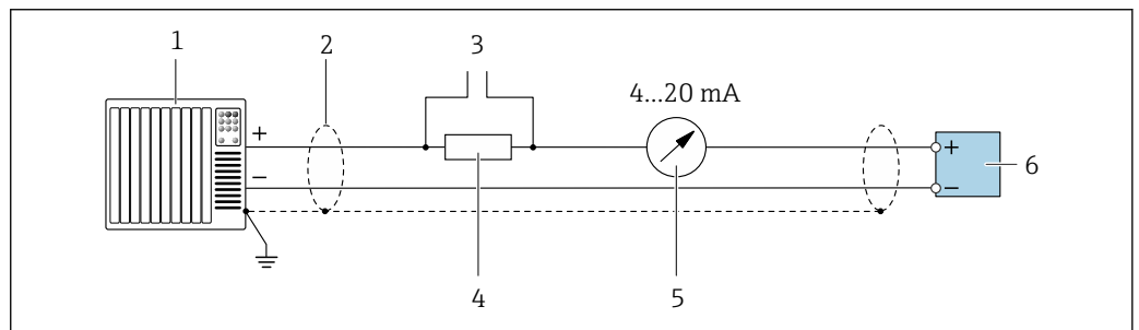
39 Exemple de raccordement de la sortie courant 4...20 mA HART (active)
