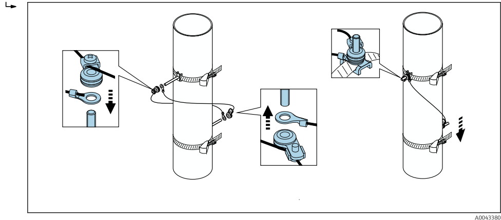
27 Positionnement des colliers de serrage (étapes 2 à 4)
