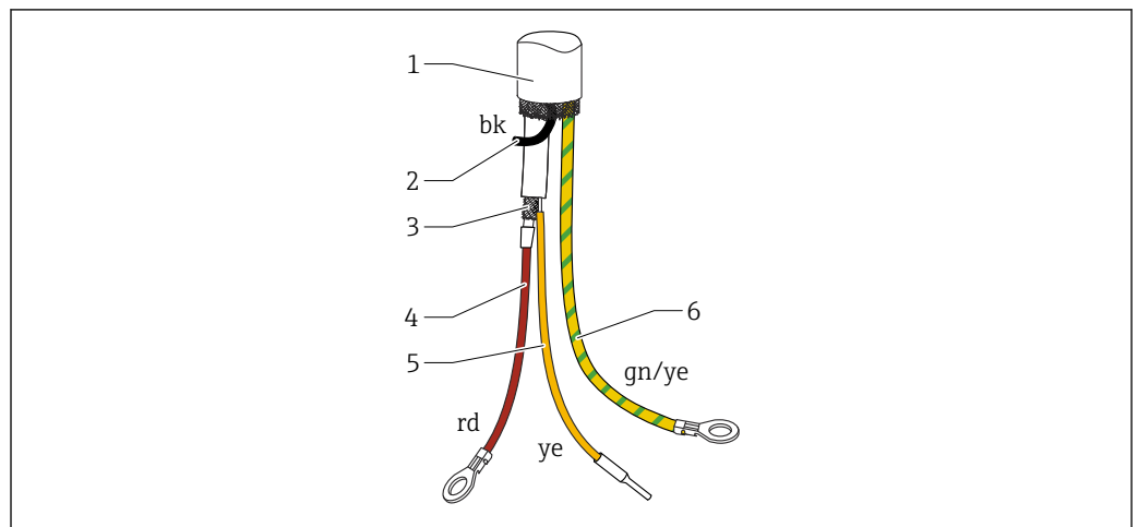
13 电缆的连接线芯
