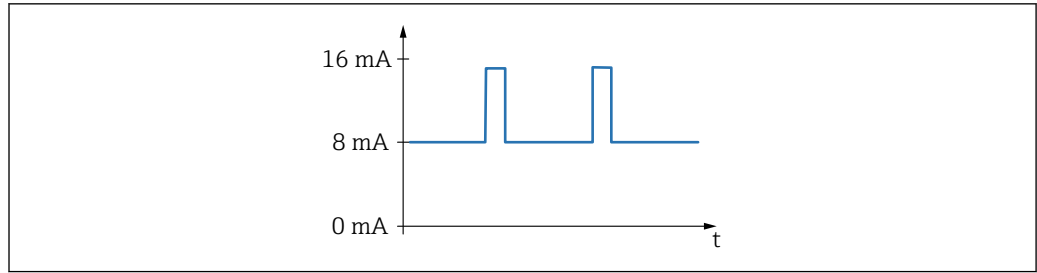
图 20 频率: 17 ... 185 Hz
