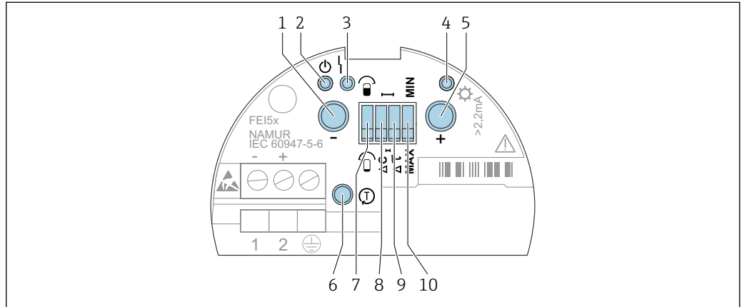
28 FEI58 的人机接口
