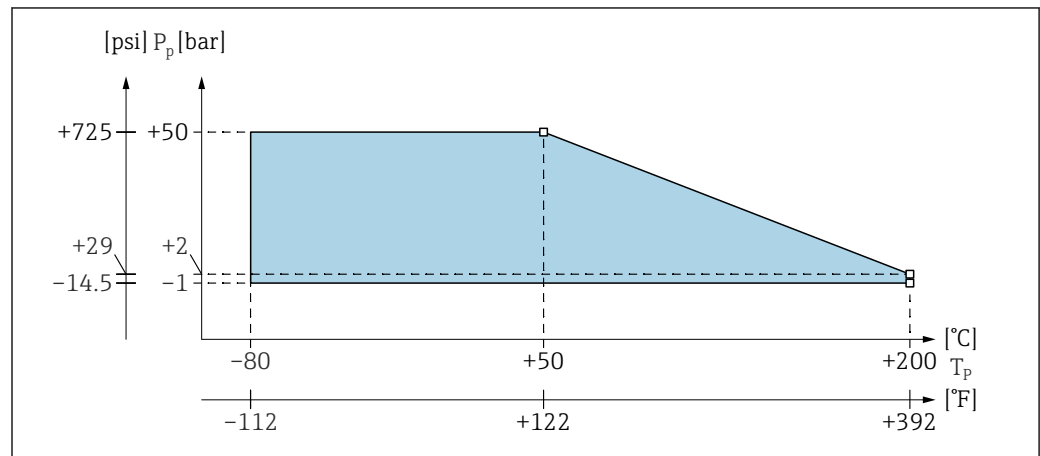
62 Diagrama de deriva de presión y temperatura para sondas de cable de longitud inactiva totalmente aislada
