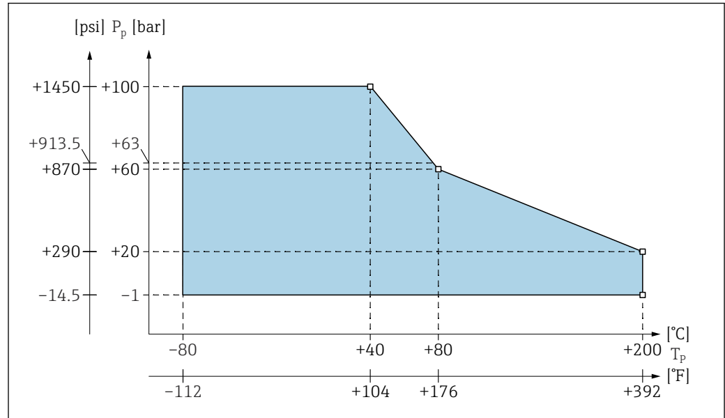
61 Diagrama de deriva de presión y temperatura para sondas de cable sin longitud inactiva o con longitud inactiva
