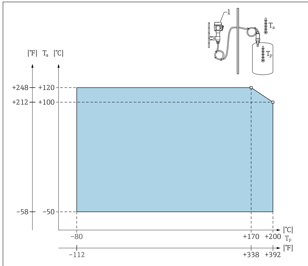
59 Diagrama del rango de presión de proceso: sonda con caja separada
