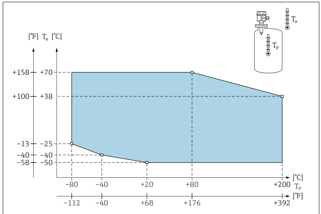
58 Diagrama del rango de presión de proceso: sonda con caja compacta
