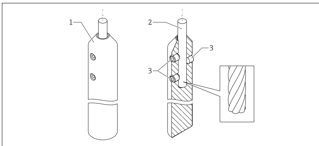
6 Visión general del contrapeso tensor
