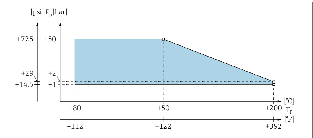
62 Diagramme de déclassement de la pression et de la température pour les sondes à câble de longueur inactive entièrement isolées
