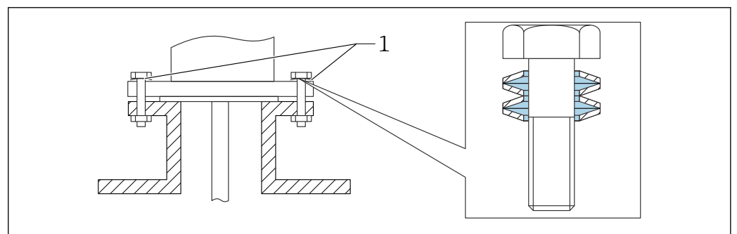
12 Montage sur rondelle élastique
