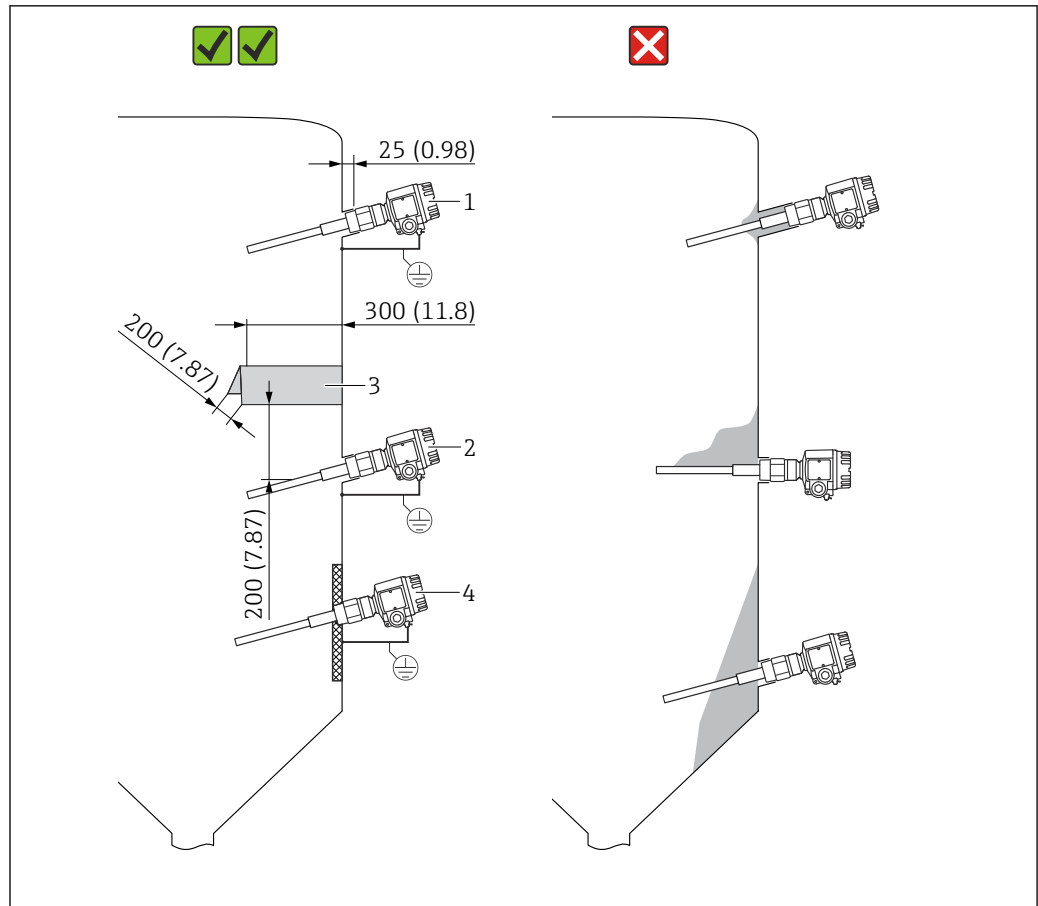
2 Montaggio laterale della sonda . Unità di misura mm (in)
