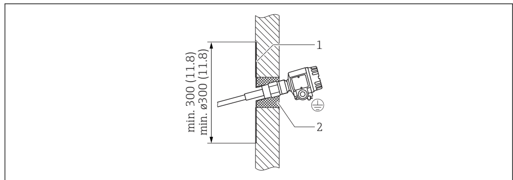
3 Sonda installata in una parete di cemento
