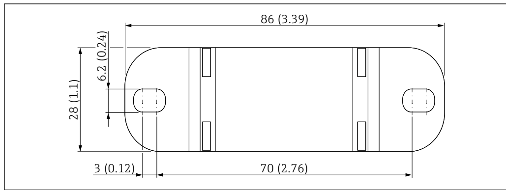
10 Descrizione della staffa da parete. Unità di misura mm (in)
