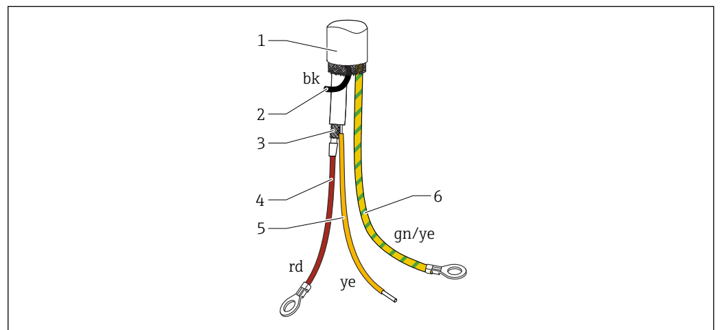
12 Connessioni del cavo
