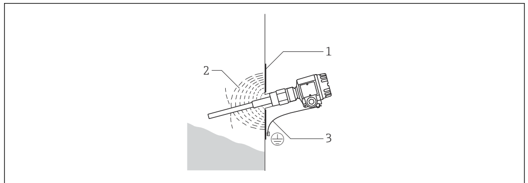
4 Sonda installata nella parete in plastica
