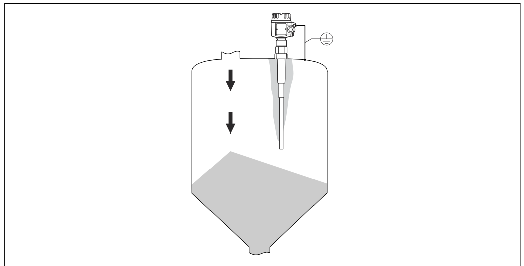
5 Depositi sull'asta della sonda
