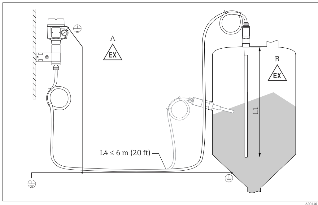
8 Connessione della sonda e della custodia separata
