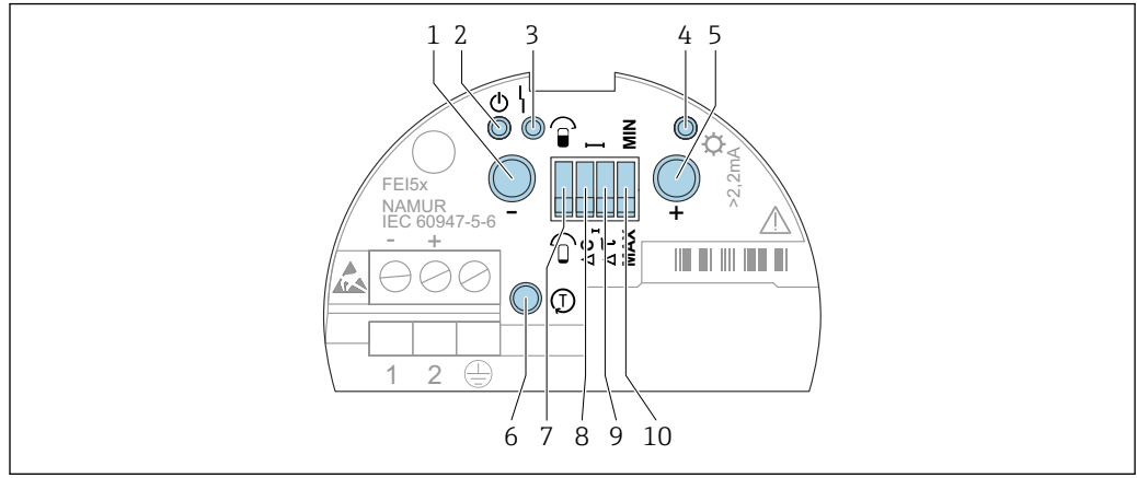
24 Interfaz de usuario de FEI58
