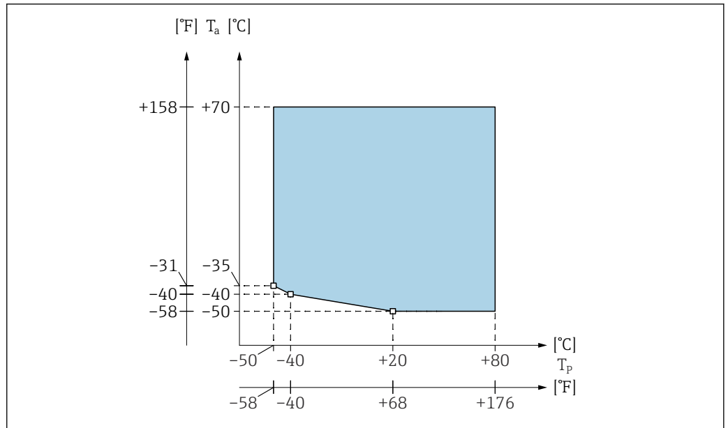
59 Sonda totalmente aislada
