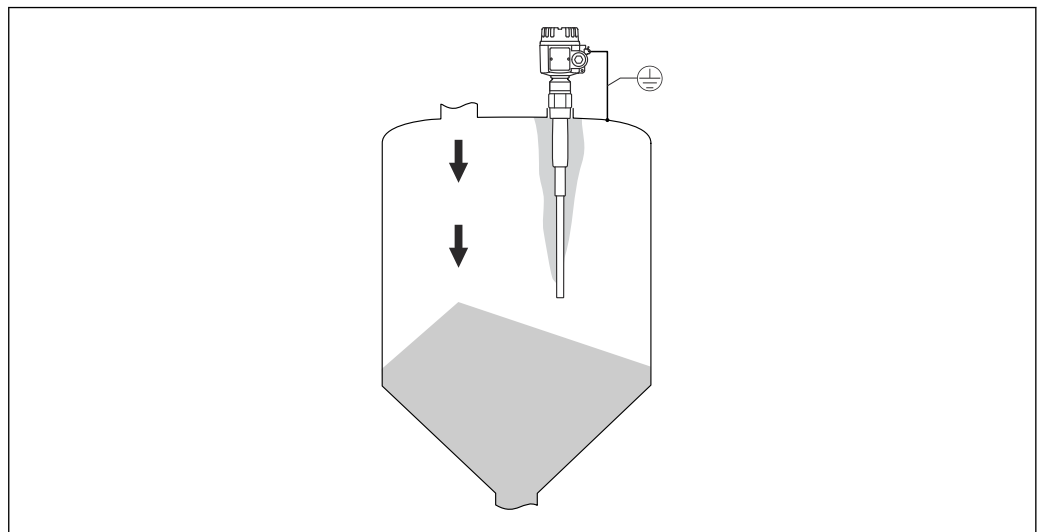
5 Ansatzbildung auf dem Sondenstab
