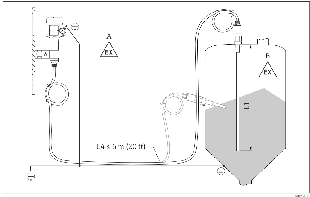
8 Anschluss der Sonde und des Separatgehäuses
