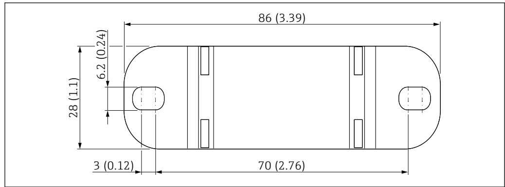
10 Wandhalterung – Übersicht. Maßeinheit mm (in)
