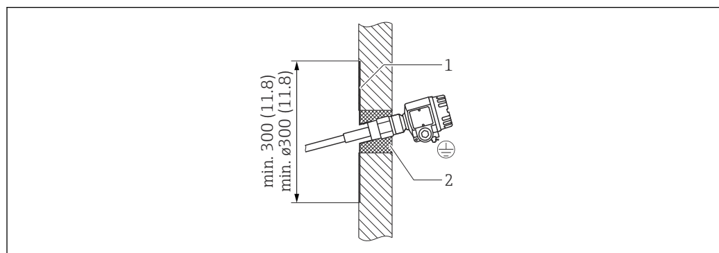
3 In einer Betonwand installierte Sonde
