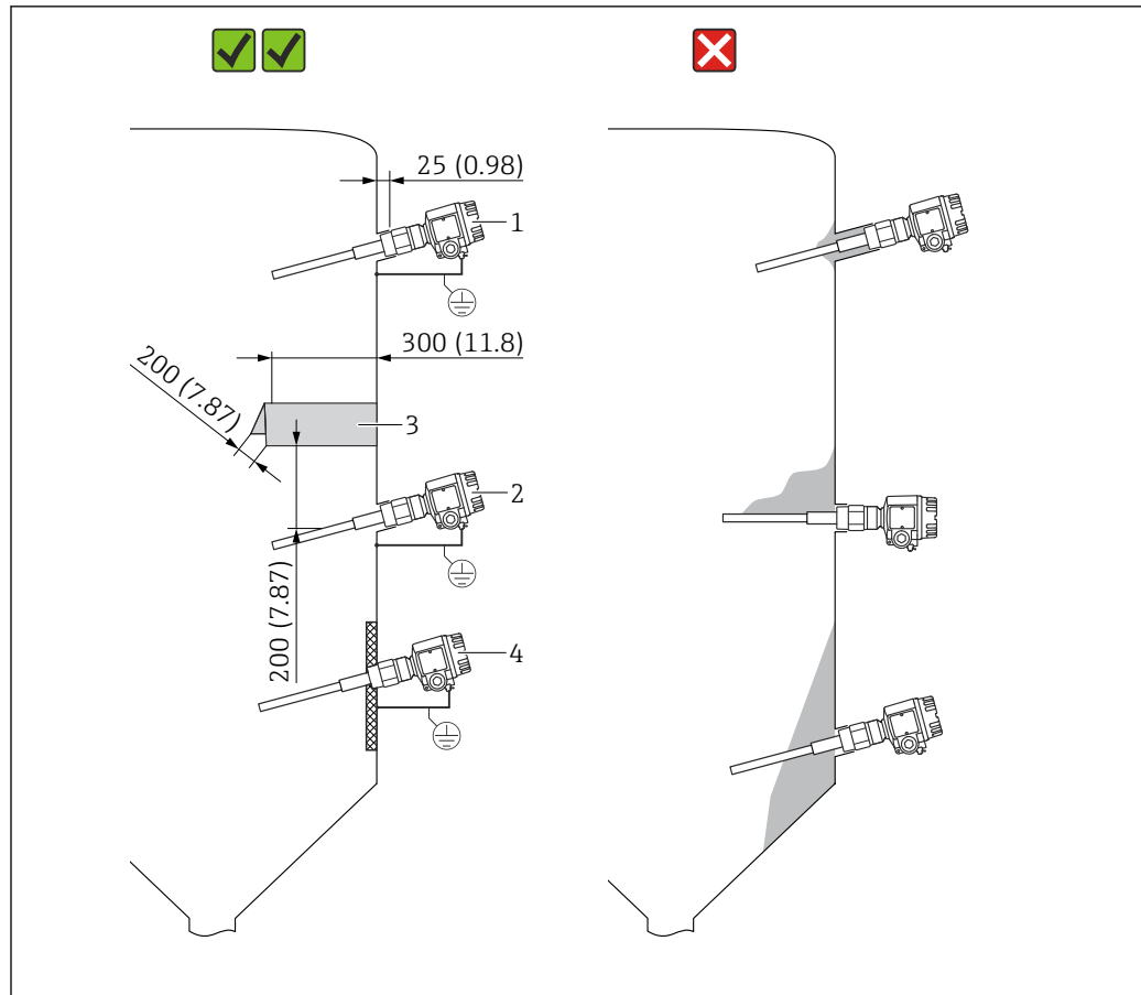
2 Montage der Sonde von der Seite . Maßeinheit mm (in)
