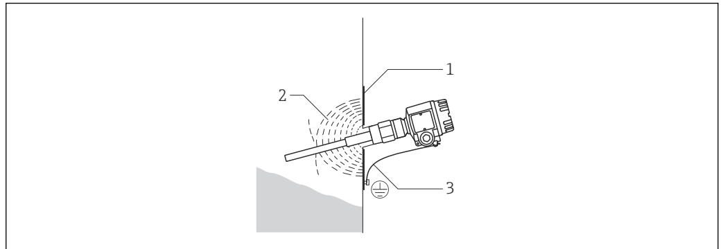
4 In einer Kunststoffwand installierte Sonde
