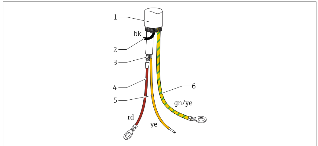
15 Кабельные соединения
