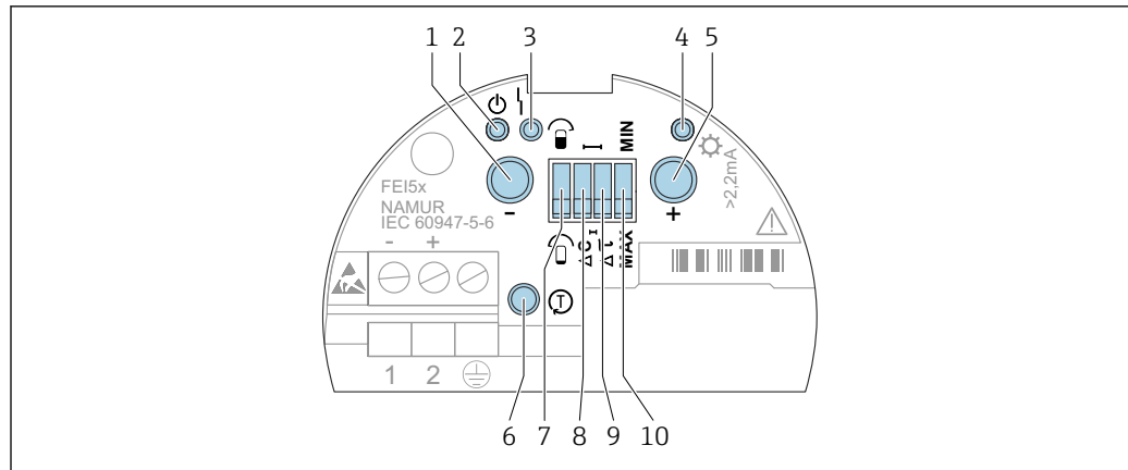
45 Интерфейс пользователя для электронной вставки FEI58
