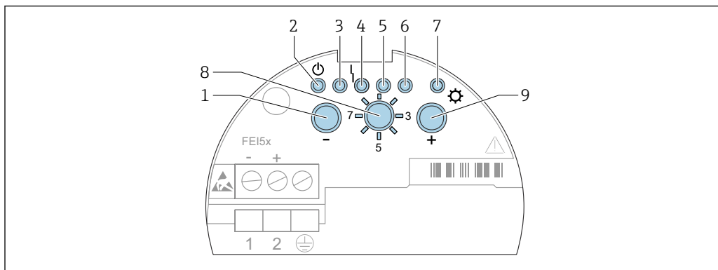
21 Интерфейс пользователя для электронных вставок FEI51, FEI52, FEI54, FEI55
