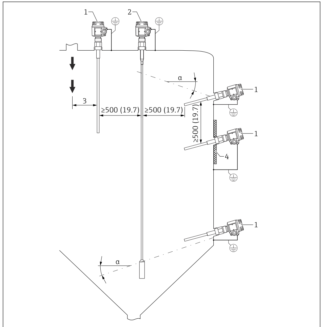
1 Примеры монтажа. Единица измерения мм (дюйм)
