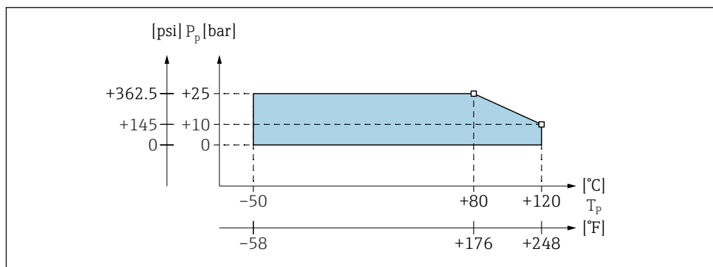
64 Диаграмма отклонения рабочего давления и температуры от номинальных значений: полностью изолированный зонд
