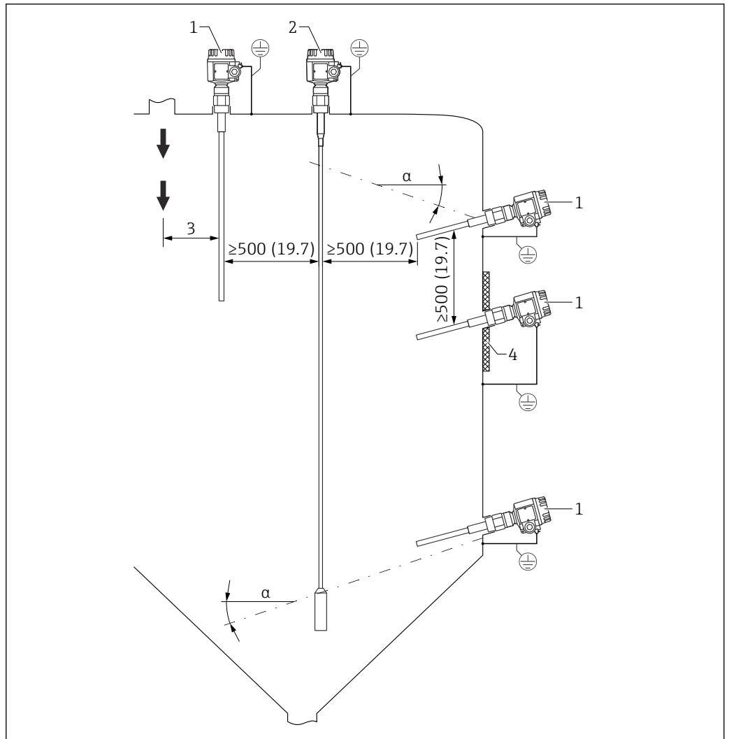
図 1 取付例。測定単位 mm (in)
