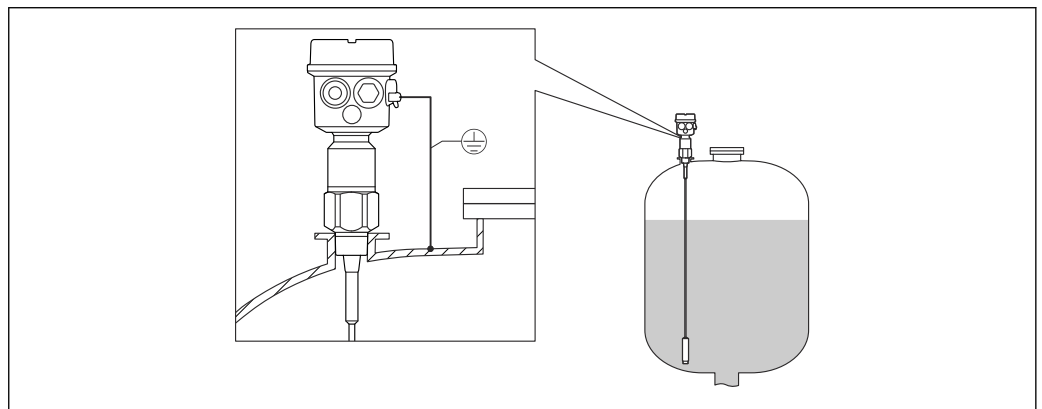
图 11 探头安装在导电材质的罐体中
