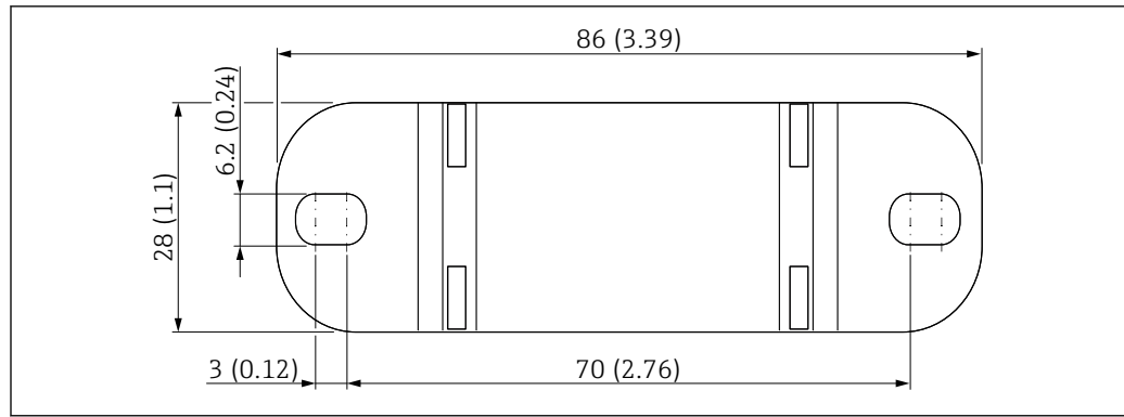
15 Visão geral do suporte de parede. Unidade de medida mm (in)
