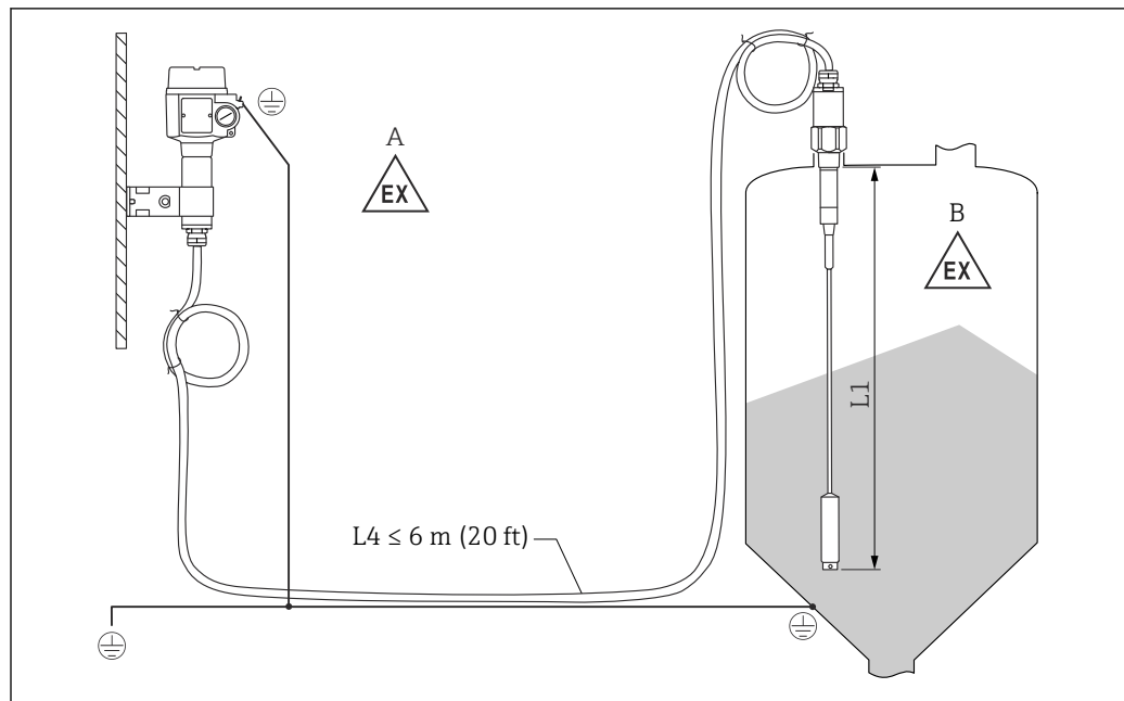
15 Anschluss der Sonde und des Separatgehäuses
