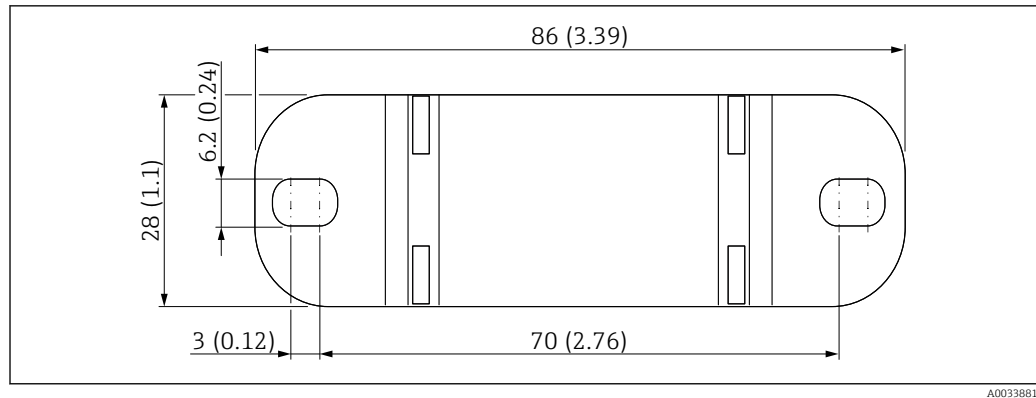
17 Wandhalterung – Übersicht. Maßeinheit mm (in)
