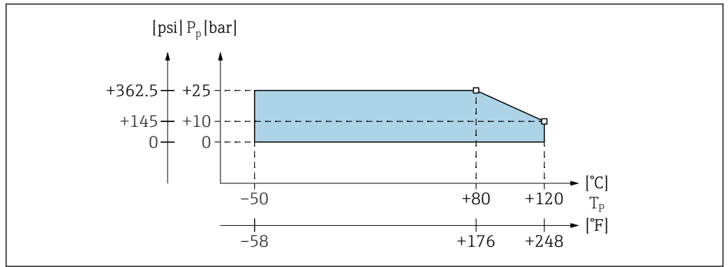
図 21 プロセス圧力と温度ディレーティングの図：完全絶縁プローブ
