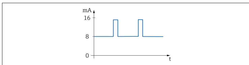
図 23 周波数 17~185 Hz の場合の PFM 信号
