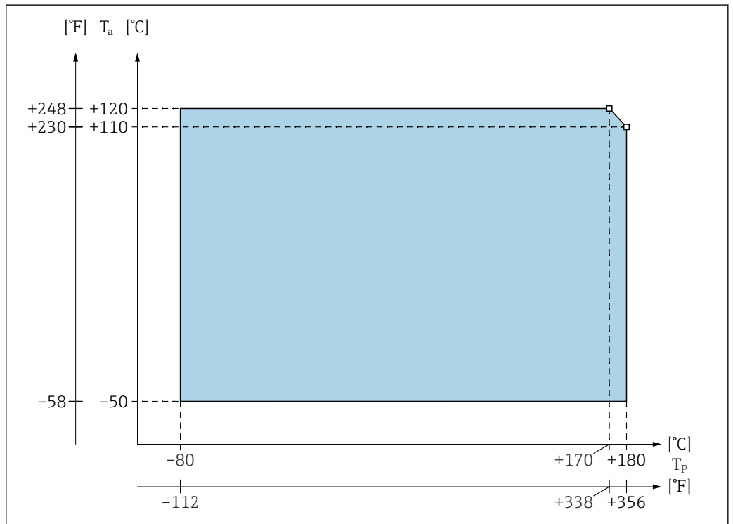
図 22 プロセス圧力範囲図
