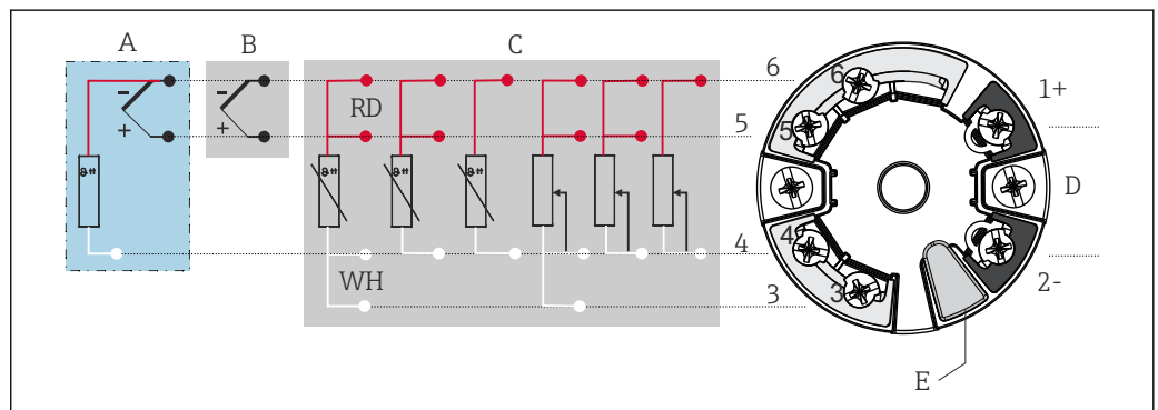
図 3 ヘッド組込型伝送器の端子割当て
