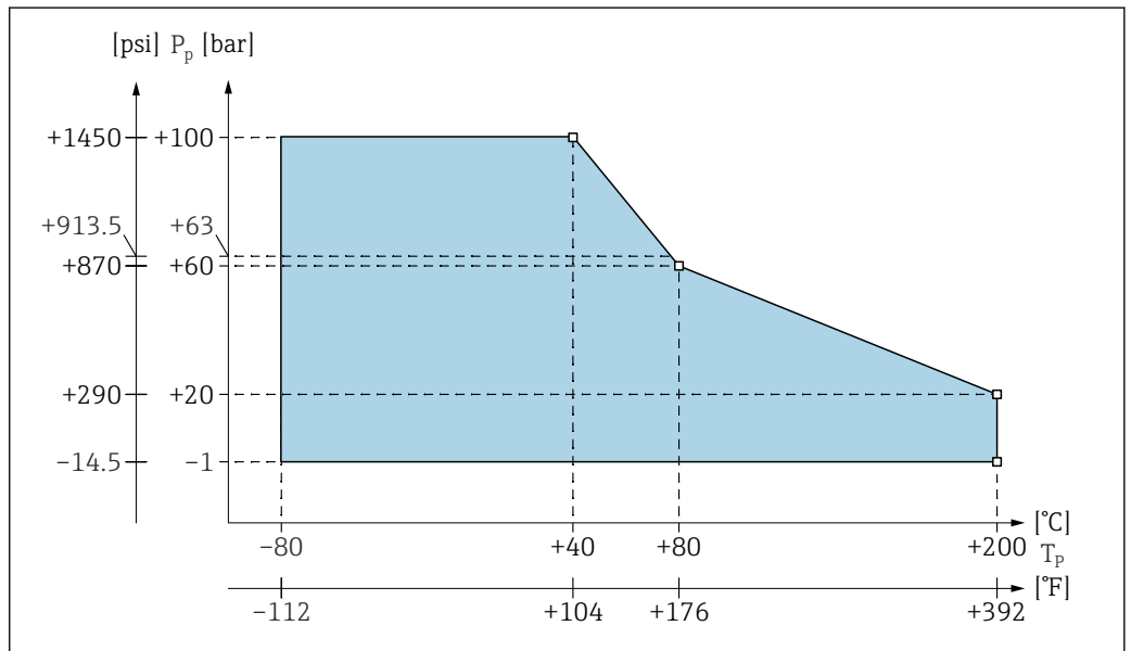
19 Grafik Prozessdruck- und Temperatur-Derating
