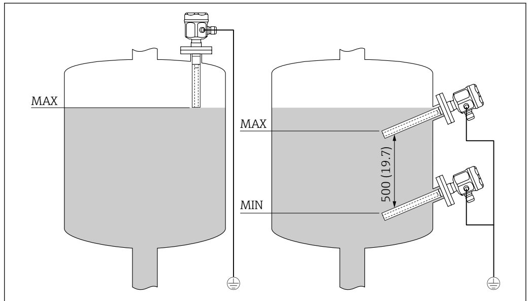
12 Einbau des Sensors in nicht leitenden Tanks. Maßeinheit mm (in)
