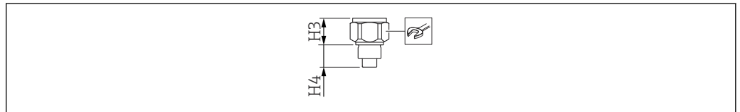
28 Hygieneanschluss mit Gewinde G \frac{3}{4} und frontbündiger Dichtung. Übersicht
