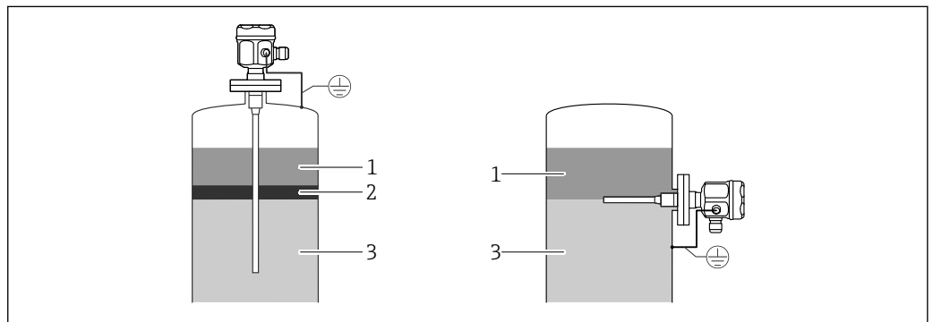
2 Trennschicht - Übersicht
