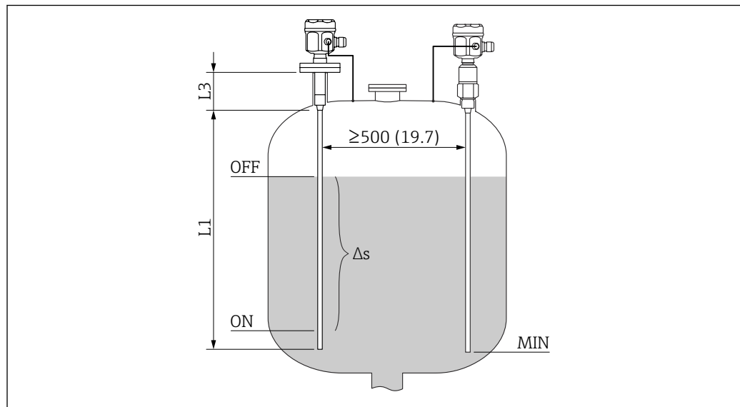
8 Messbedingungen. Maßeinheit mm (in)
