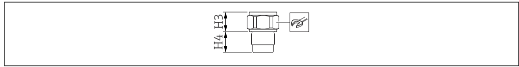
29 Hygieneanschluss mit Gewinde G1 und frontbündiger Dichtung. Übersicht
