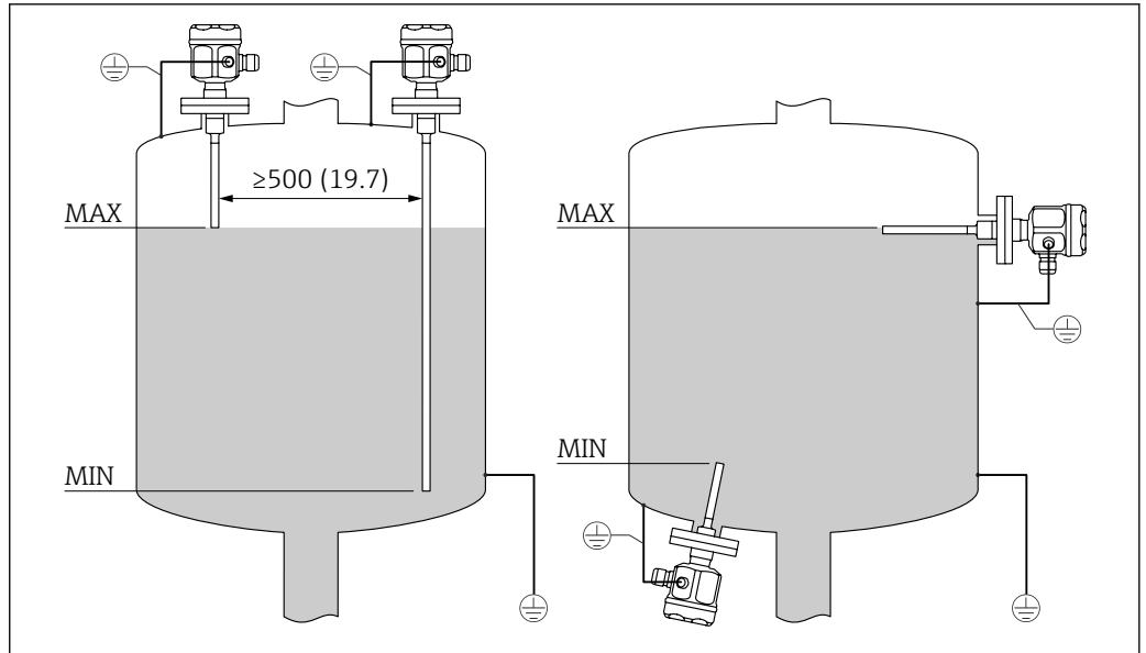
11 Einbau des Sensors in elektrisch leitenden Tanks. Maßeinheit mm (in)
