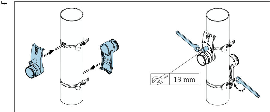
16 Anturin pidikkeiden asennus
