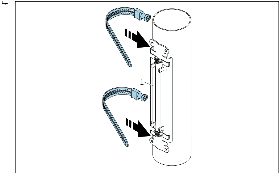
4 Anturin pidikkeen asento ja kiristyshihnojen asennus.
