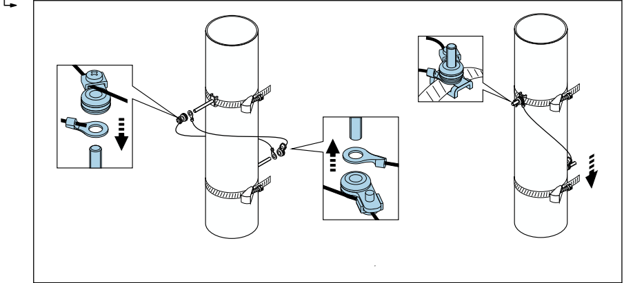
14 Kiristysihnojen sijoittaminen (vaiheet 2...4)
