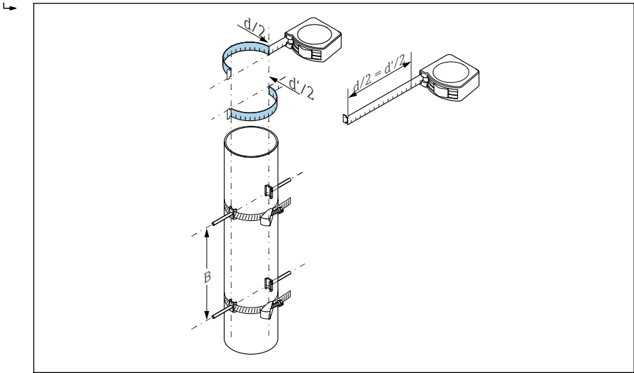
15 Kiristyshihnojen ja asennuspulttien sijoittaminen mittanauhalla (vaiheet 2 - 4)
