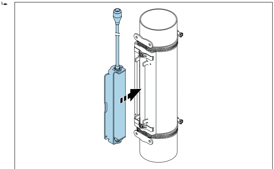
11 Placera sensorhuset
