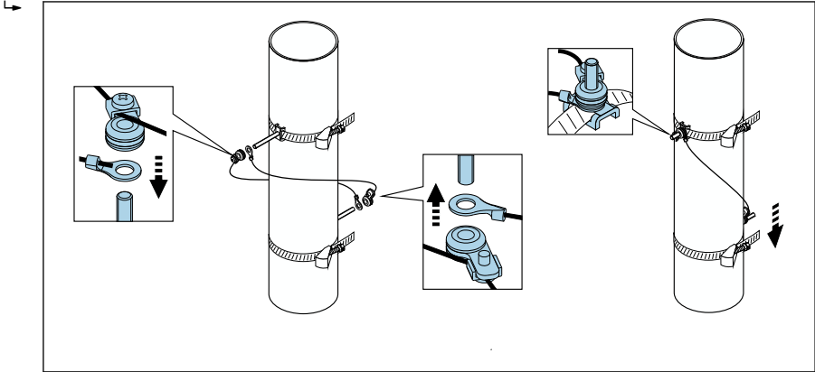
14 Placera spännbanden (arbetsmoment 2 till 4)
