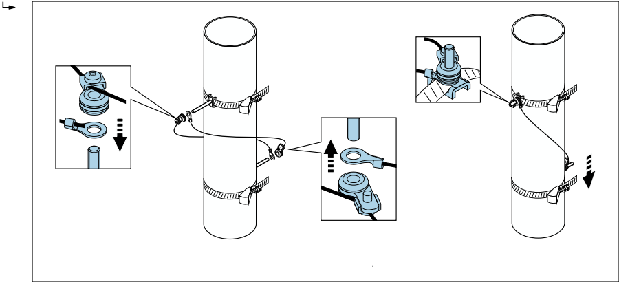
☞ 14 스트랩 밴드 배치(2~4단계)
