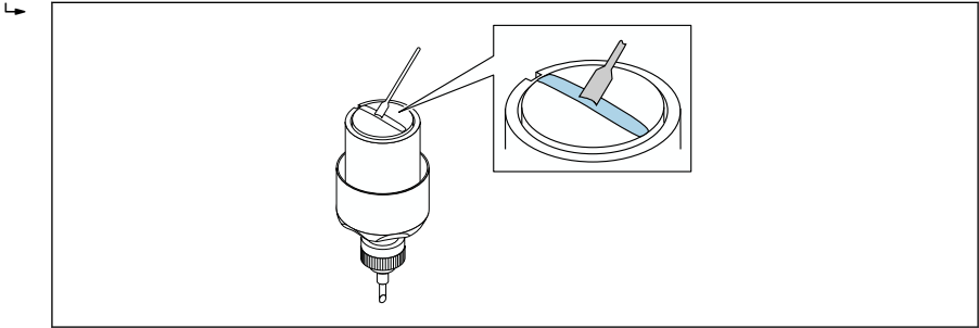
☞ 17 센서 접촉면을 커플링 젤로 코팅(커플링 패드가 없는 경우)
