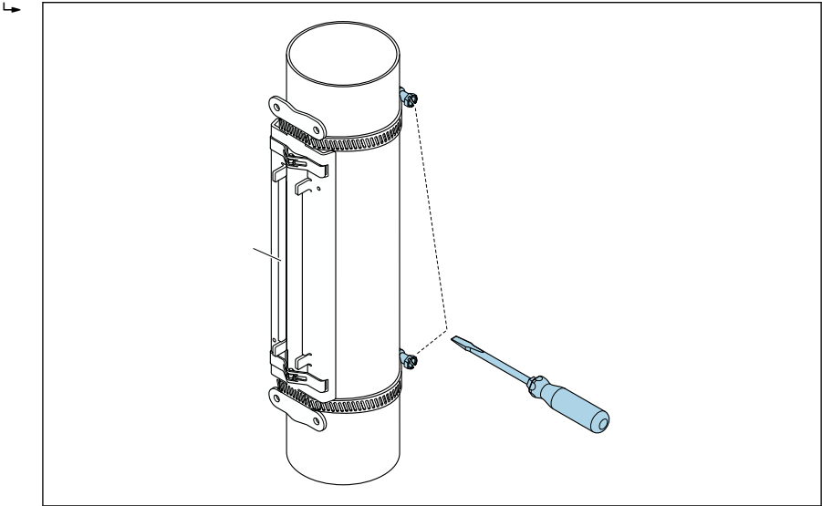
☞ 5 스트랩 밴드의 장력 조절 나사를 조이십시오.
