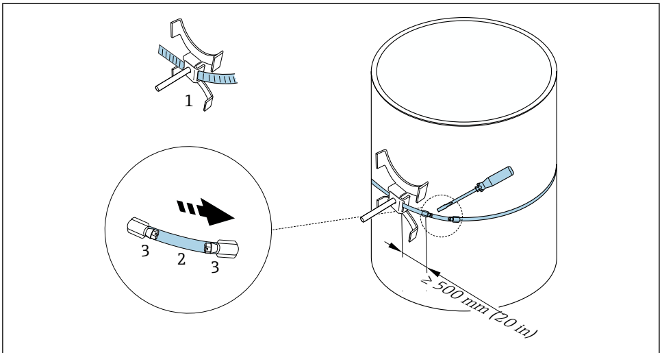
8 홀더 및 스트랩 밴드(큰 공칭 직경)
