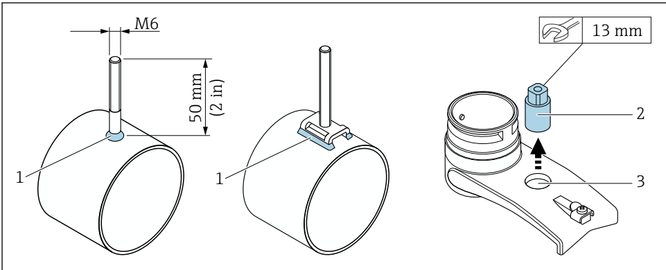
9 홀더 및 용접 볼트
