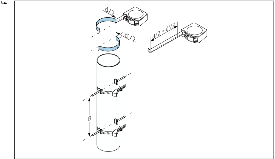
15 줄자를 사용해 스트랩 밴드 및 설치 볼트 배치(2~4단계)
