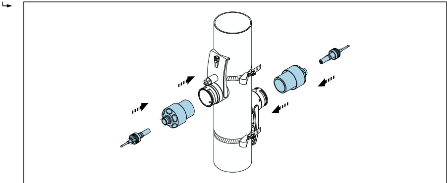
☞ 18 센서 설치 및 센서 케이블 연결
