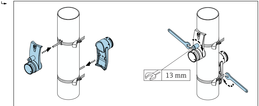
16 센서 홀더 설치
