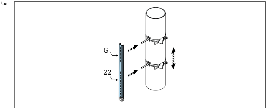
19 설치 레일에 따른 거리 결정(예: G22)
