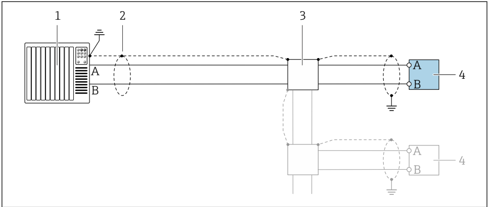
3 Csatlakozási példa: Modbus RS485, nem veszélyes terület és 2. zóna/2. alo.
