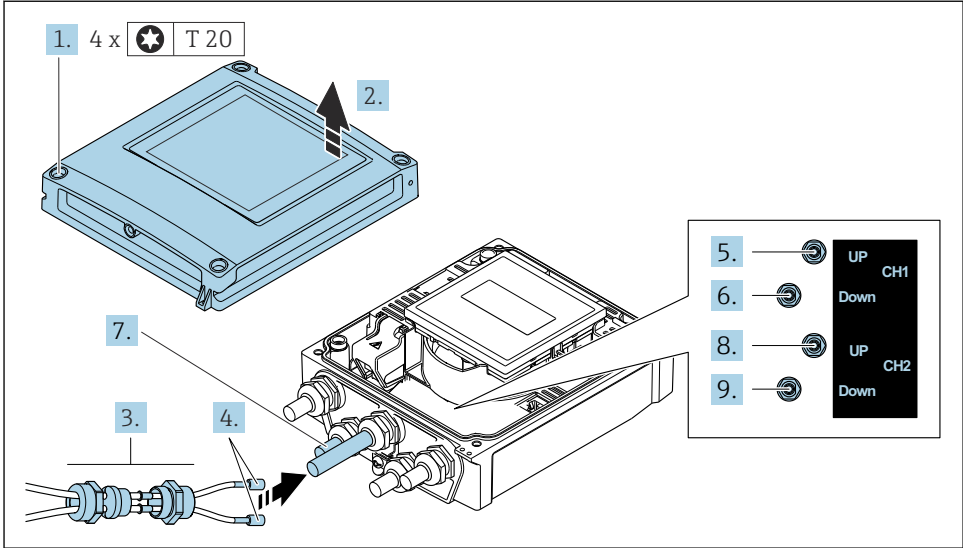
☞ 2 트랜스미터: 단자가 있는 주 전자 모듈
