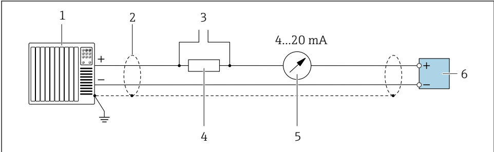
☞ 4 4~20 mA HART 전류 출력(능동)의 연결 예
