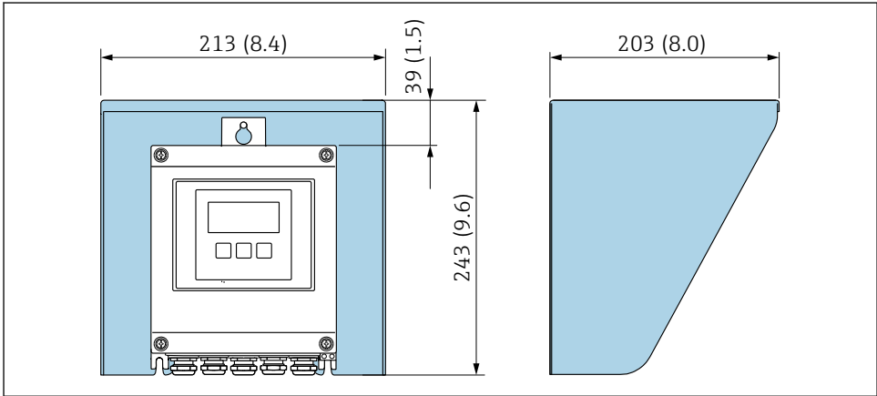
☐ 1 내후성 커버; 공학 단위: mm (in)
