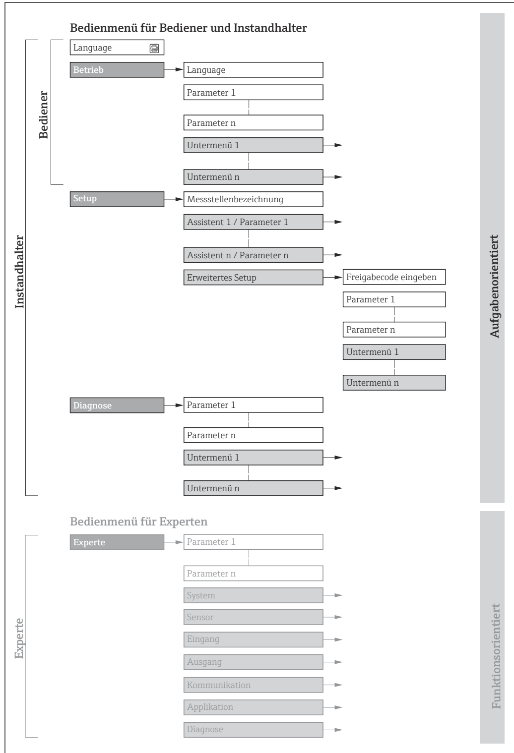
21 Schematischer Aufbau des Bedienmenüs
