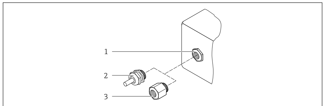
36 Mögliche Kabeleinführungen/-verschraubungen
