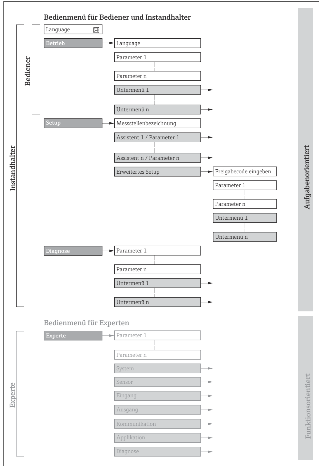
22 Schematischer Aufbau des Bedienmenüs
