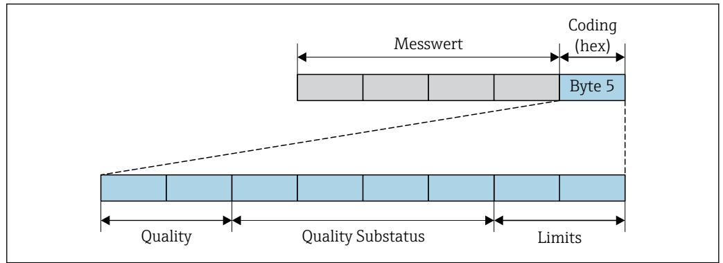
33 Struktur des Coding-Byte
