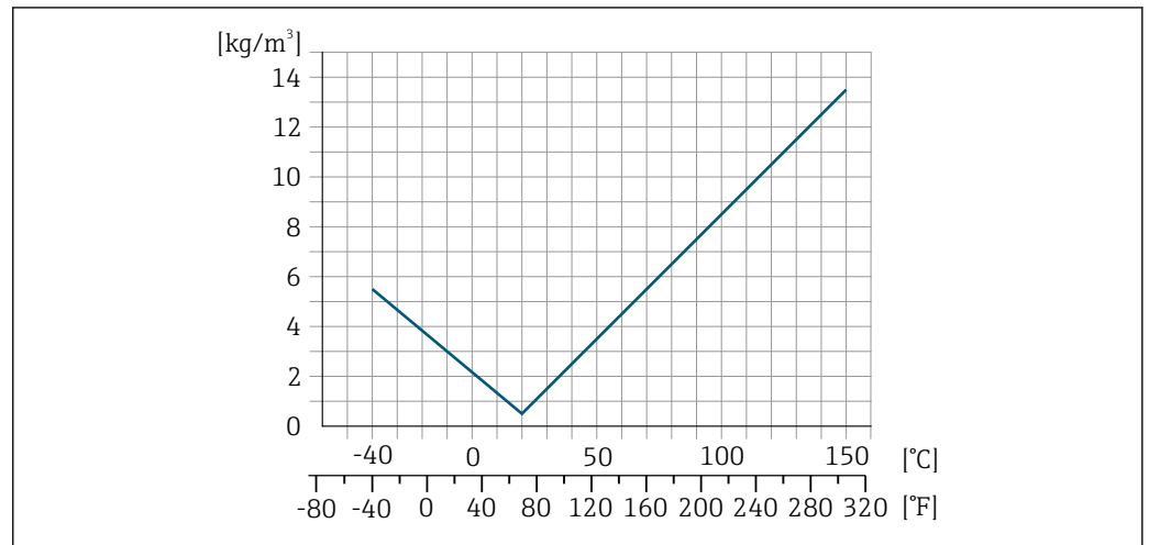
34 Felddichtejustierung, Beispiel bei +20 °C (+68 °F)
