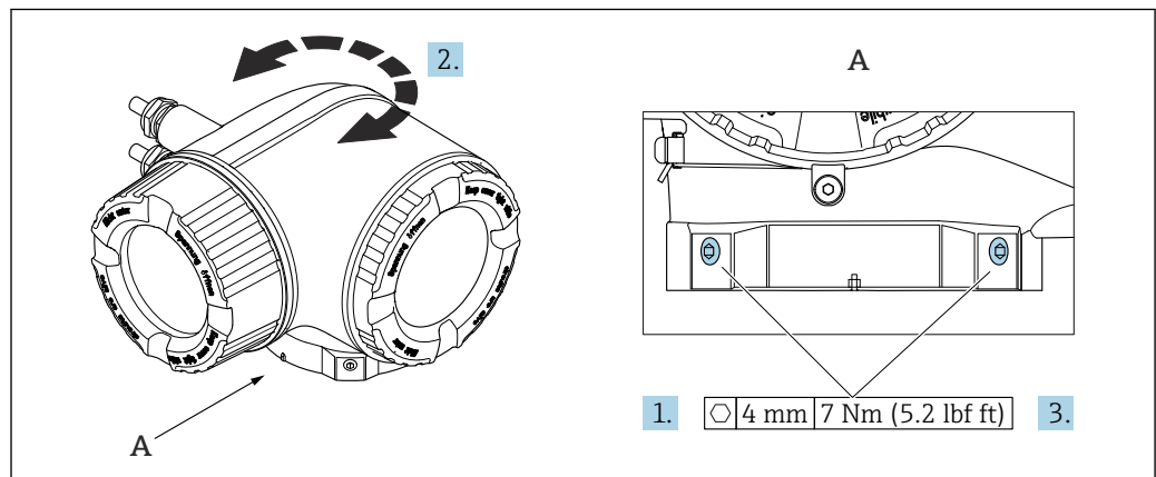
14 Ex-Gehäuse
