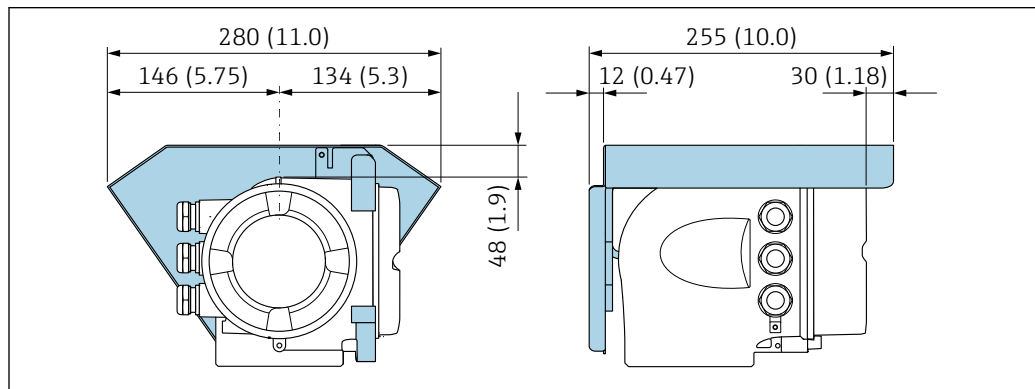
12 Wetterschutzhaube Proline 500; Maßeinheit mm (in)
