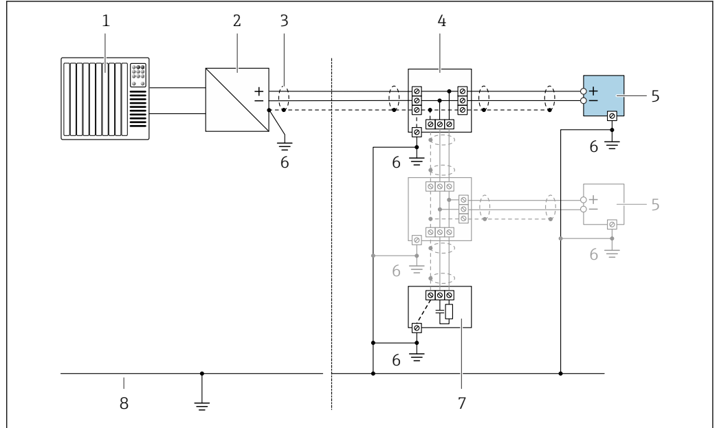
20 Anschlussbeispiel für PROFIBUS PA
