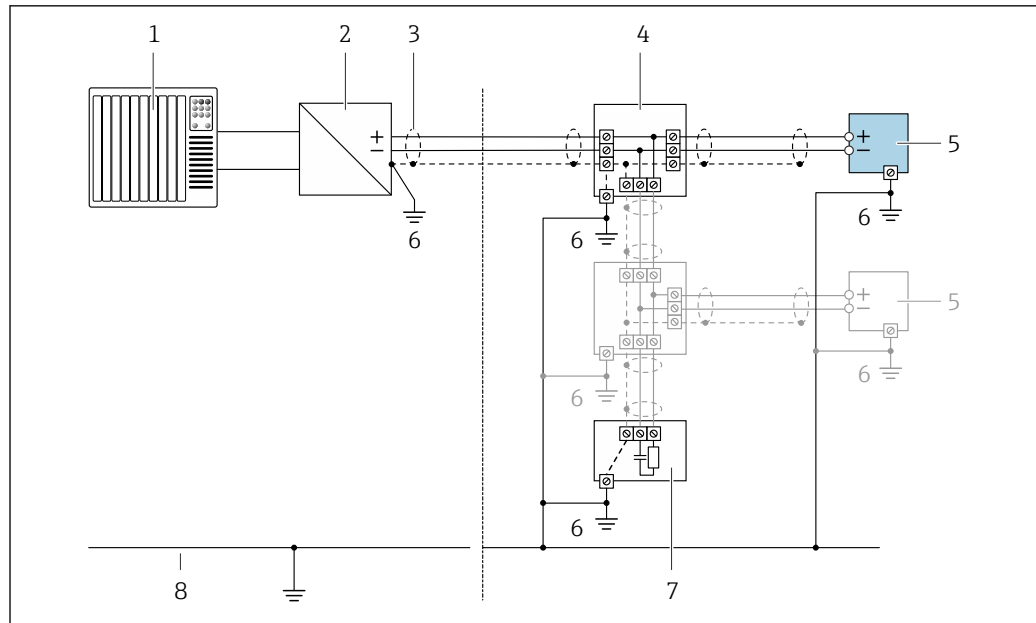
17 Anschlussbeispiel für PROFIBUS PA
