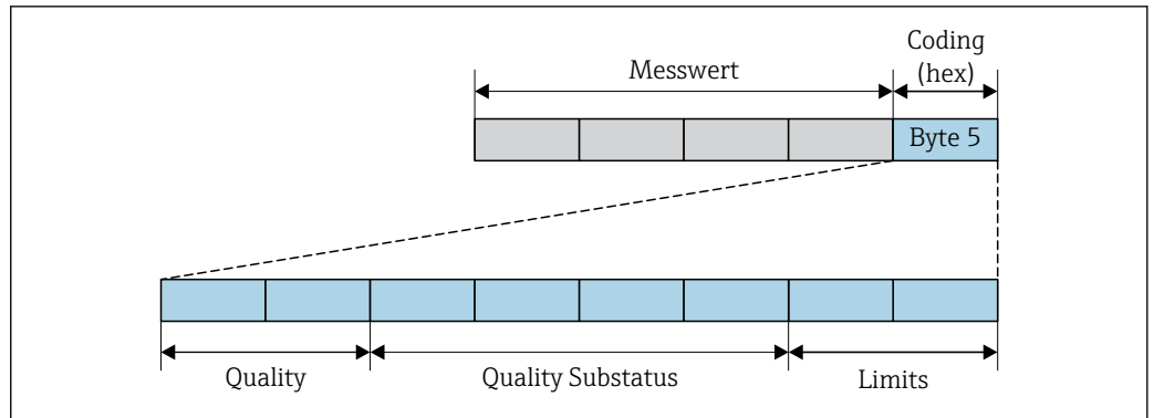
40 Struktur des Coding-Byte
