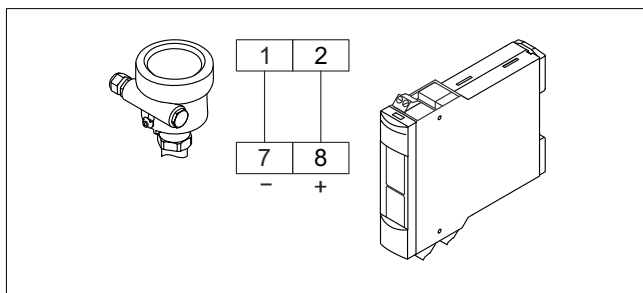
3 Připojení senzoru na jakýkoliv NAMUR senzor
