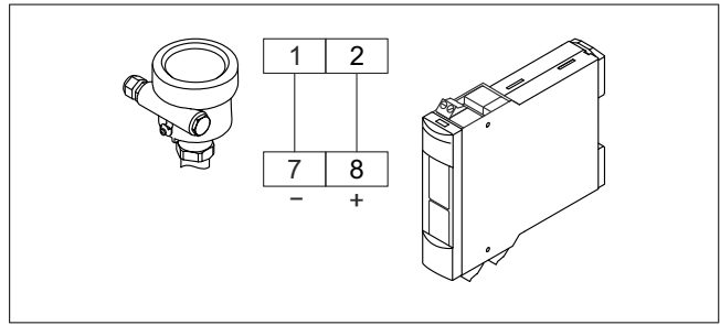
3 Подключение любого датчика NAMUR
