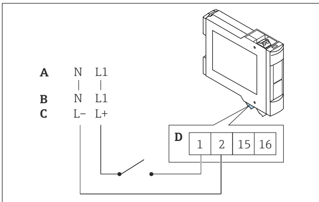
2 Расположение клемм питания
