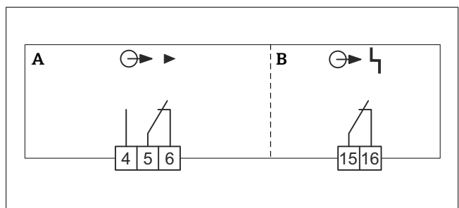
4 Подключение выходов
