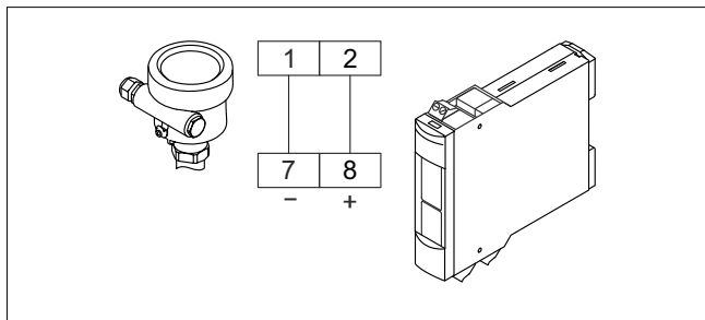
3 Anschluss mit beliebigem NAMUR-Messaufnehmer
