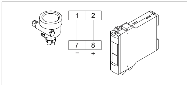
3 Priključivanje senzora na bilo koji NAMUR senzor
