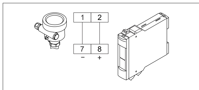
3 Koble sensoren til eventuell NAMUR-sensor
